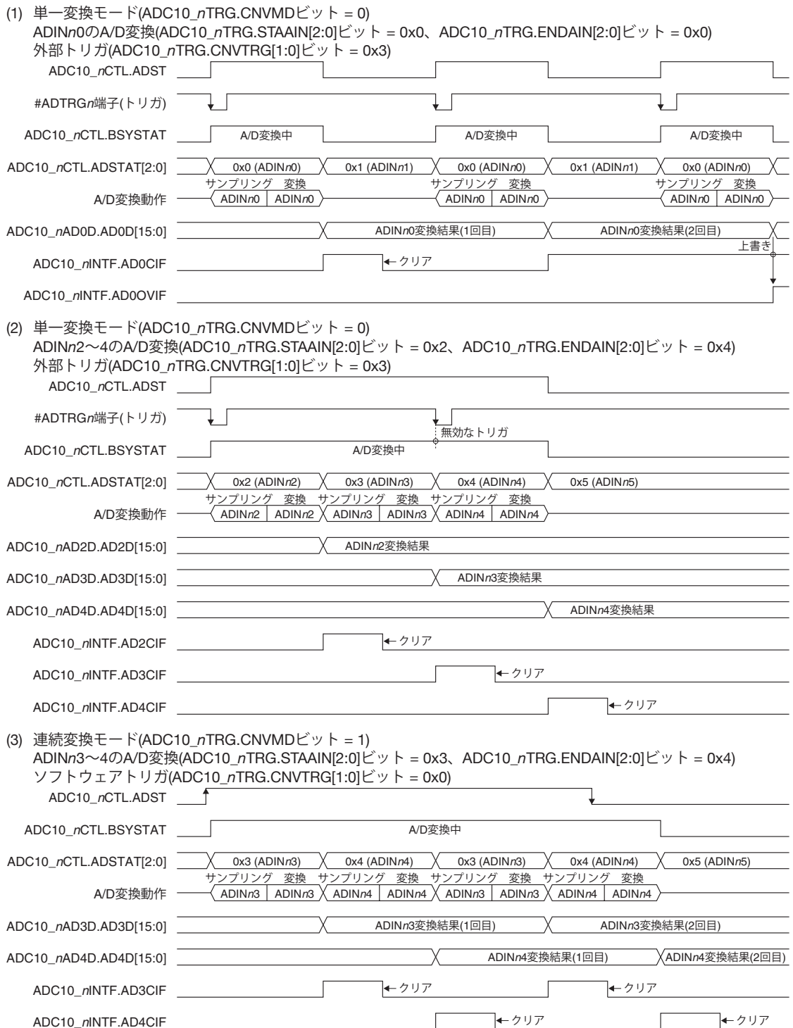
図17.4.4.1 A/D変換動作
