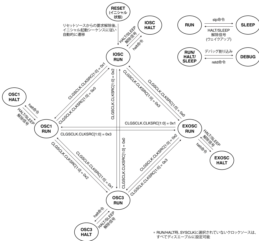
図2.4.2.1 動作モード間の状態遷移図
