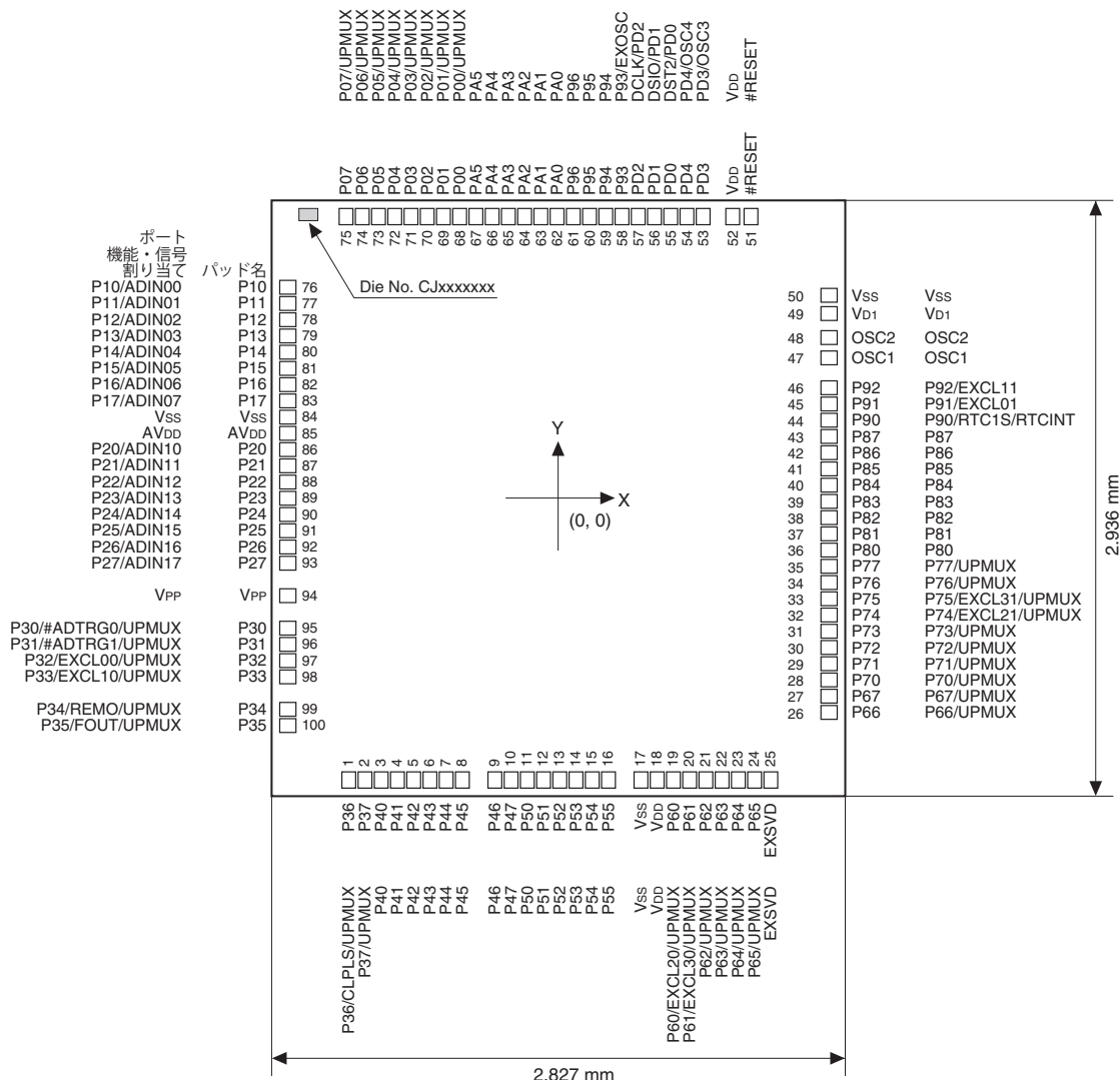
図1.3.2.1 S1C17589パッド配置図(チップ)
