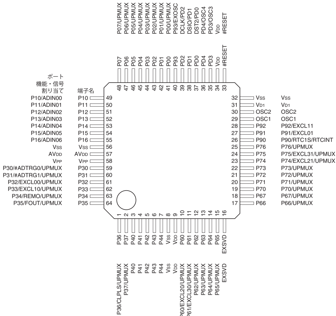
図1.3.1.3 S1C17589端子配置図 (QFP13-64PIN)
