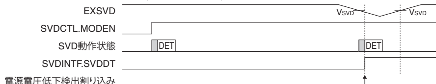
図10.4.2.1 SVD動作
