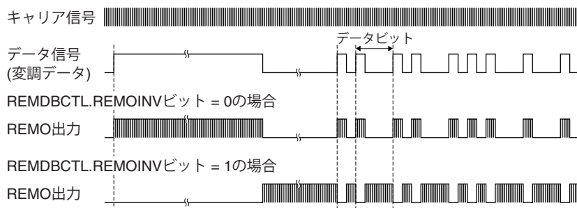
図16.4.3.1 REMO出力波形の例
