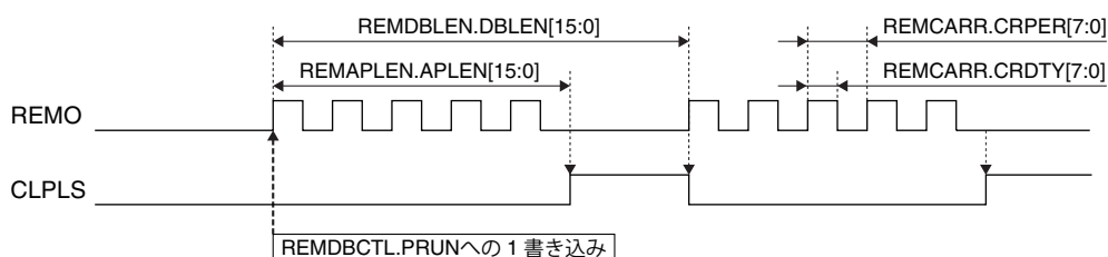
図16.6.2 駆動波形生成例
