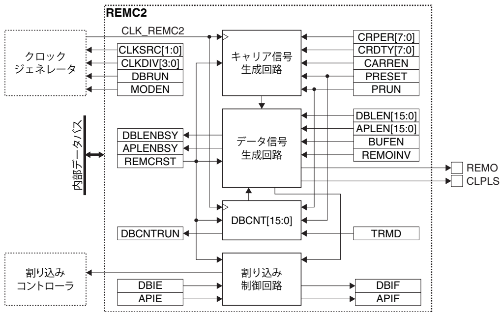
図16.1.1 REMC2の構成
