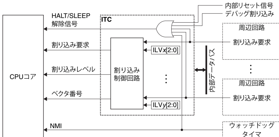
図5.1.1 ITCの構成
