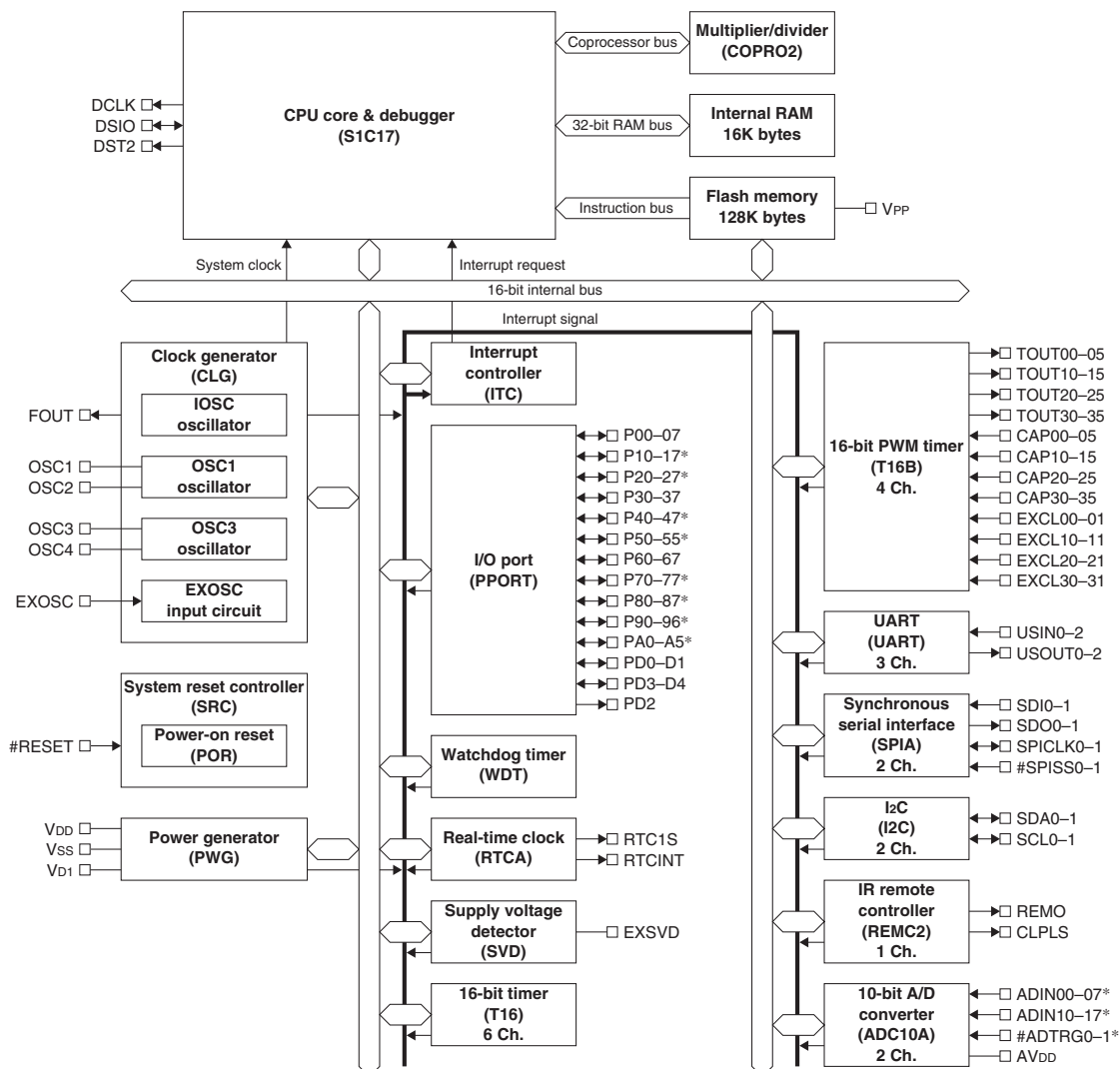
図1.2.1 S1C17589ブロック図
