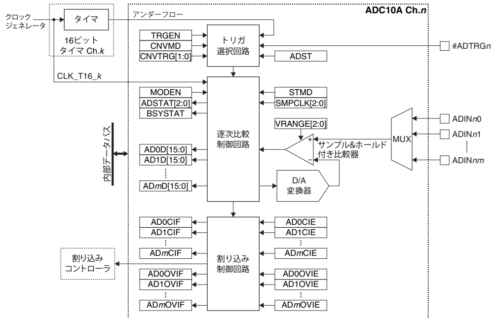
図17.1.1 ADC10Aの構成
