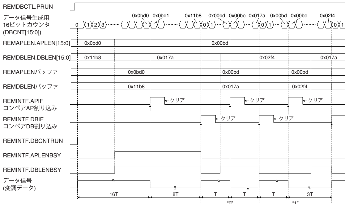
図16.4.4.1 連続送信例
