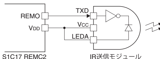
図16.2.2.1 REMC2と外部赤外線機器の接続例
