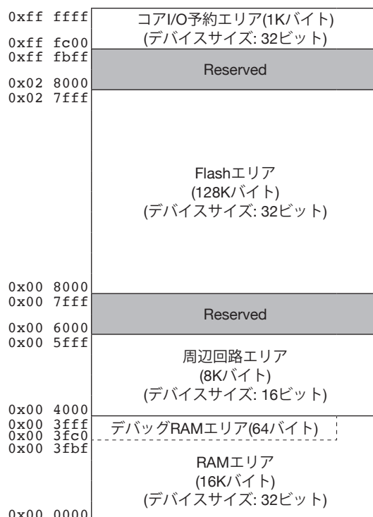
図4.1.1 メモリマップ
