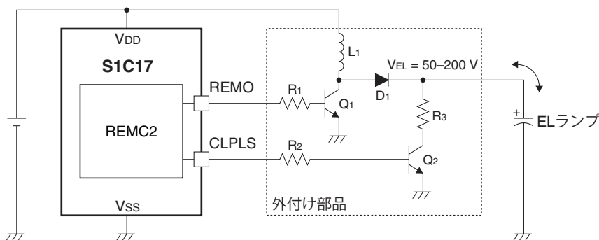
図16.6.1 ELランプ駆動回路例
