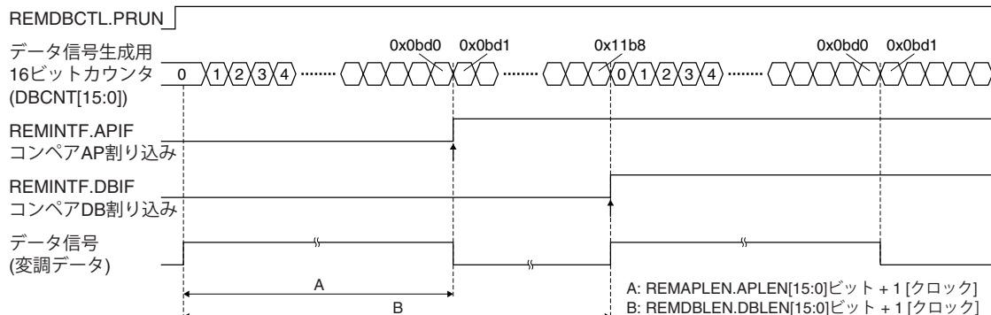
図16.4.3.3 データ信号生成例
