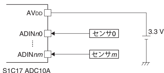
図17.2.2.1 ADC10Aと外部機器との接続
