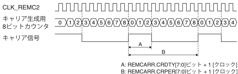
図16.4.3.2 キャリア信号生成例
