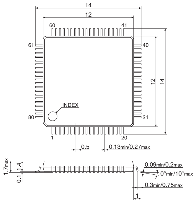
図21.2 QFP14-80PIN/パッケージ寸法
