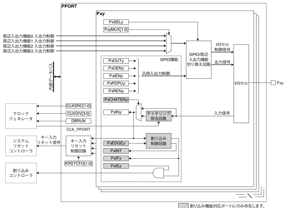
図6.1.1 PPORTの構成
