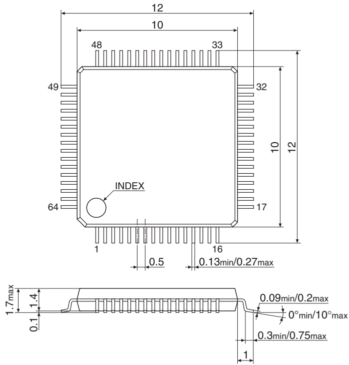
図21.3 QFP13-64PIN/パッケージ寸法
