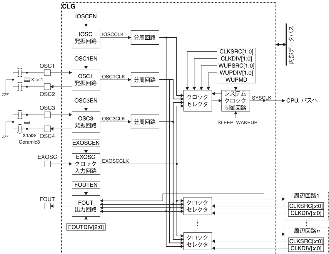
図2.3.1.1 CLGの構成
