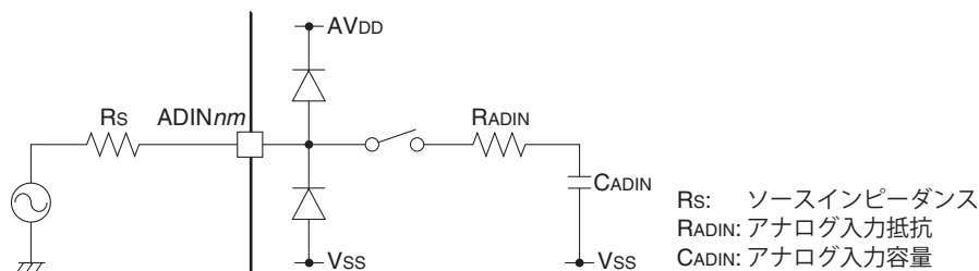
図17.3.2.1 アナログ入力等価回路
