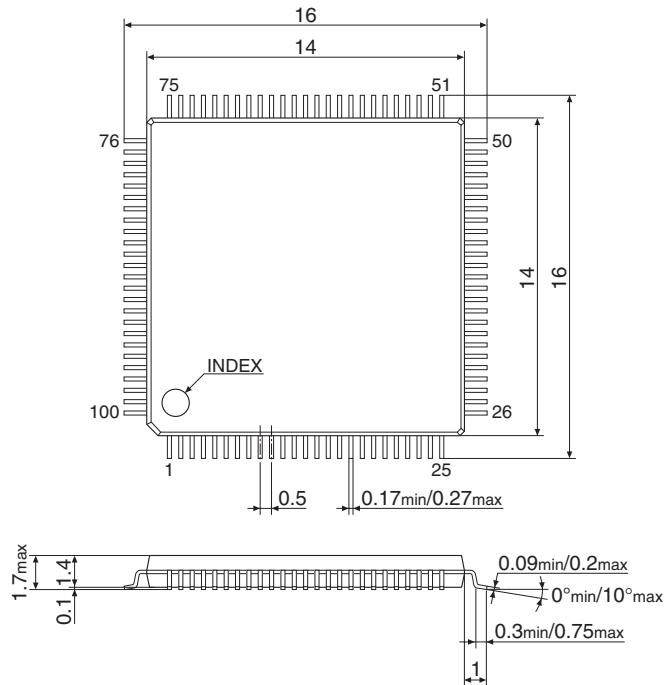
図21.1 QFP15-100PIN/パッケージ寸法
