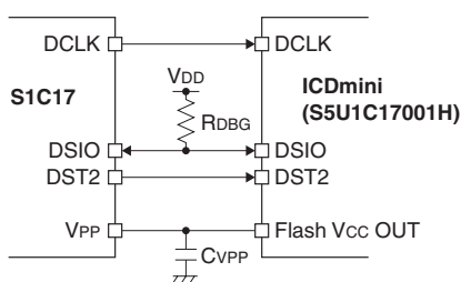
図4.3.3.1 外部接続
