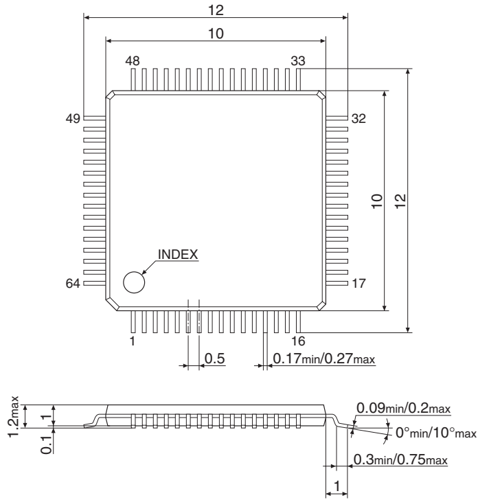
図22.2 TQFP13-64PIN/パッケージ寸法
