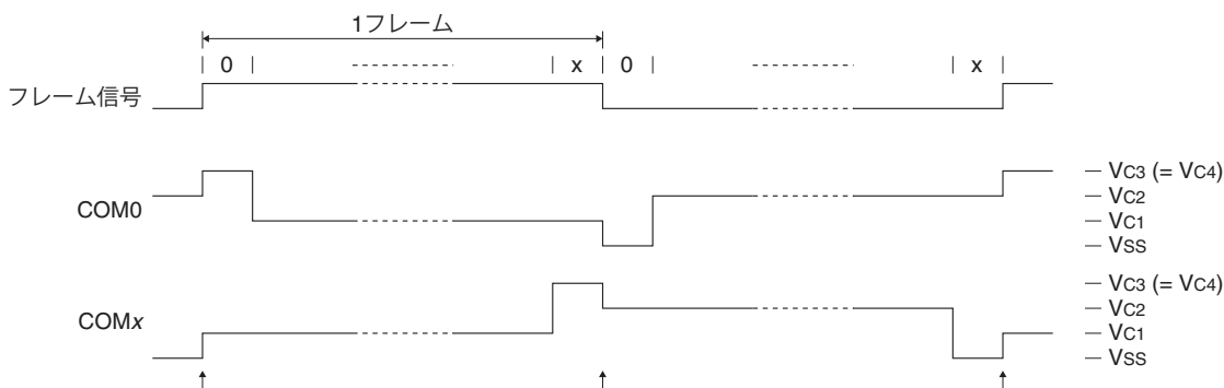
図17.7.1 フレーム割り込みタイミング(1/xデューティ、1/3バイアス)
