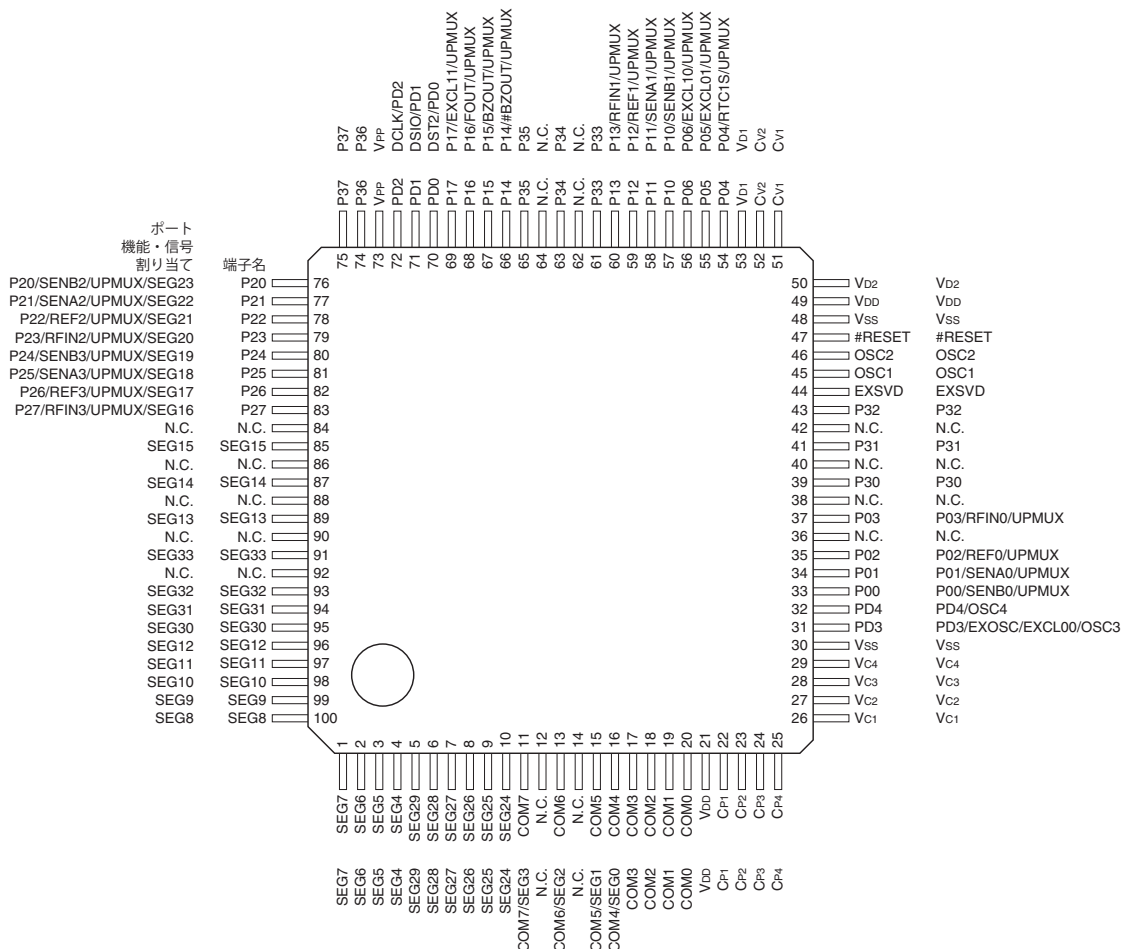
図1.3.1.4 S1C17W15端子配置図 (QFP15-100PIN)
