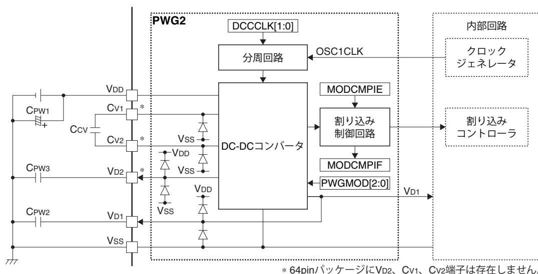
図2.1.1.1 PWG2の構成
