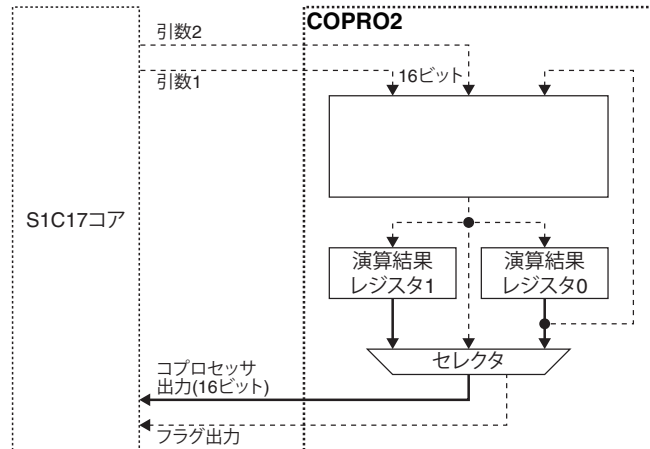
図19.6.1 演算結果読み出しモードのデータ経路
