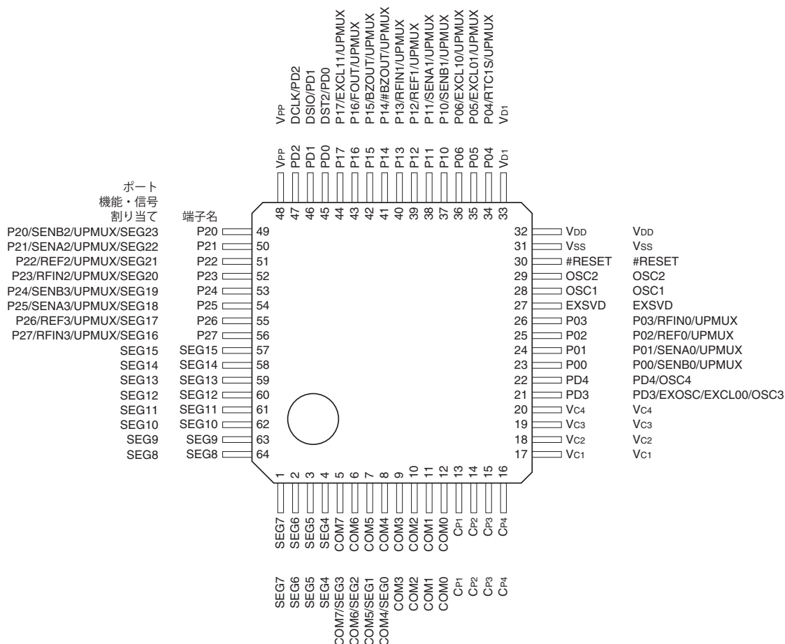
図1.3.1.2 S1C17W15端子配置図 (TQFP13-64PIN)
