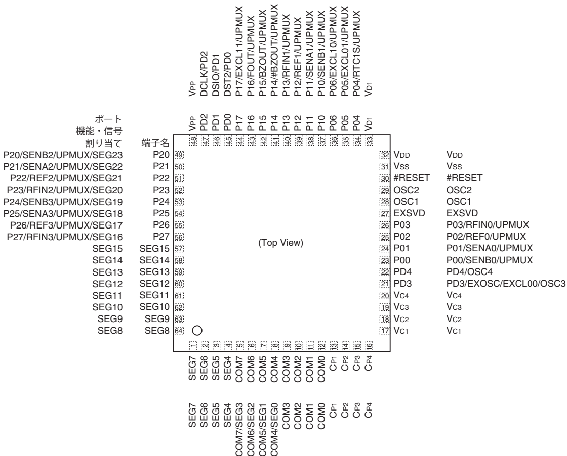
図1.3.1.1 S1C17W15端子配置図 (SQFN9-64PIN)
