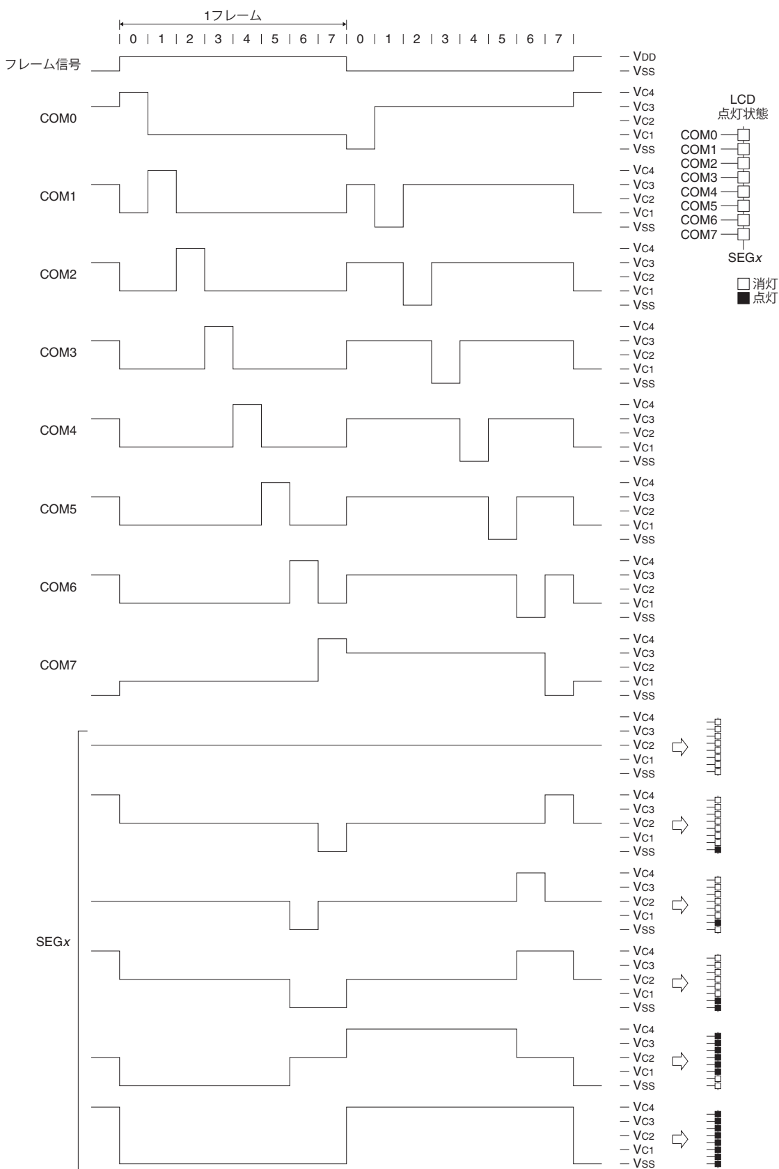
図17.5.5.1 1/8デューティの駆動波形(1/4バイアス)
