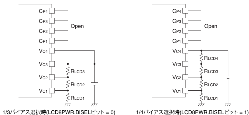
図17.4.2.1 外部印加モード1外部結線例(抵抗分割)
