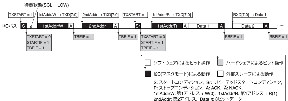
図14.4.4.2 10ビットアドレスモードのデータ送受信開始動作例(マスターモード)
