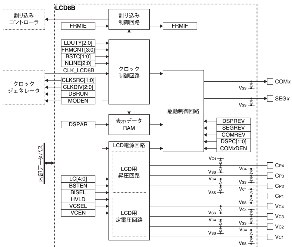
図17.1.1 LCD8Bの構成
