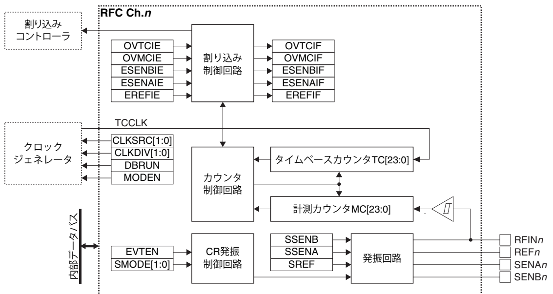
図18.1.1 RFCの構成
