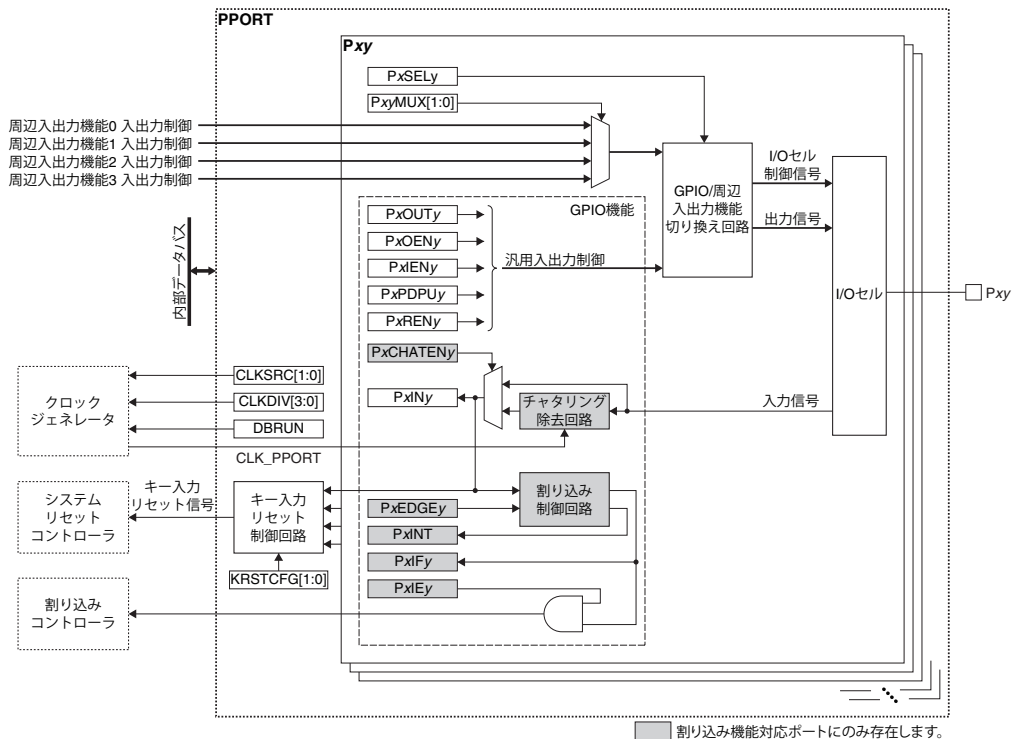
図6.1.1 PPORTの構成
