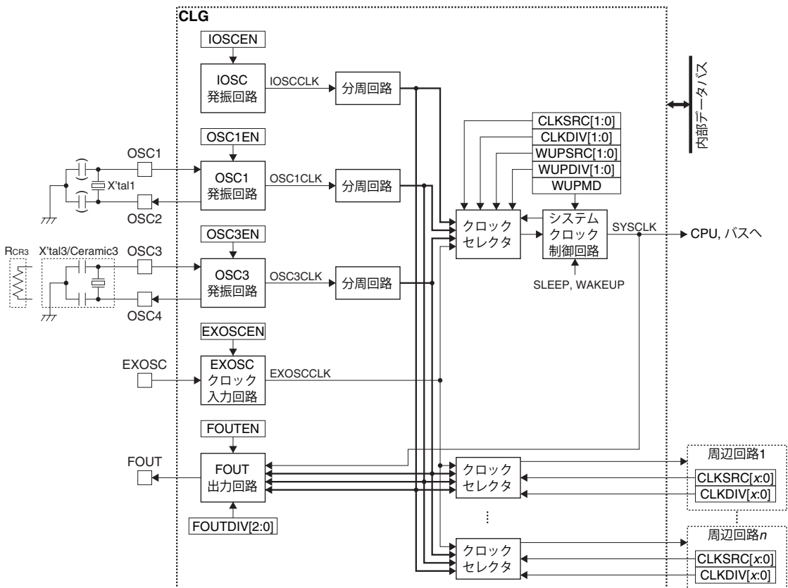
図2.3.1.1 CLGの構成
