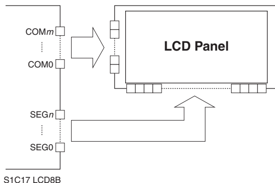
図17.2.2.1 LCD8BとLCDパネルの接続例
