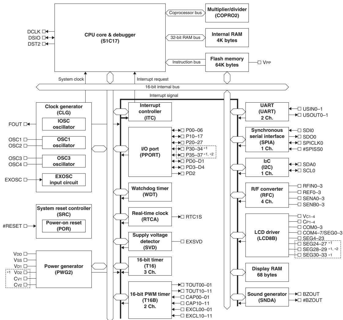
図1.2.1 S1C17W15ブロック図
