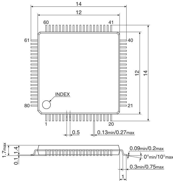
図22.3 QFP14-80PIN/パッケージ寸法
