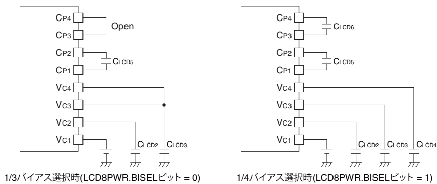
図17.4.3.1 外部印加モード2外部結線例(VC1印加時)
