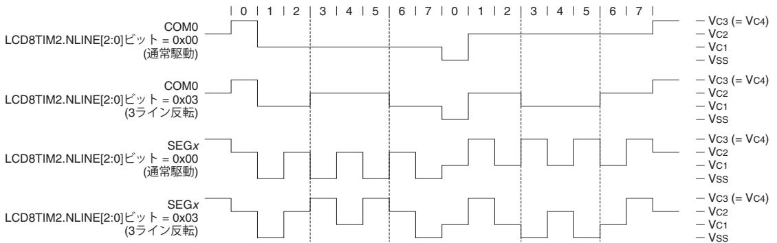
図17.5.7.1 1/8デューティ(1/3バイアス)の通常駆動時と3ライン反転時の駆動波形
