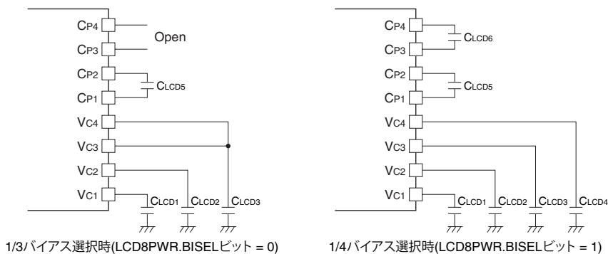
図17.4.1.1 内部生成モード外部結線例
