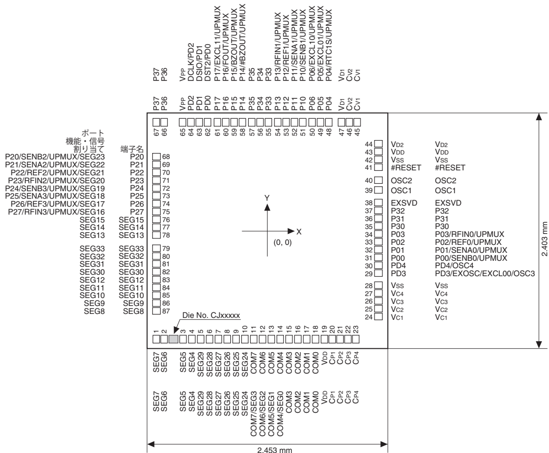
図1.3.2.1 S1C17W15/パッド配置図(チップ)
