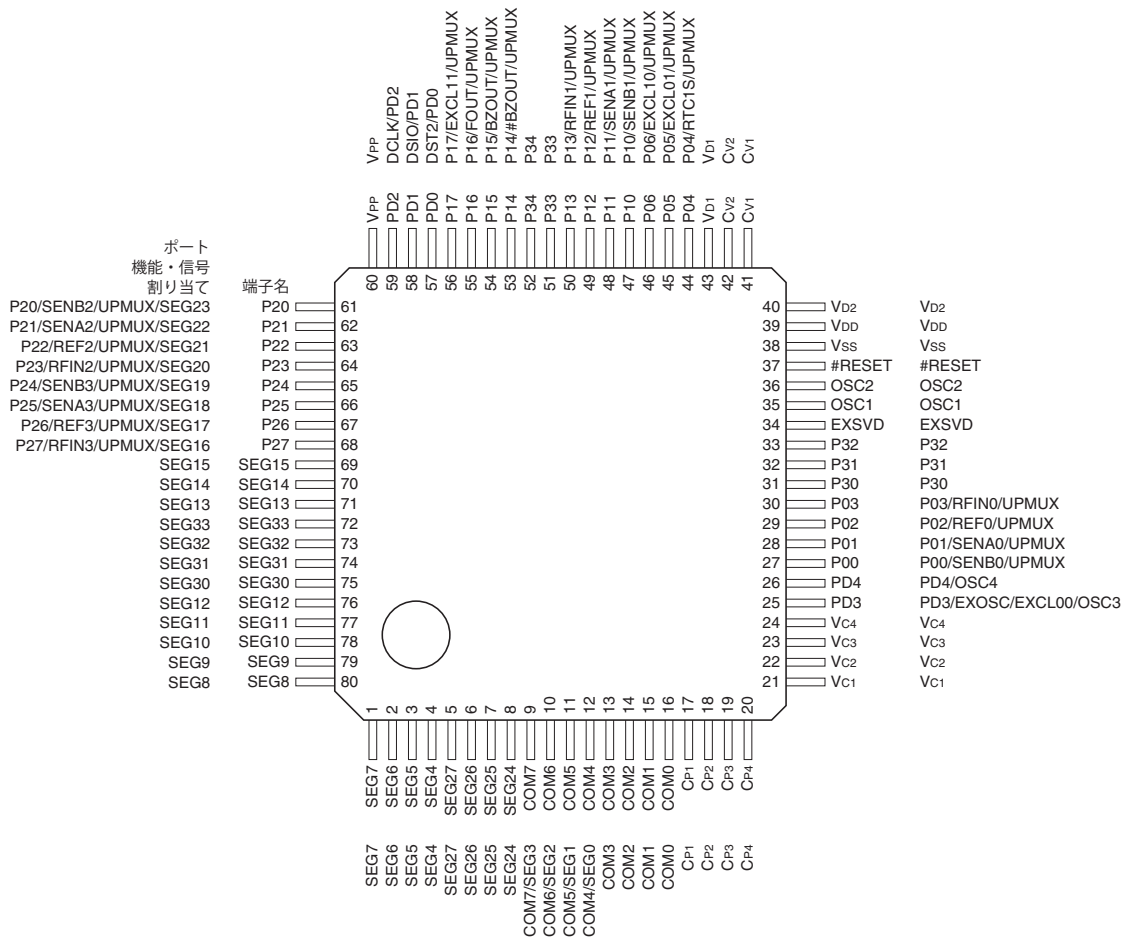
図1.3.1.3 S1C17W15端子配置図 (QFP14-80PIN)
