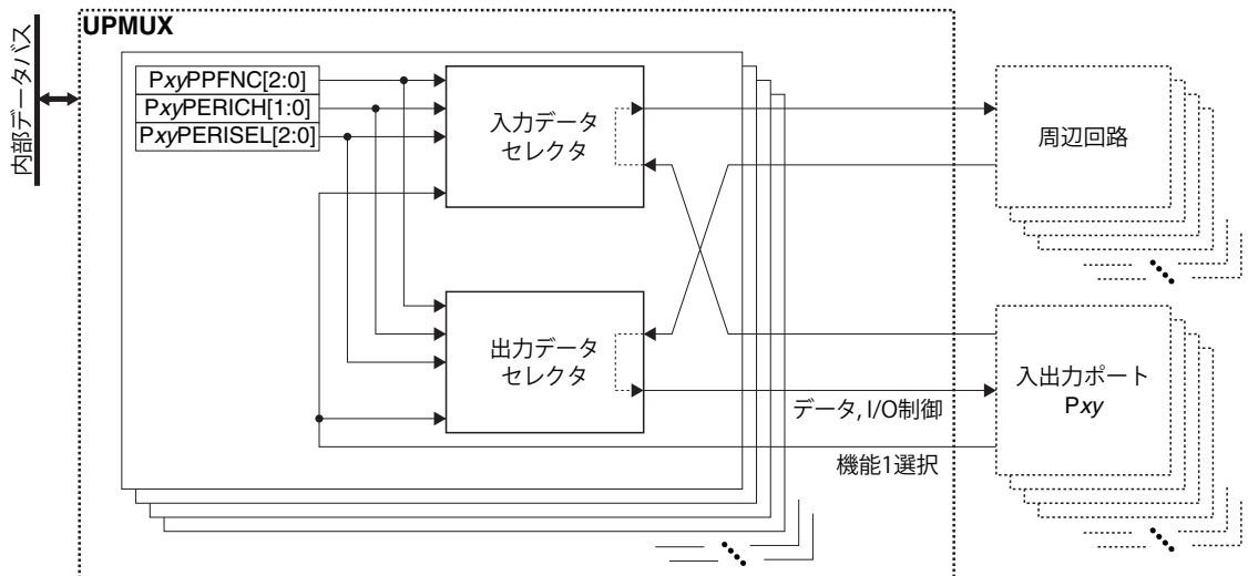
図7.1.1 UPMUXの構成
