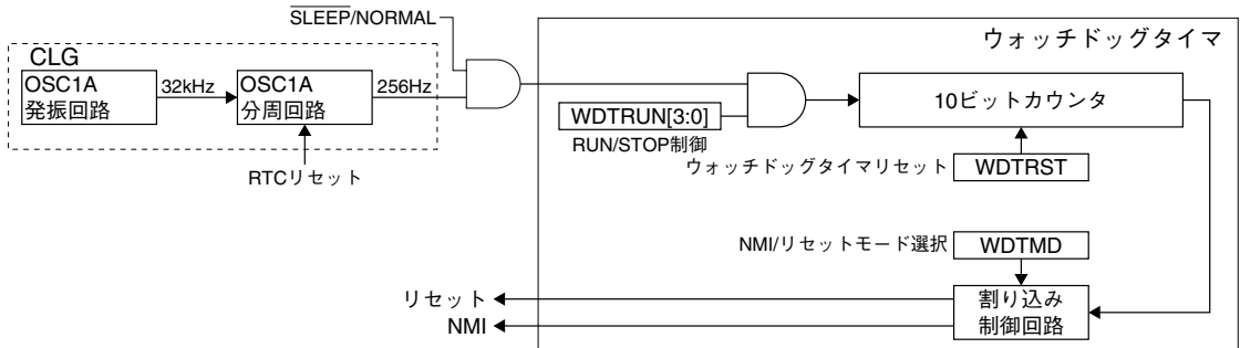
図13.1.1 WDTの構成
