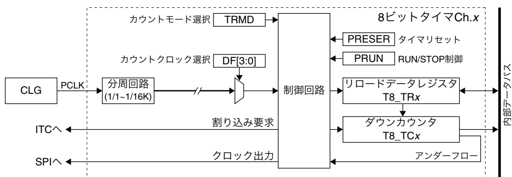
図10.1.1 T8モジュールの構成
