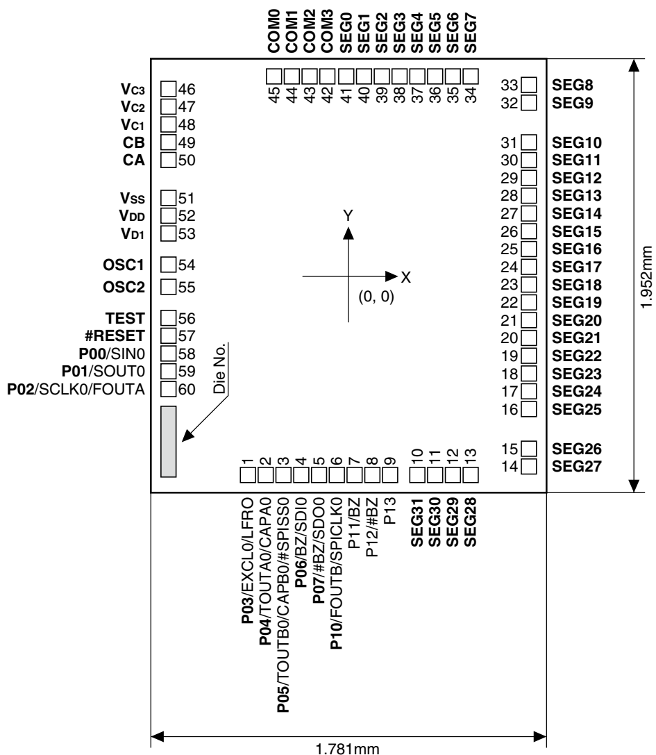
図1.3.1.1 S1C17153/パッド配置図
