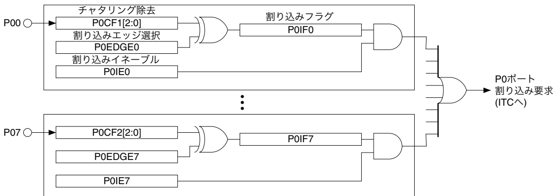
図9.5.1 ポート入力割り込み回路の構成
