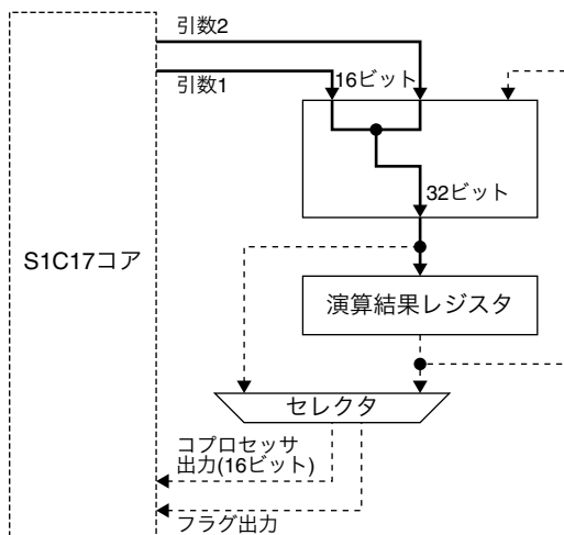
図19.5.1 初期化モード時のデータ経路
