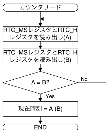
図8.3.5.1 カウンタ読み出し手順
