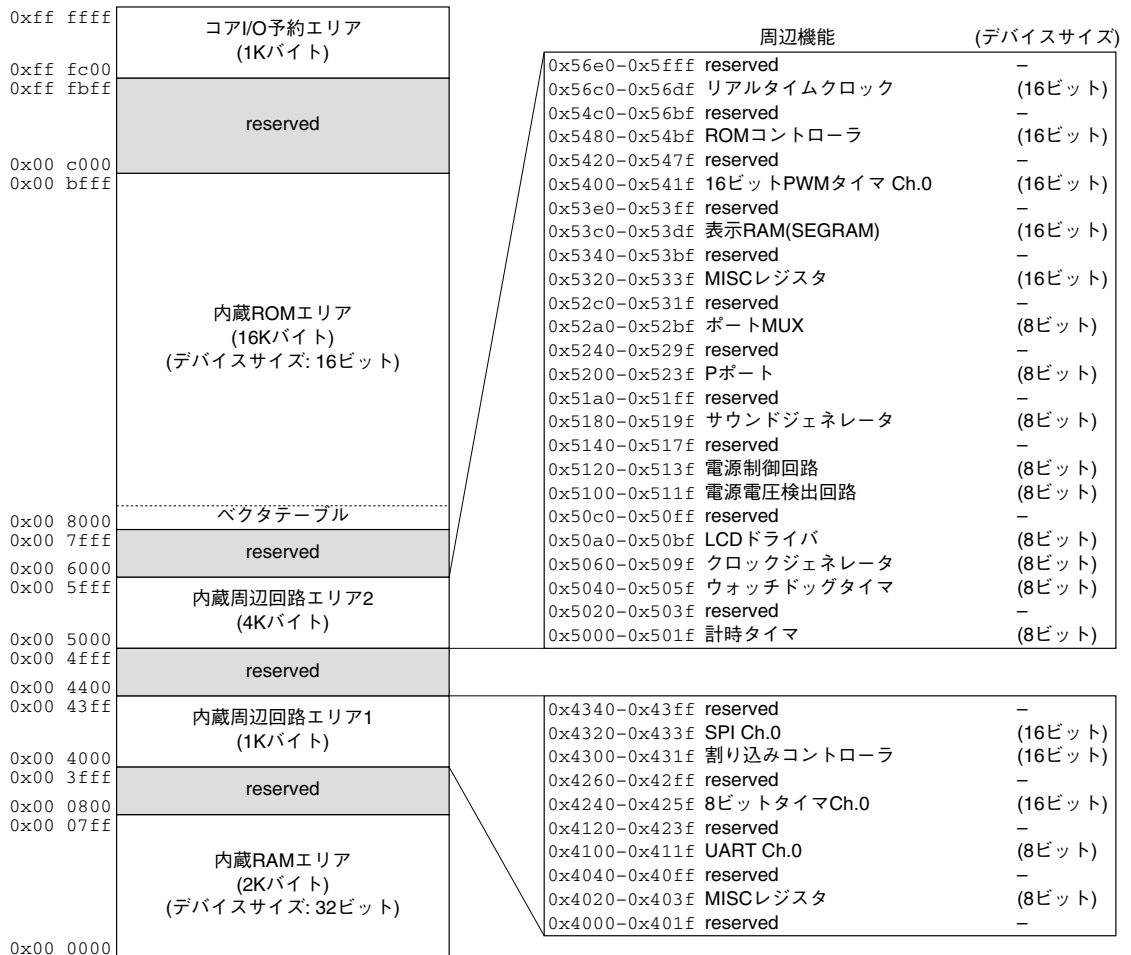
図3.1 S1C17153メモリマップ
