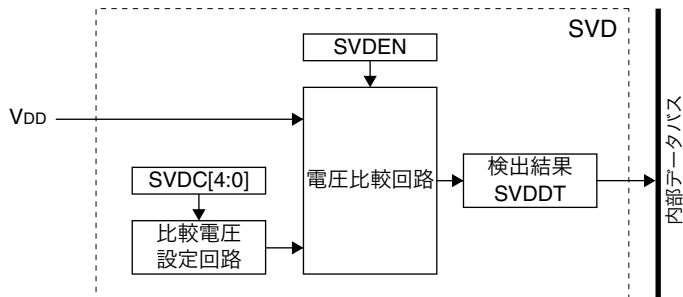
図18.1.1 SVD回路の構成
