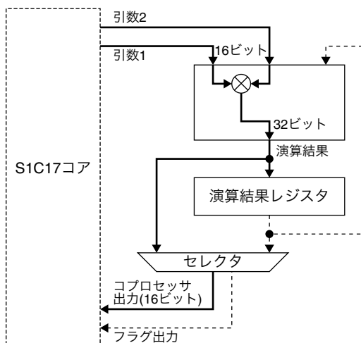
図19.3.1 乗算モードのデータ経路
