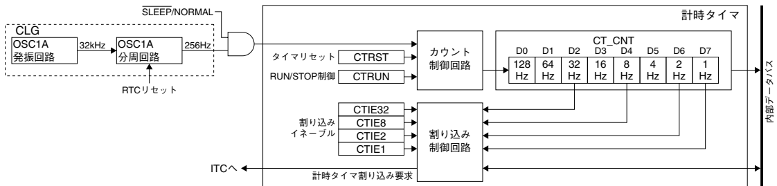
図12.1.1 CTの構成
