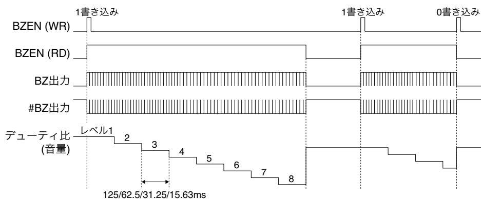
図17.5.4.1 エンベロープモードのブザー出力
