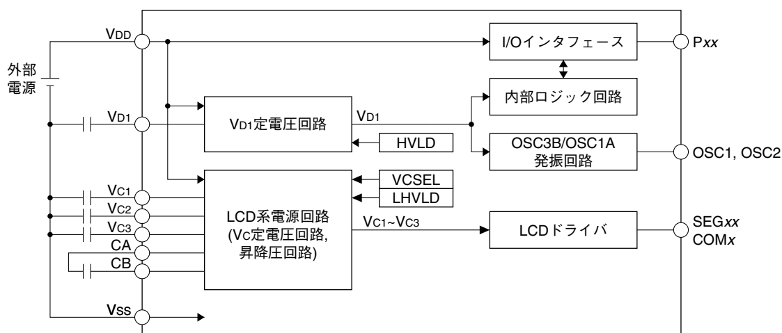
図4.2.1 内部電源回路の構成
