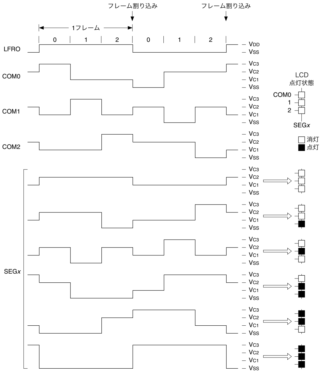
図16.4.2.2 1/3デューティ駆動波形
