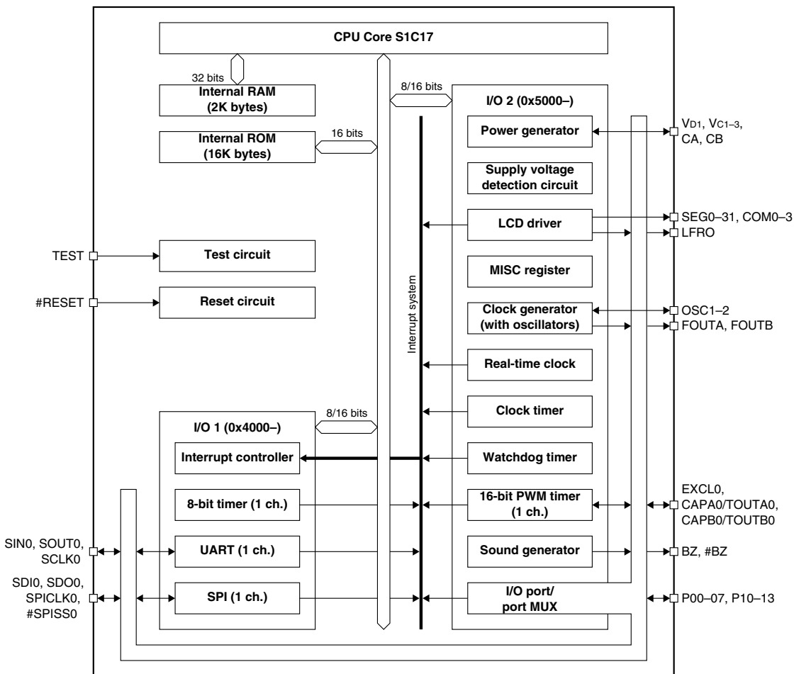
図1.2.1 S1C17153ブロック図
