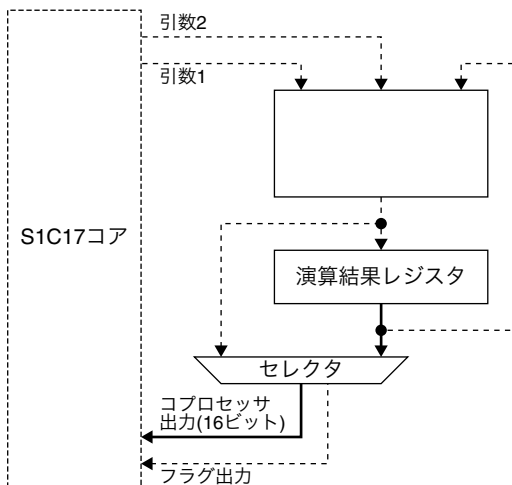
図19.6.1 演算結果読み出しモードのデータ経路
