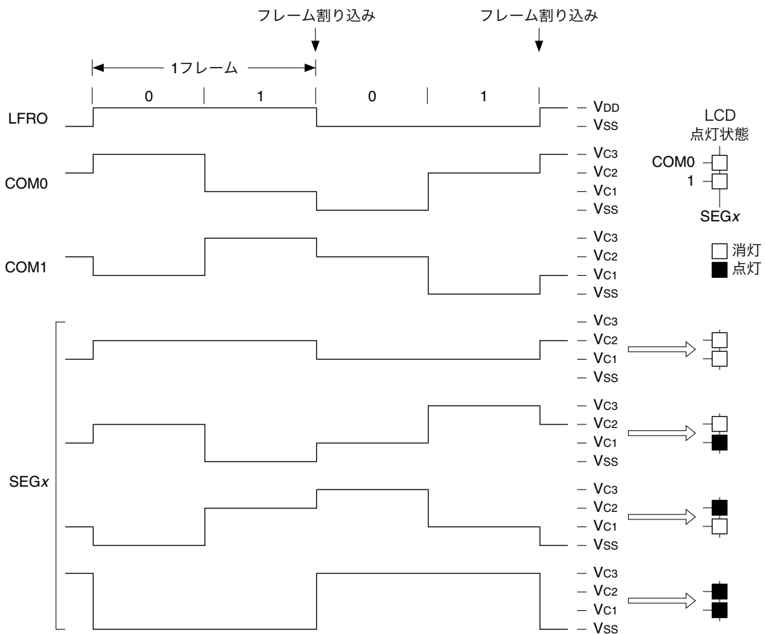
図16.4.2.3 1/2デューティ駆動波形
