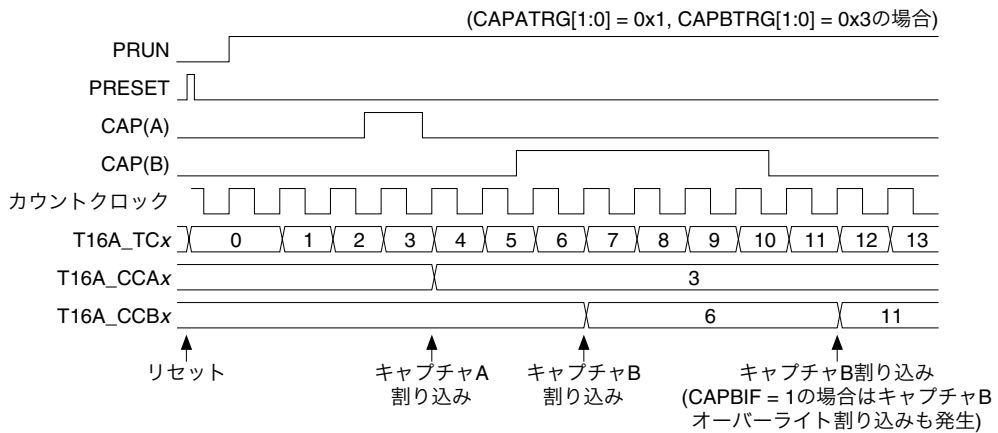
図11.5.4.2 キャプチャモード時動作タイミング
