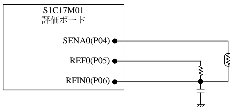
図 4.12.1 R/F 変換機サンプルプログラム ハードウェア接続図（S1C17M01）
