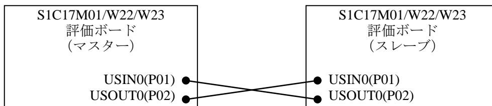
図 4.7.1 UART サンプルプログラムハードウェア接続図
