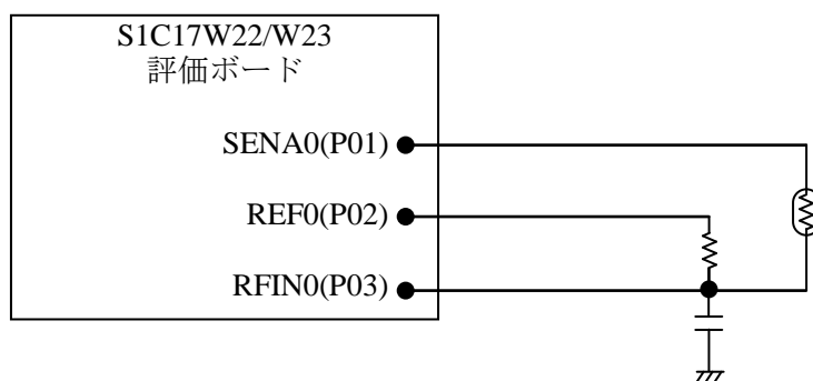
図 4.12.2 R/F 変換機サンプルプログラム ハードウェア接続図（S1C17W22/W23）
