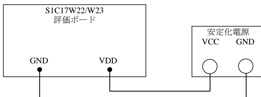
図 4.16.1 パワージェネレータサンプルプログラム ハードウェア接続図
