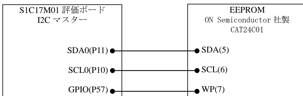
図 4.17.1 EEPROM サンプルプログラム ハードウェア接続図
