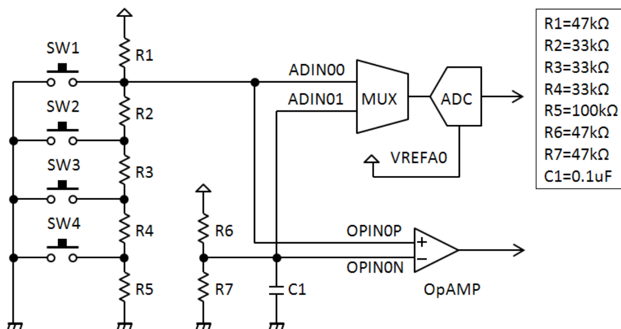
図 4.18.1 ADC,Comparator サンプルプログラム 外部接続回路
