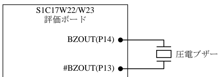
図 4.13.1 サウンドジェネレータサンプルプログラム ハードウェア接続図 (S1C17W22/W23)
