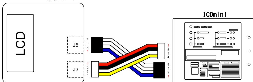
図 3.4.3 ICDmini と S5U1C17W23T との接続図
