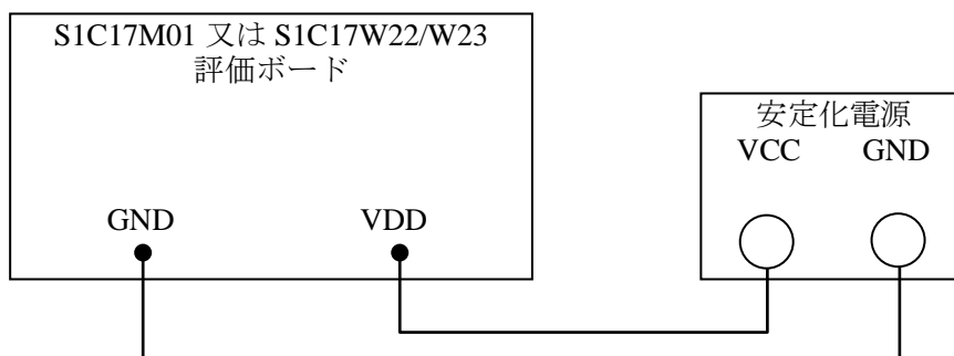
図 4.15.1 電源電圧検出回路サンプルプログラム ハードウェア接続図
