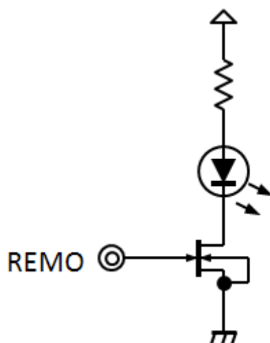
図 4.19.1 REMC サンプルプログラム 赤外発光ダイオード接続回路例
