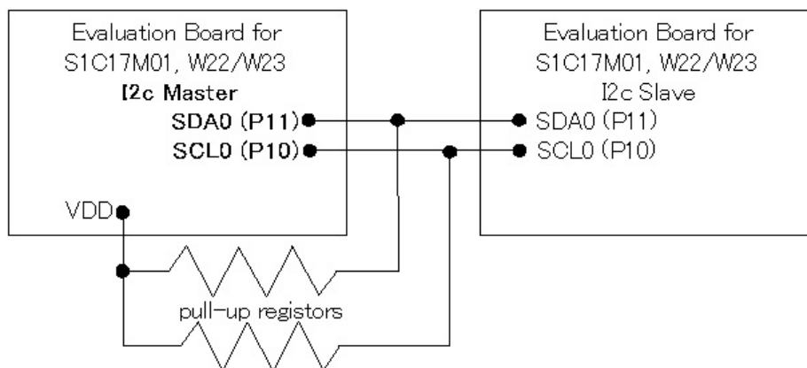
図 4.9.1 I2C マスター、スレーブサンプルプログラムハードウェア接続図
