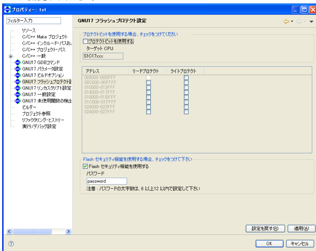
図11.2.3.1 Flash セキュリティパスワードの設定
