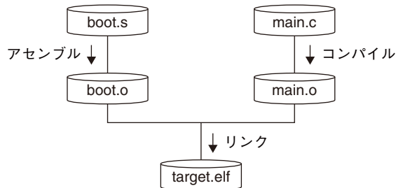
図12.1.6.1 ファイルの依存関係(例)
