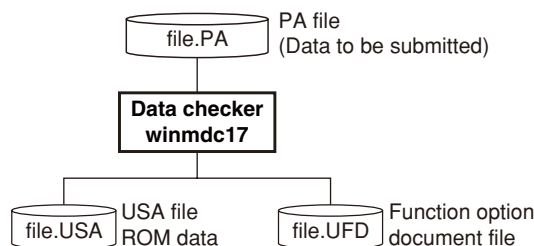
図11.2.4.1 PAファイルのアンパックフロー
