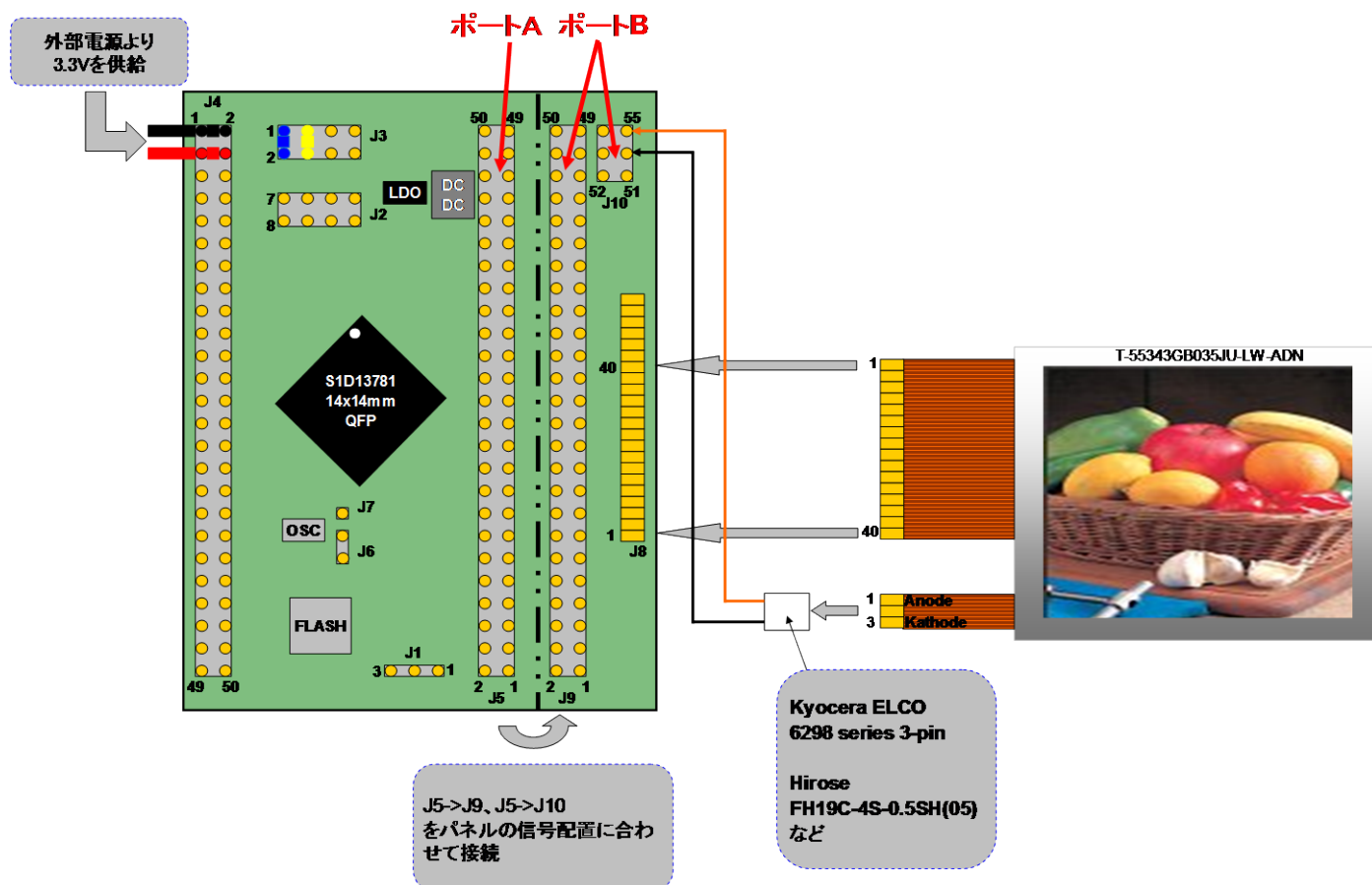
図 3-3 T-55343GD035JU-LW-ADN との接続例
