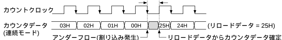
図4.9.11.3 プログラマブルタイマリロードタイミング
