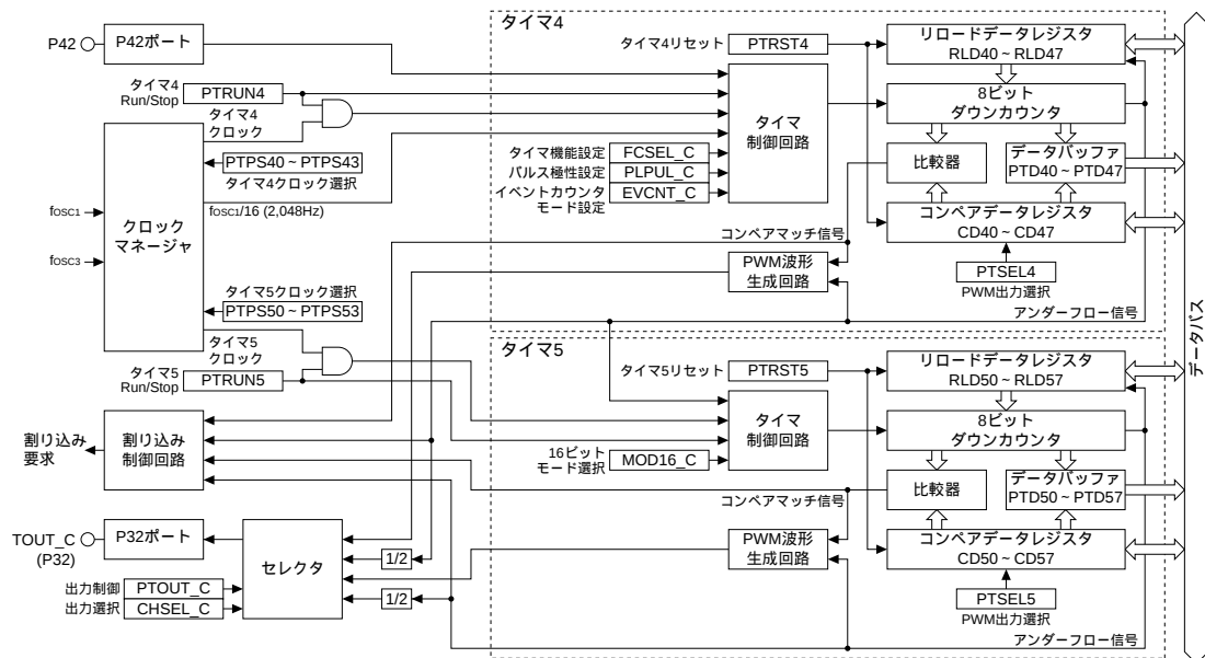
図4.9.1.3 プログラブルタイマCh. Cの構成 (タイマ4、タイマ5)
