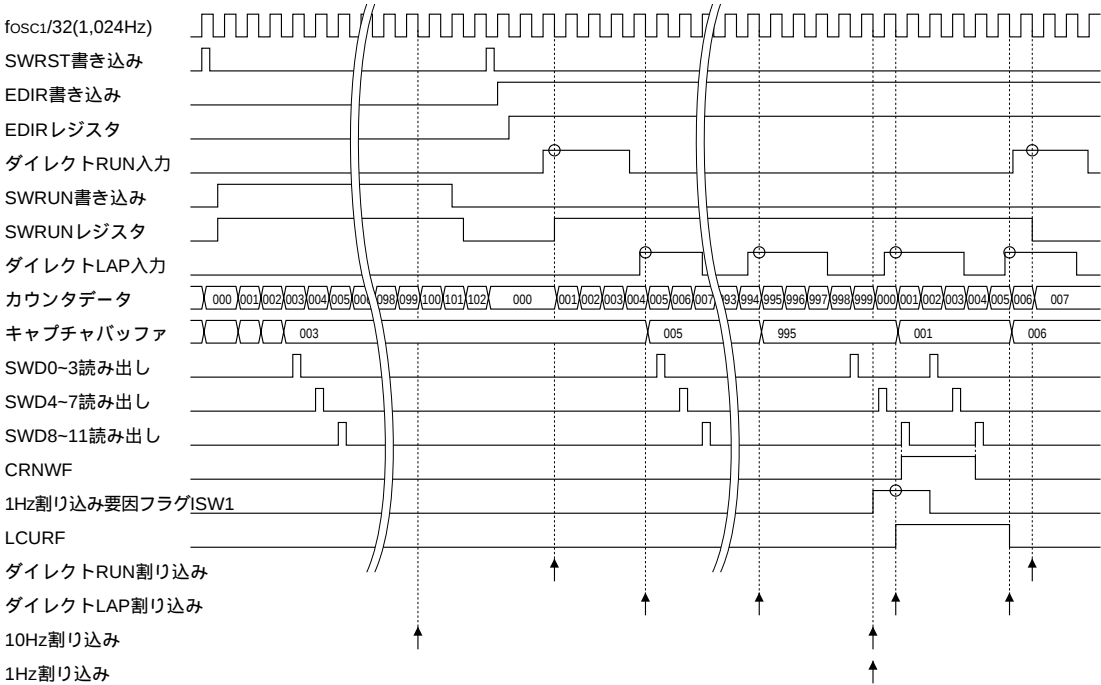
図4.8.7.2 ストップウォッチタイムのタイミングチャート
