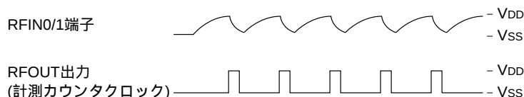
図4.13.3.2 発振波形
