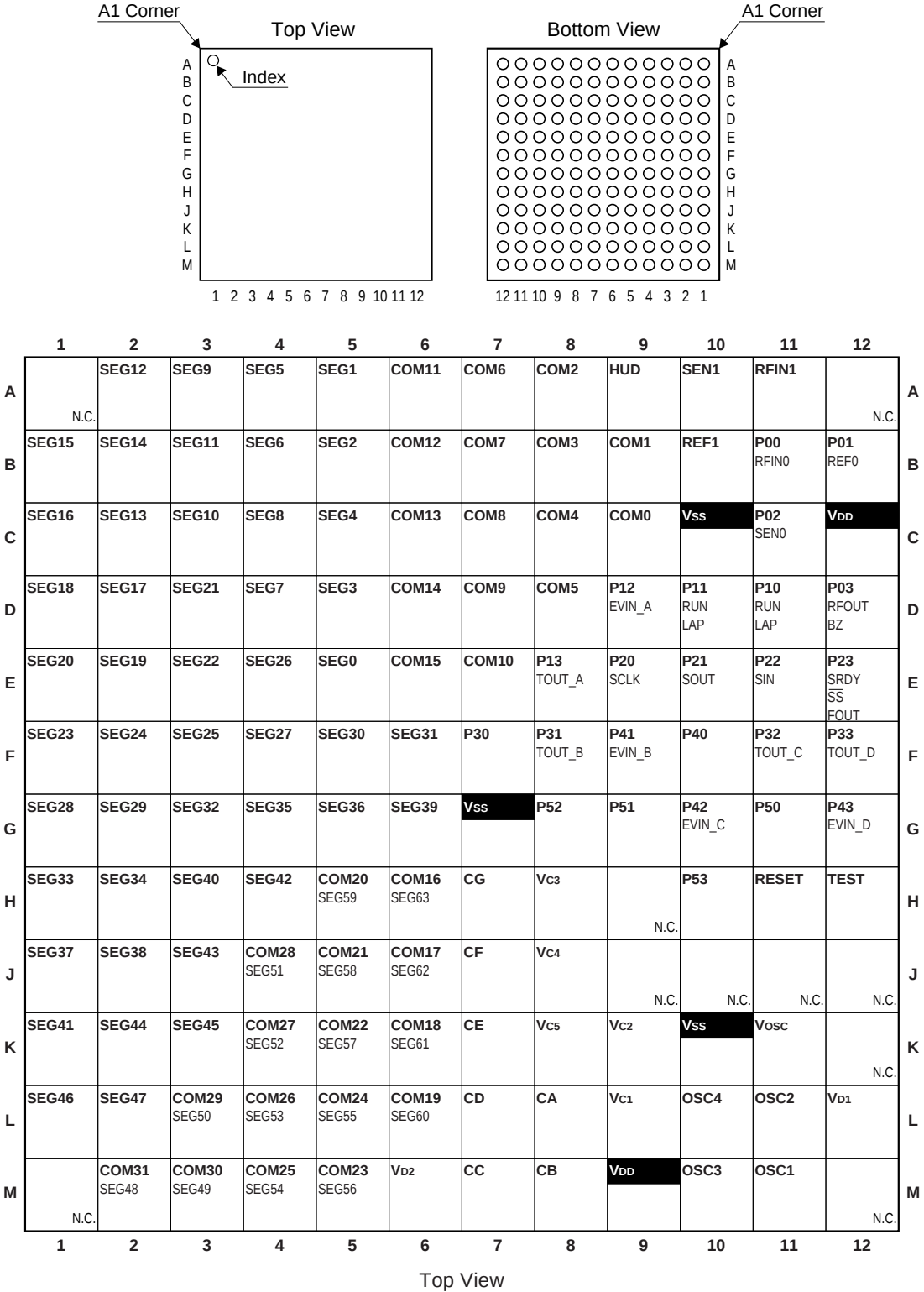
図1.3.2 端子配置図( VFBGA10H-144 )
