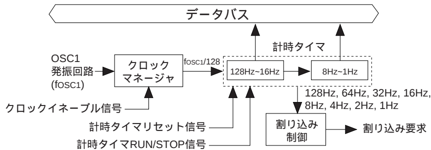
図4.7.1.1 計時タイムのブロック図
