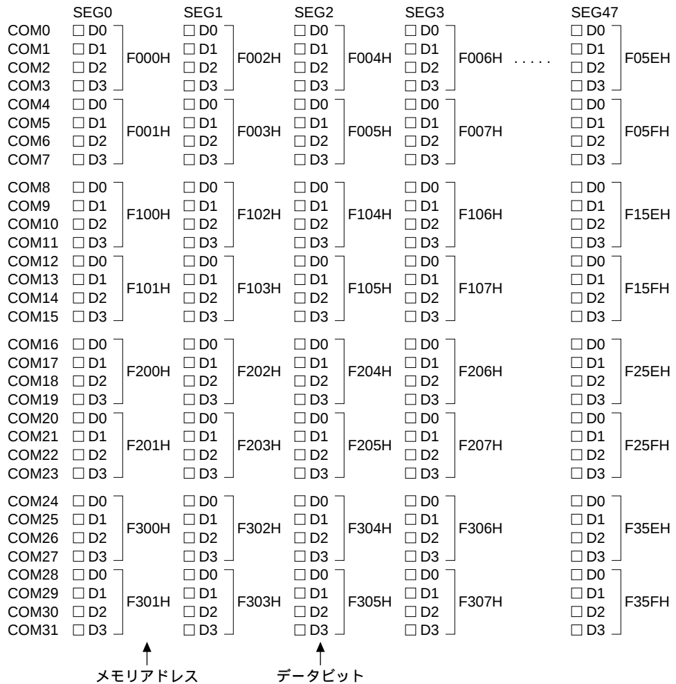
図4.6.4.1 表示メモリとLCDドットマトリクス対応 (1/32デューティ選択時)
