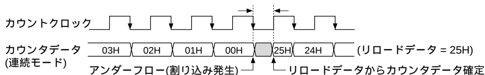
図5.2.3 プログラブルタイマリロードタイミング
