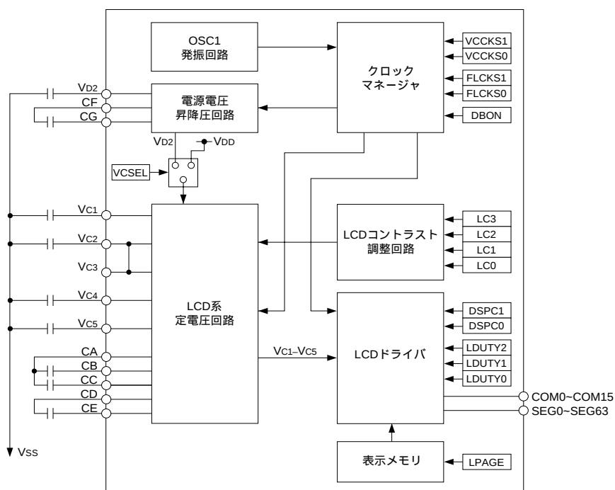
図4.6.1.2 LCDDライバと駆動電源の構成( Vc2基準, 1/4バイアスの場合 )
