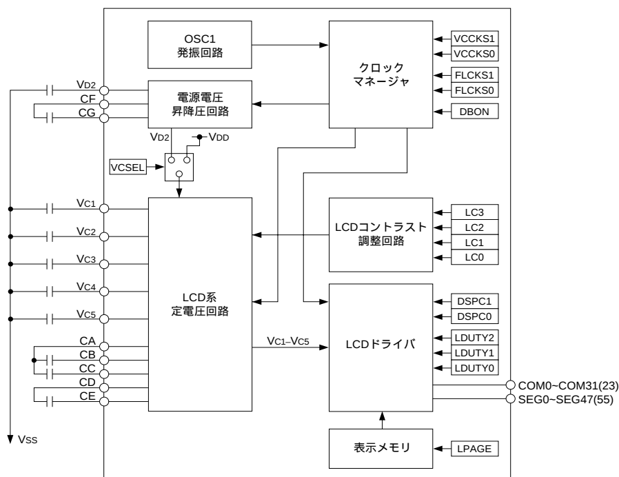
図4.6.1.1 LCDDライバと駆動電源の構成( Vc2基準, 1/5バイアスの場合 )
