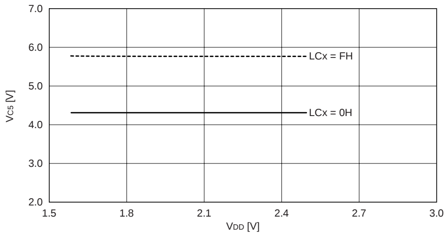
LCD駆動電圧電源電圧特性( 1/5バイアス, V_{C2} 基準, 電源電圧昇降圧回路使用時 )
