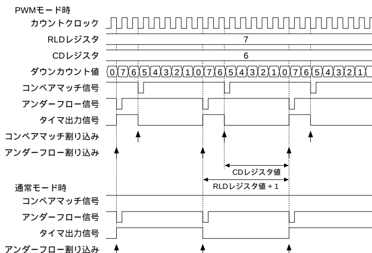
図4.9.5.1 PWM波形の生成
