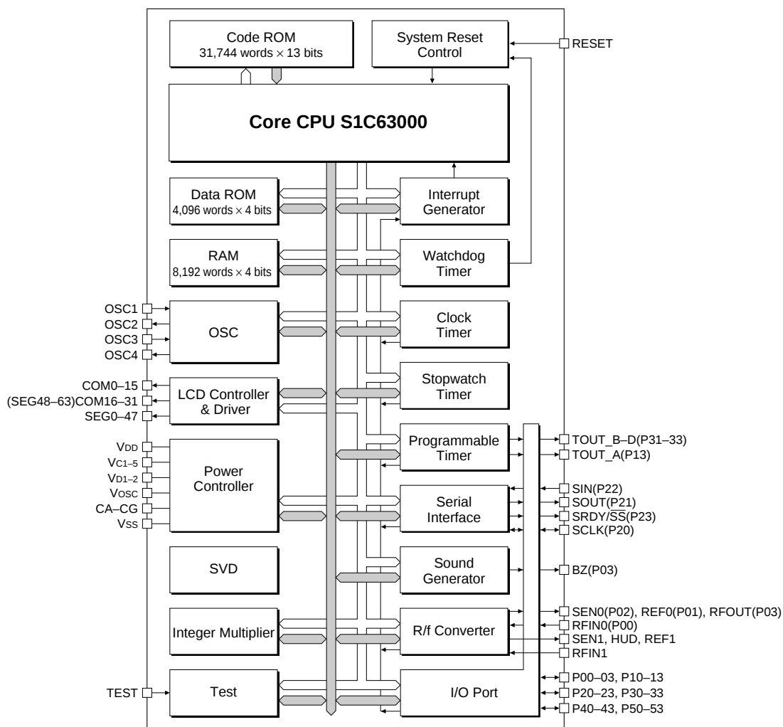
図1.2.1 ブロック図
