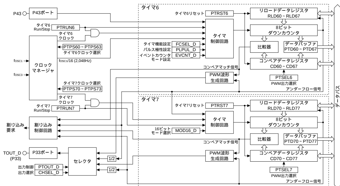
図4.9.1.4 プログラマブルタイマCh. Dの構成( タイマ6、タイマ7 )
