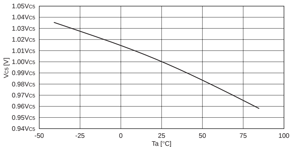
LCD駆動電圧温度特性( 1/4バイアス, V_{C2} 基準, 電源電圧昇降圧回路未使用時)
