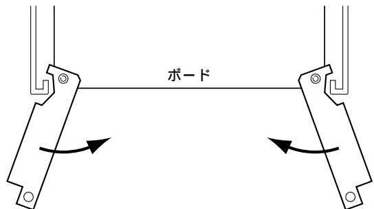
図A.2.2 ボードの装着
