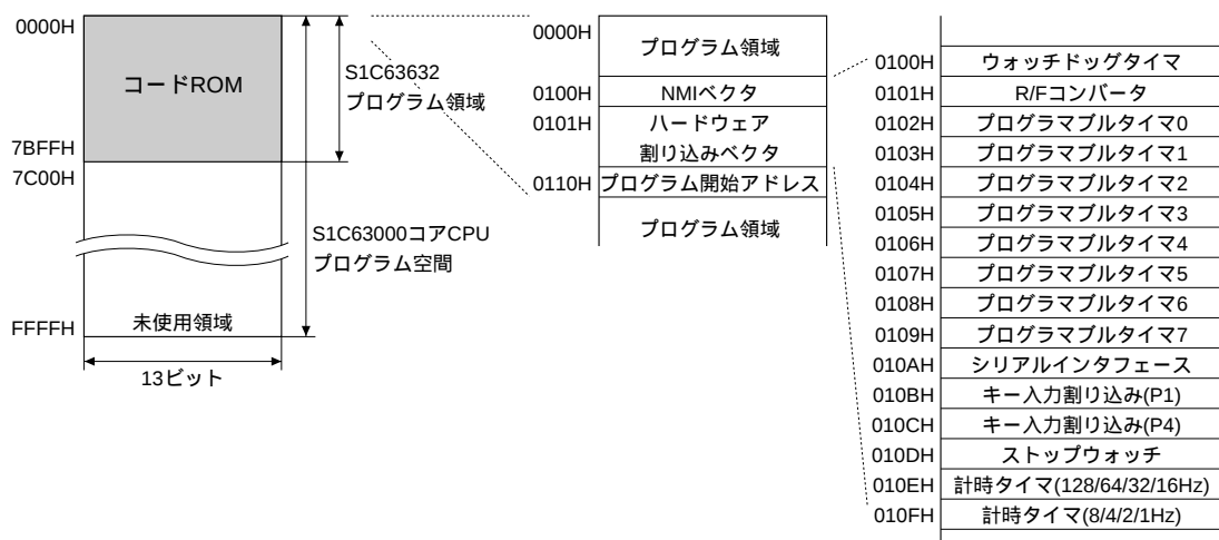
図3.2.1 コードROMの構成
