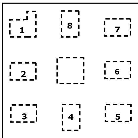
図 2 端子配置図
