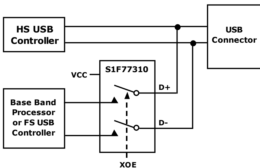
図 1 応用回路例
