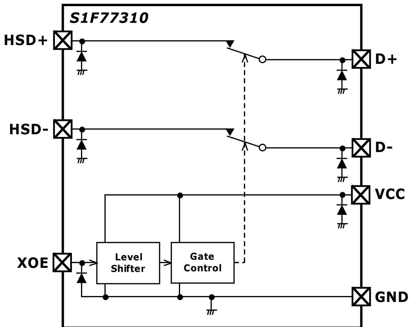
図 4 ブロック図
