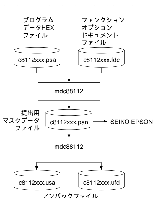
図3.3.2.1 mdc88112の実行フロー
