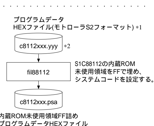
図3.1.2.1 fil88112の実行フロー
