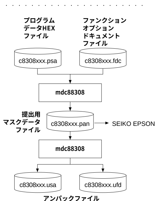
図3.3.2.1 mdc88308の実行フロー
