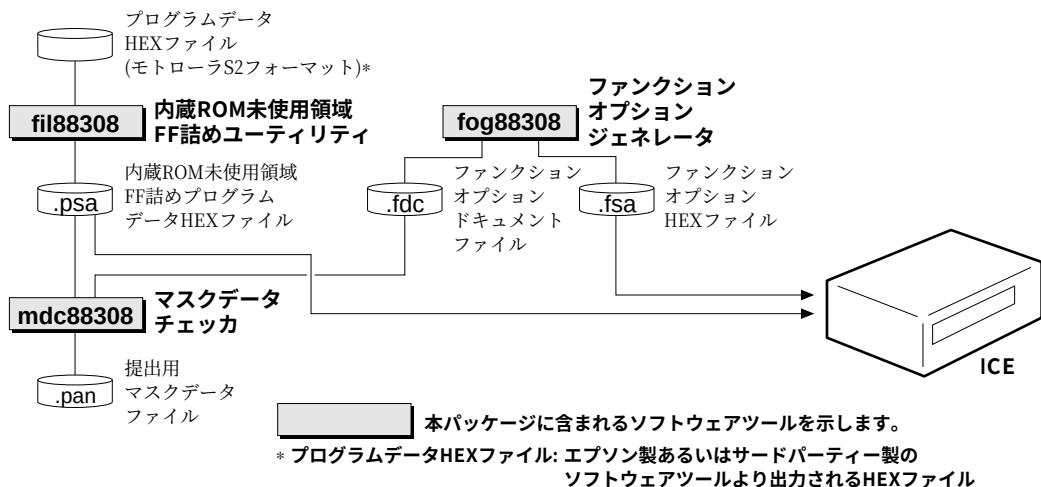
図1.3.1 ソフトウェア開発フロー
