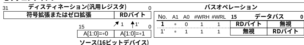
図4.12 16ビットデバイスからのバイトデータ読み込み
