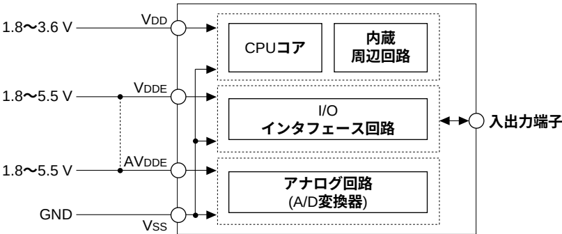
図 2.1.1 電源系
