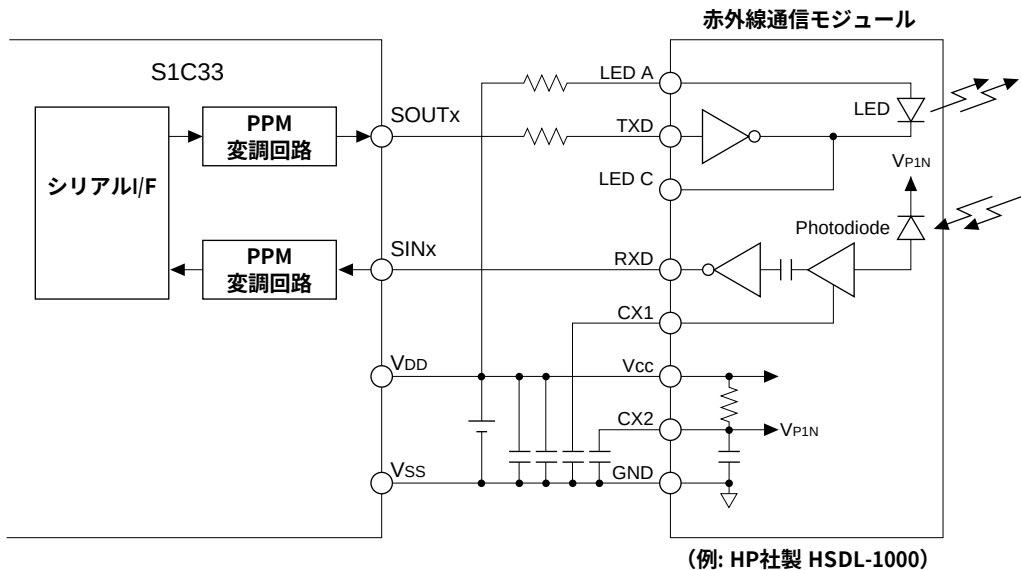
図8.14 IrDAインタフェースの構成例
