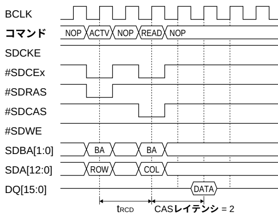
図2.5 CASレイテンシ
