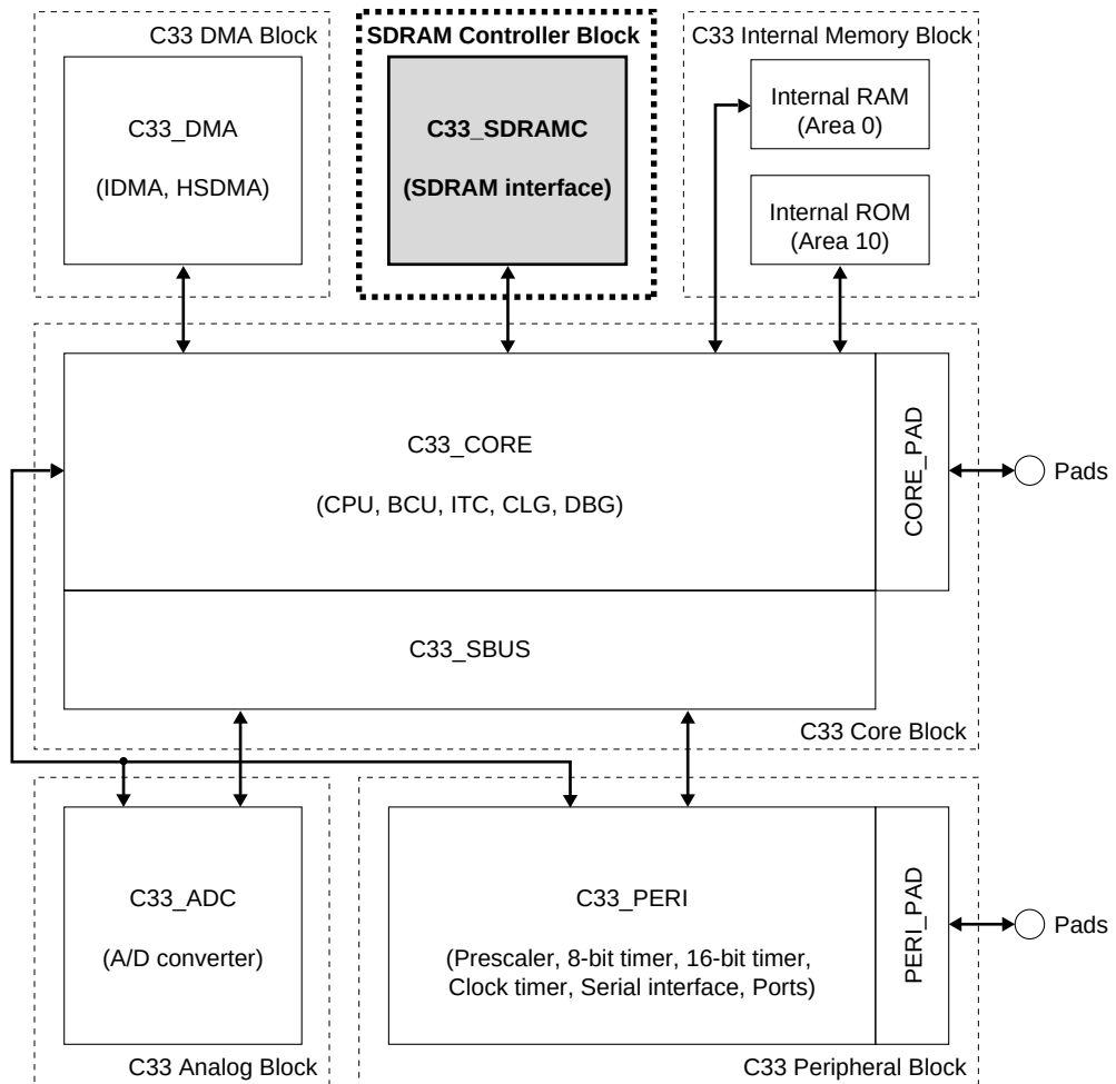
図1.1 SDRAMコントローラブロック
