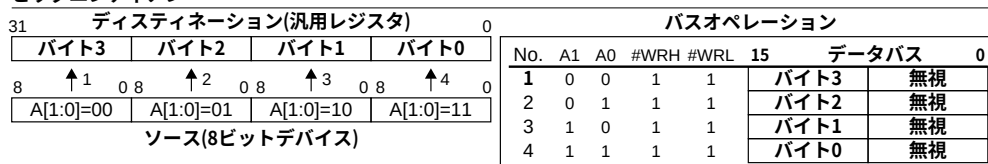
図4.14 8ビットデバイスからのワードデータ読み込み
