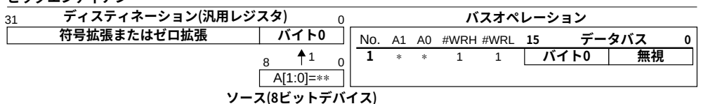
図4.18 8ビットデバイスからのバイトデータ読み込み
