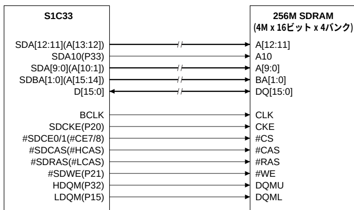
図2.2 16ビットSDRAMの接続例(32MB x 1)
