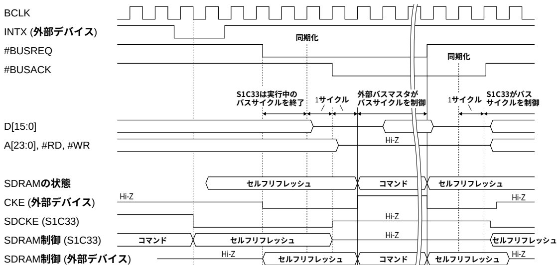
図2.14 バス解放手順
