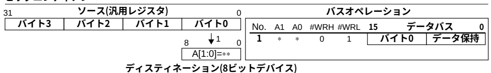
図4.17 8ビットデバイスへのバイトデータ書き込み
