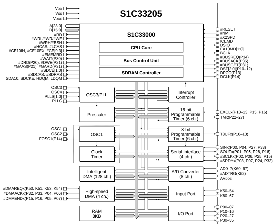
図 1.2.1 S1C33205ブロック図
