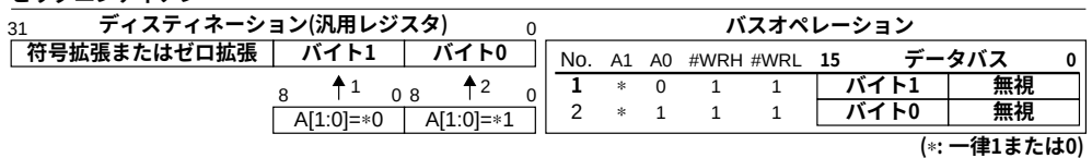
図4.16 8ビットデバイスからのハーフワードデータ読み込み
