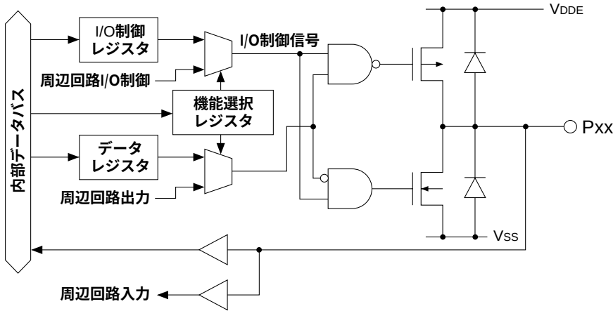
図9.2 入出力兼用ポートの構造
