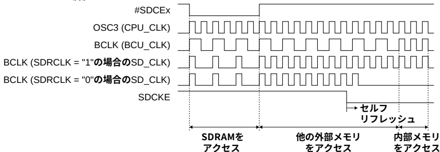
図2.9 SDRAMクロック出力
