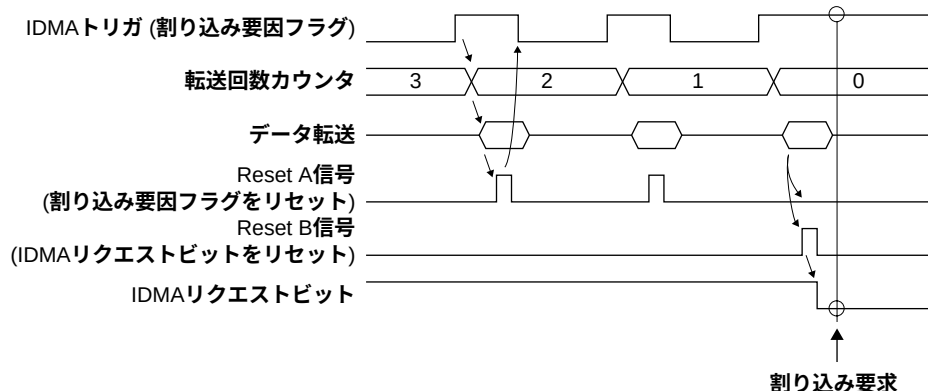
図5.2 DINTEN="1"の場合の制御
