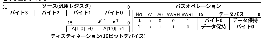
図4.11 16ビットデバイスへのバイトデータ書き込み
