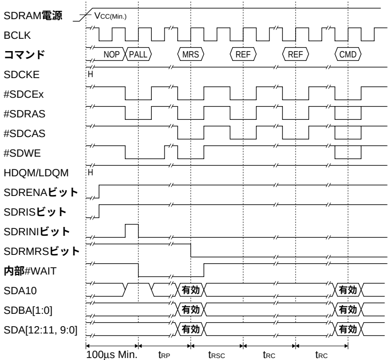
図2.10 SDRAMパワーアップと初期化
