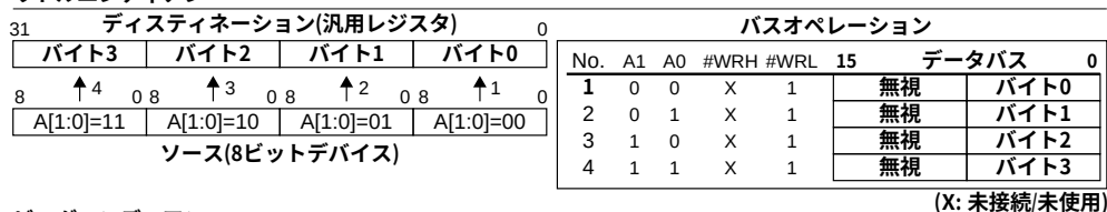
図4.13 8ビットデバイスへのワードデータ書き込み
