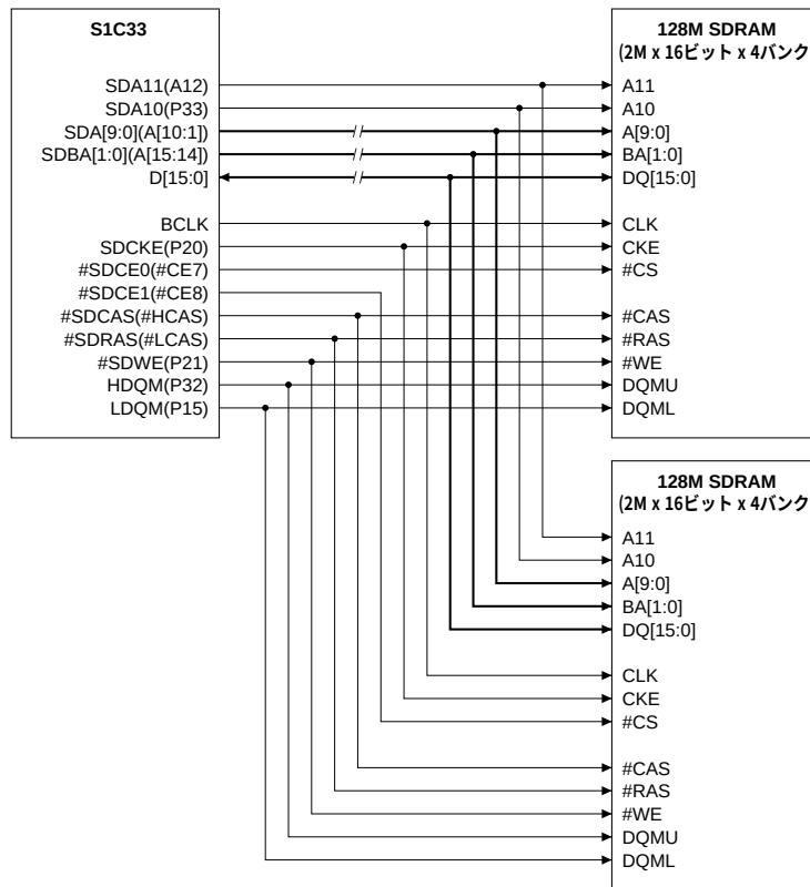
図2.3 16ビットSDRAMの接続例(16MB x 2)
