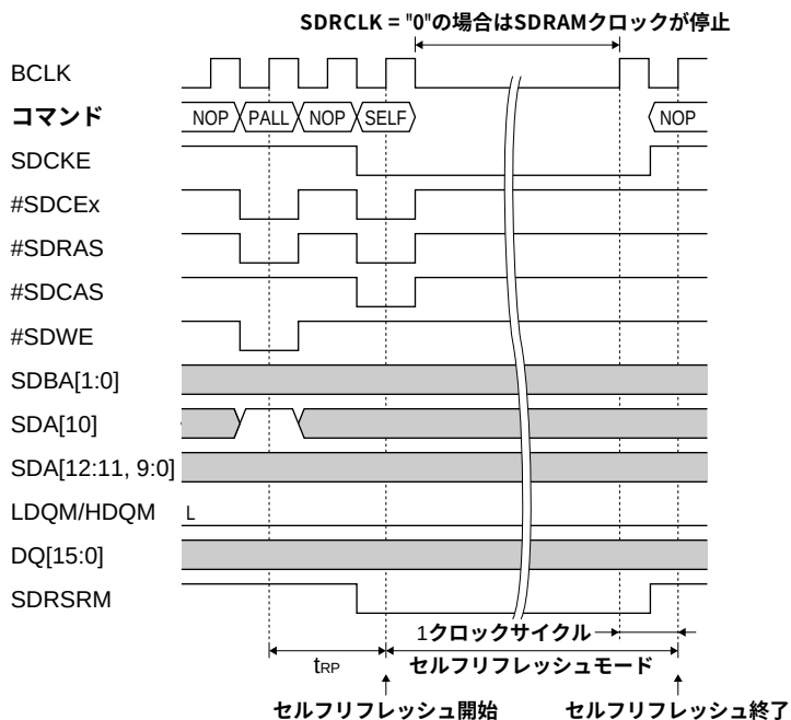
図2.13 セルフリフレッシュ
