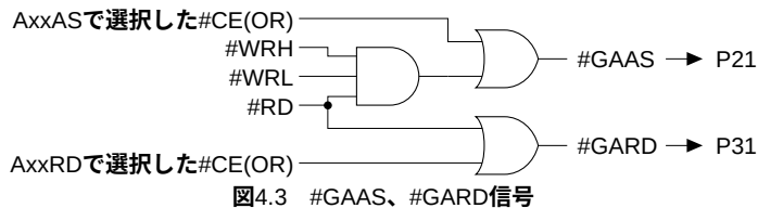
図4.3 #GAAS、#GARD信号
