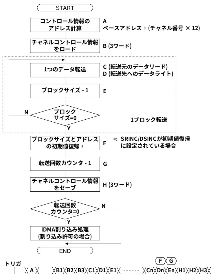
図3.3 ブロック転送モードの動作フロー
