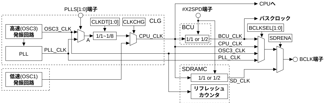
図2.8 SDRAMクロック出力回路
