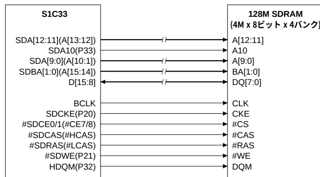
図2.4 8ビットSDRAMの接続例(16MB x 1)
