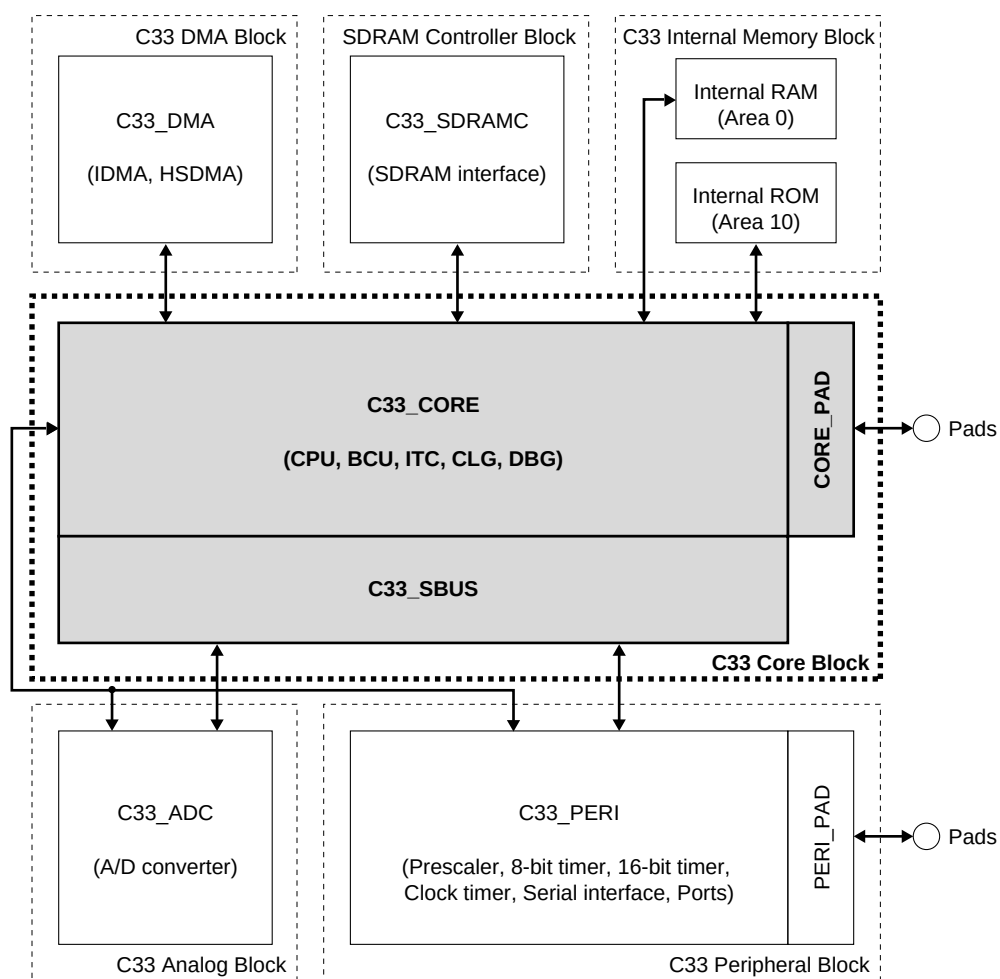
図1.1 コアブロック
