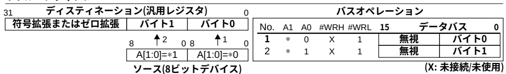
図4.15 8ビットデバイスへのハーフワードデータ書き込み
