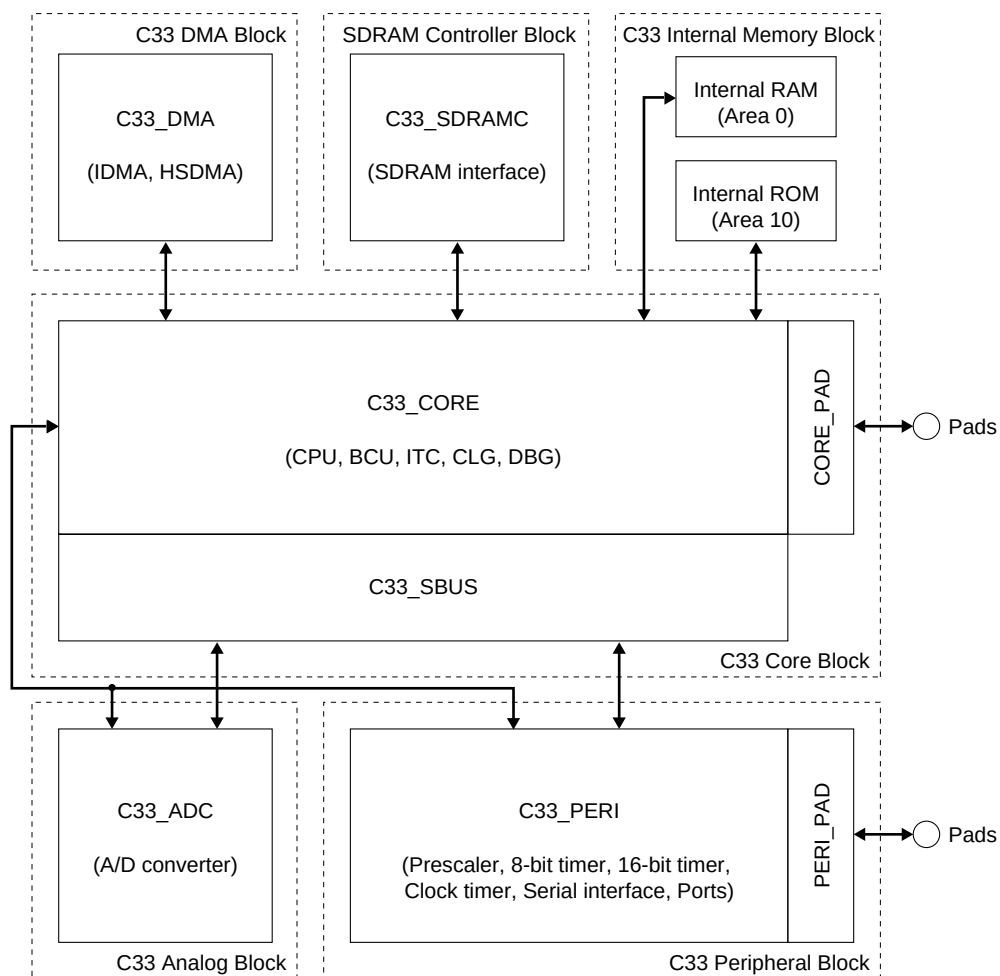
図2.1 ブロック構成
