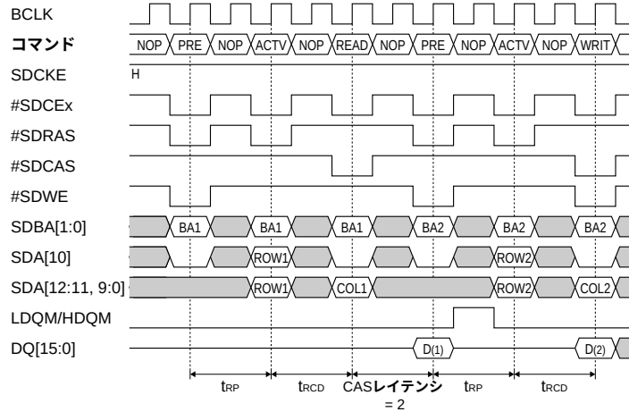
図2.11 シングルリード→シングルライト(ページ変更)
