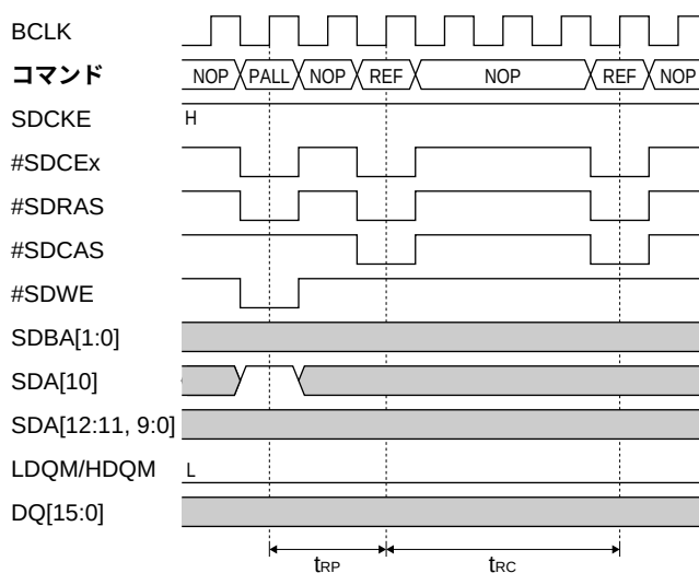
図2.12 オートリフレッシュ
