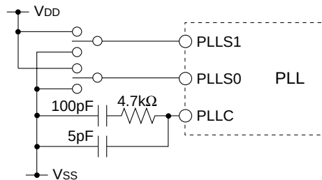
図6.3 PLL使用時の基本外部結線図
