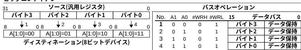
図4.13 8ビットデバイスへのワードデータ書き込み
