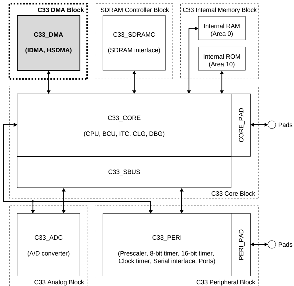
図1.1 DMAブロック
