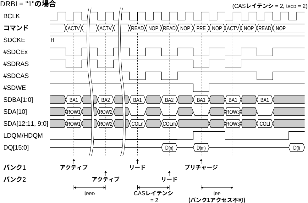
図2.6 バンクインターリーブアクセス
