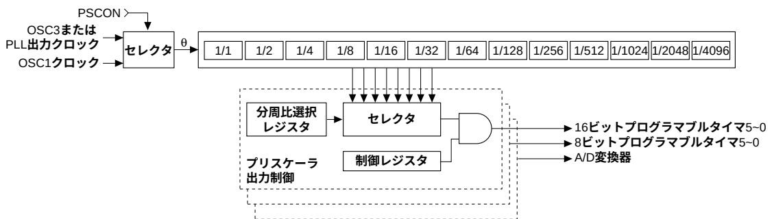
図2.1 プリスケーラとクロック制御回路の構成
