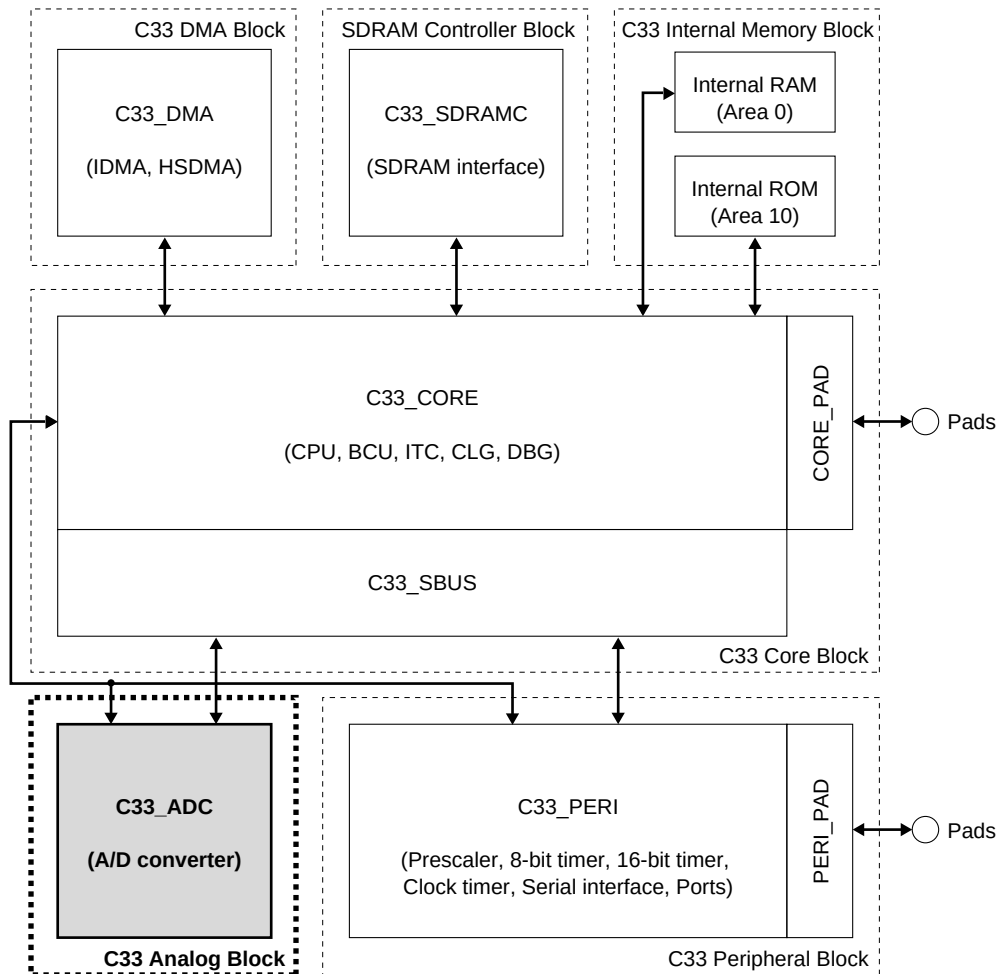
図1.1 アナログブロック
