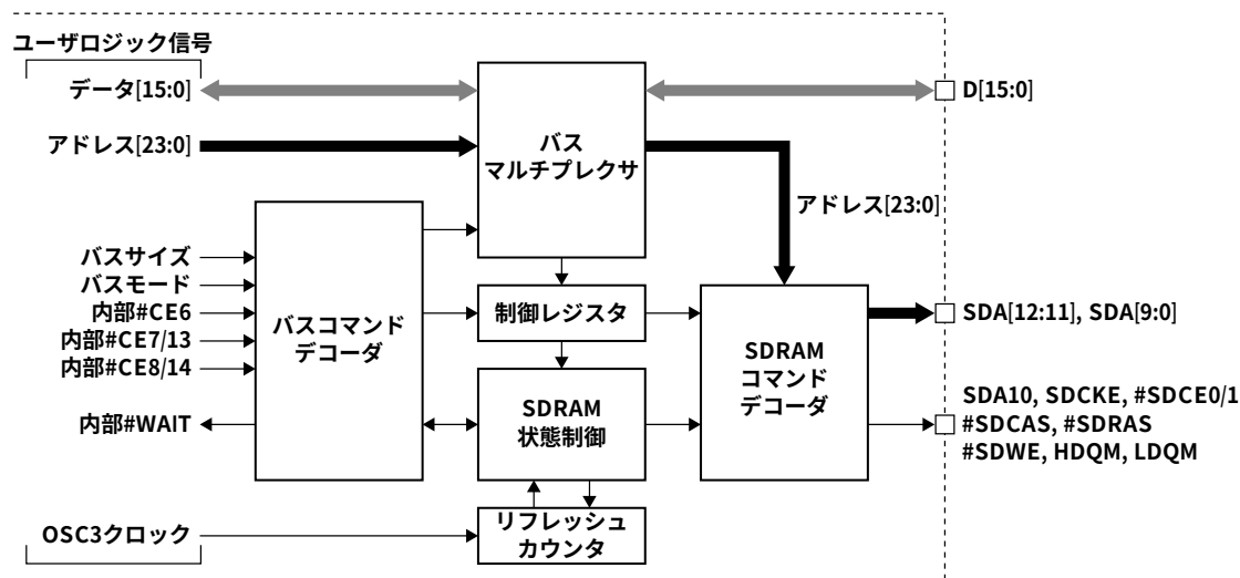
図2.1 SDRAMコントローラブロック図
