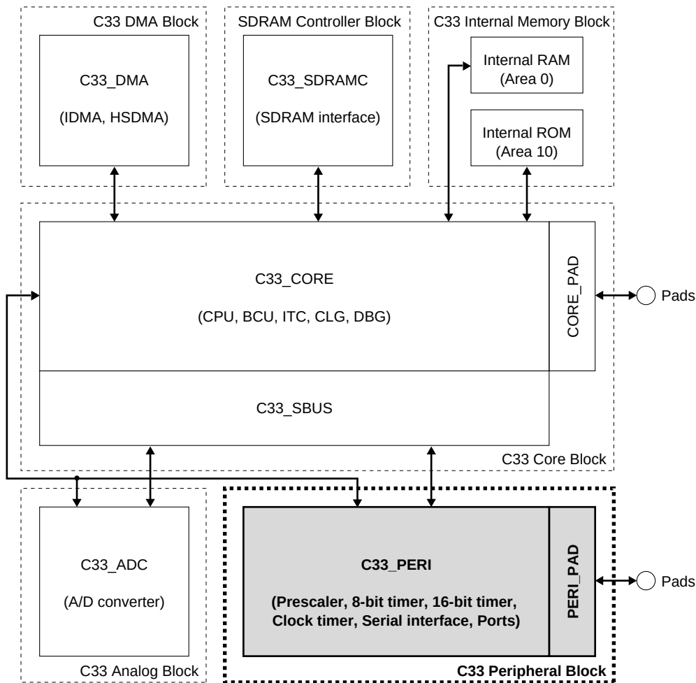
図1.1 周辺回路ブロック
