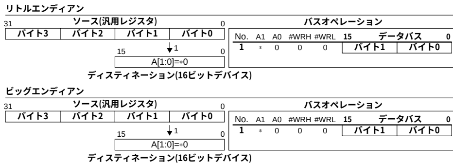
図4.9 16ビットデバイスへのハーフワードデータ書き込み
