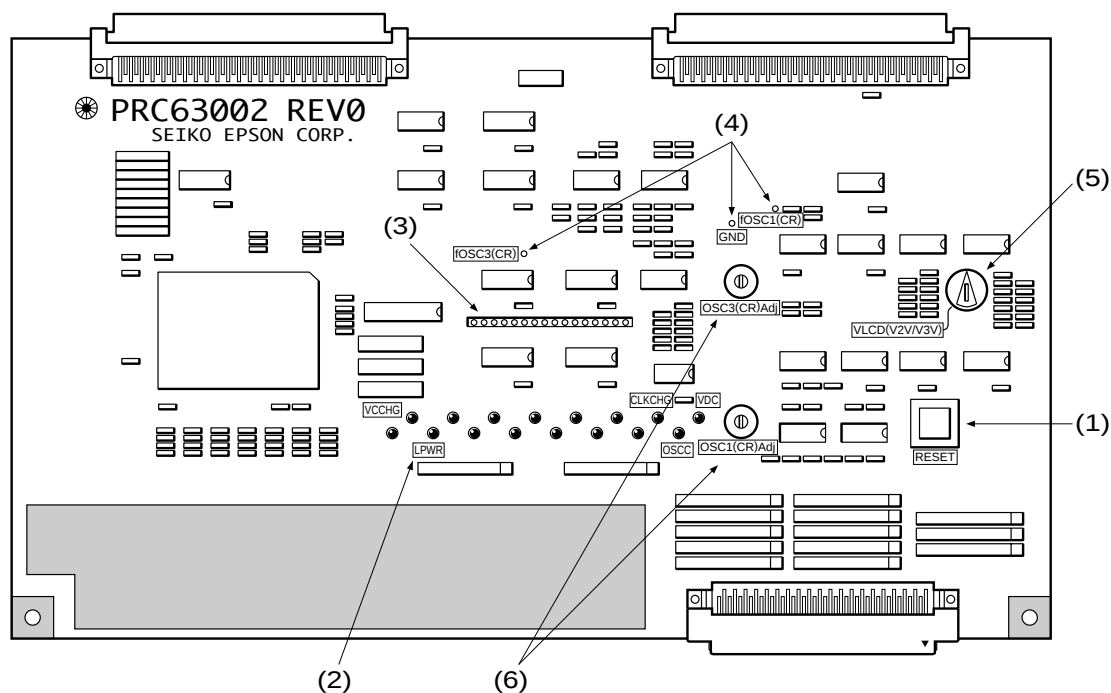
図4.1 上面図
