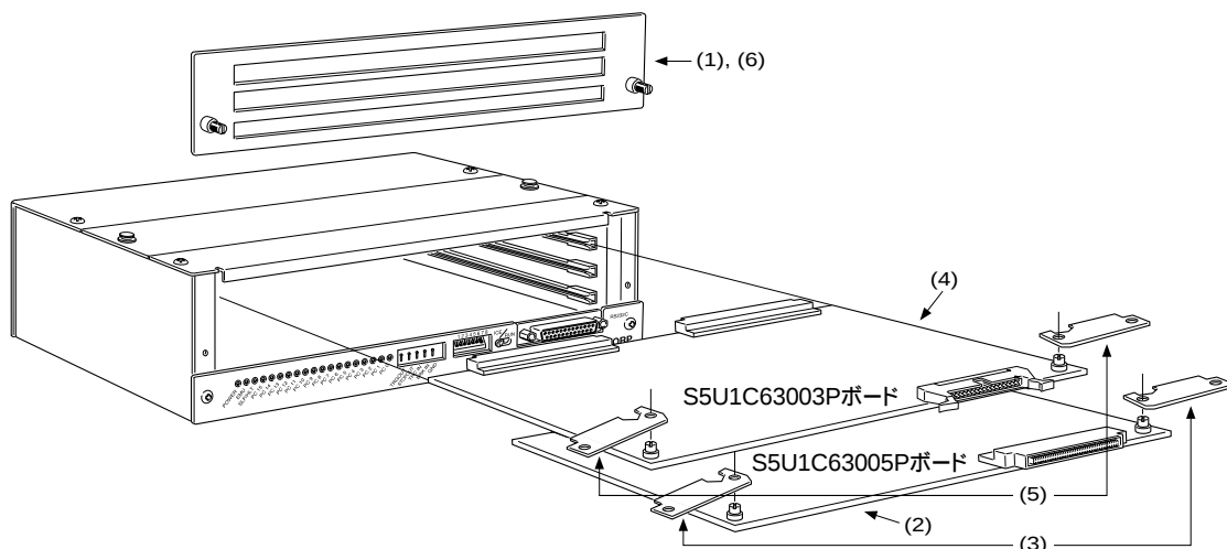
図2.1.1 S5U1C63005Pの実装
