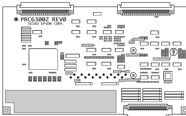
図1.3.1 S5U1C63005Pボード外形図
