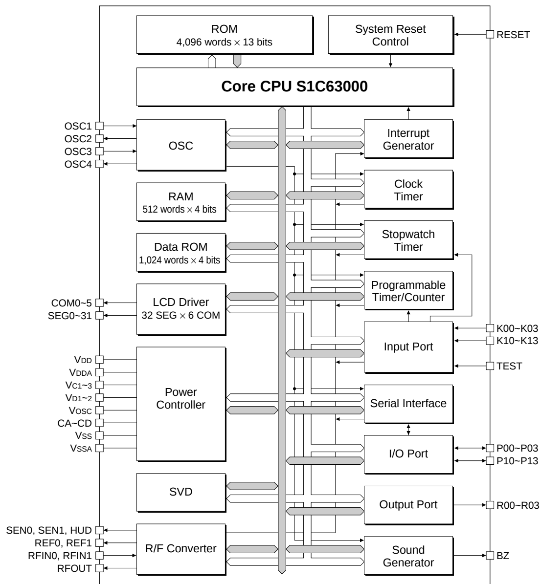
図1.2.1 ブロック図
