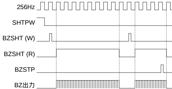
図4.13.5.1 1ショット出力のタイミングチャート
