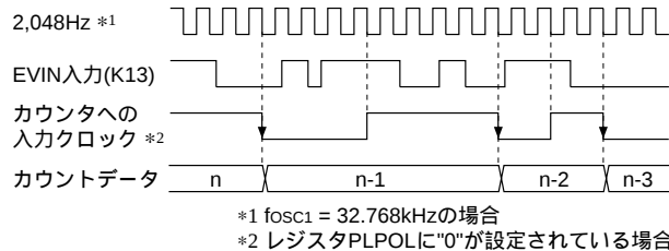
図4.11.4.2 ノイズリジェクタ付加時のダウンカウントタイミング
