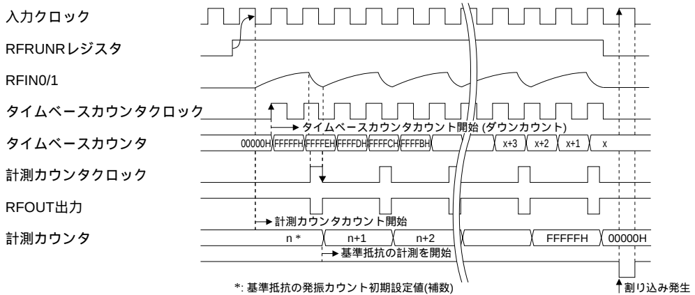
図4.14.3.1 基準発振タイミングチャート
