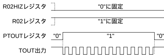
図4.11.8.2 TOUT信号の出力波形
