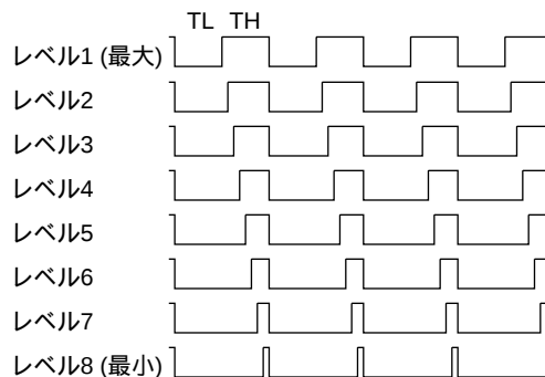
図4.13.3.1 ブザー信号波形のデューティ比
