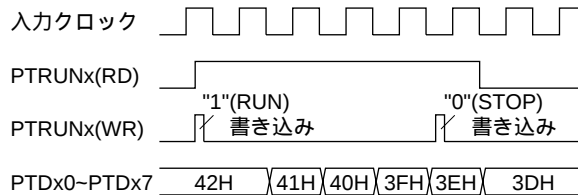
図4.11.11.1 RUN/STOP制御のタイミングチャート
