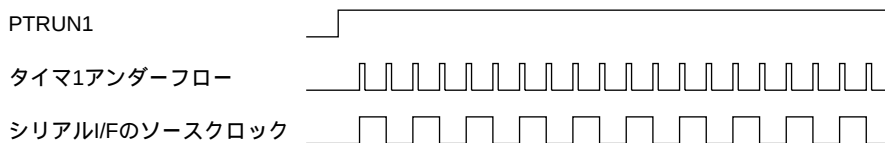
図4.11.9.1 シリアルインタフェースの同期クロック
