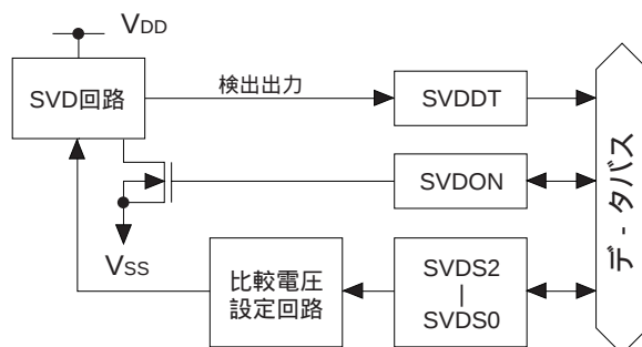
図4.15.1.1 SVD回路の構成
