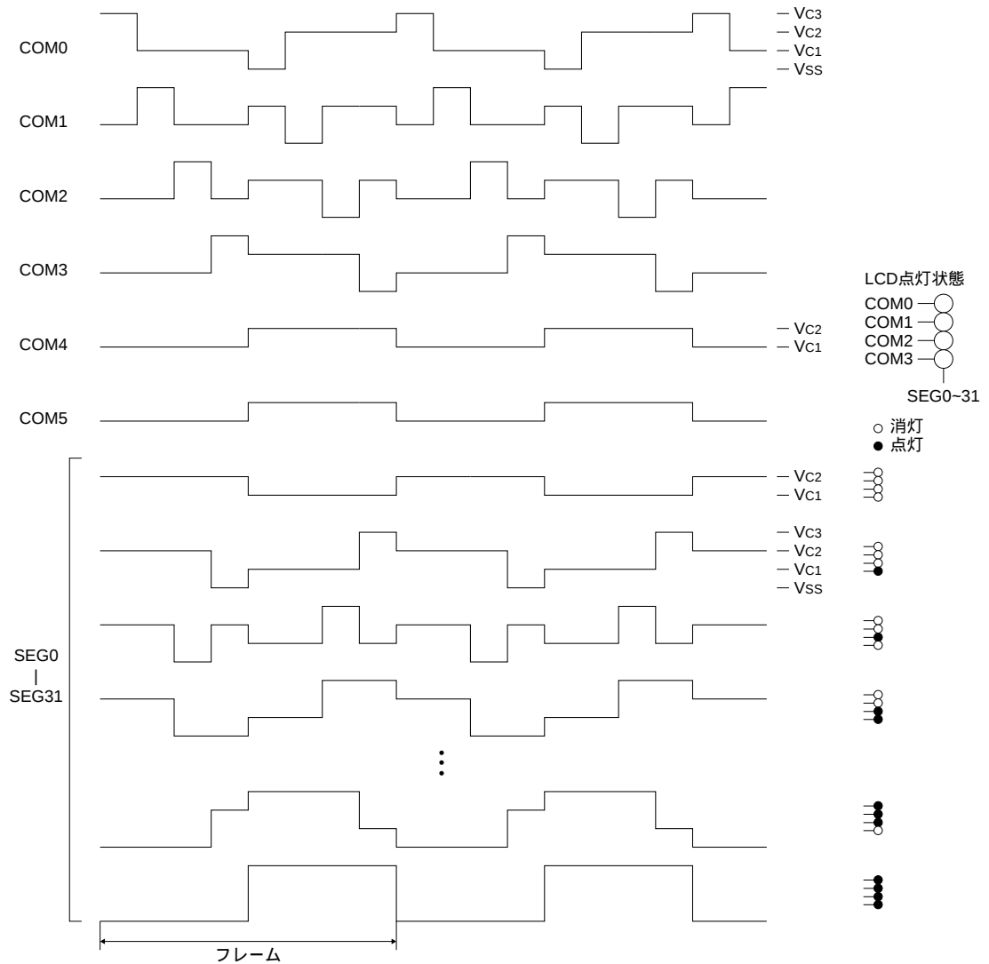
図4.8.3.3 1/4デューティLCD駆動波形
