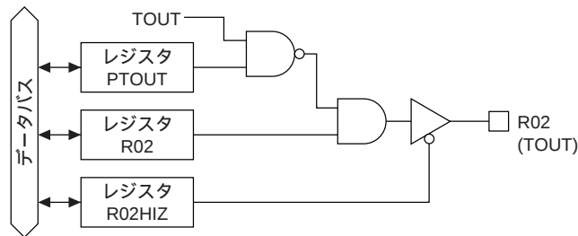
図4.11.8.1 R02の構成
