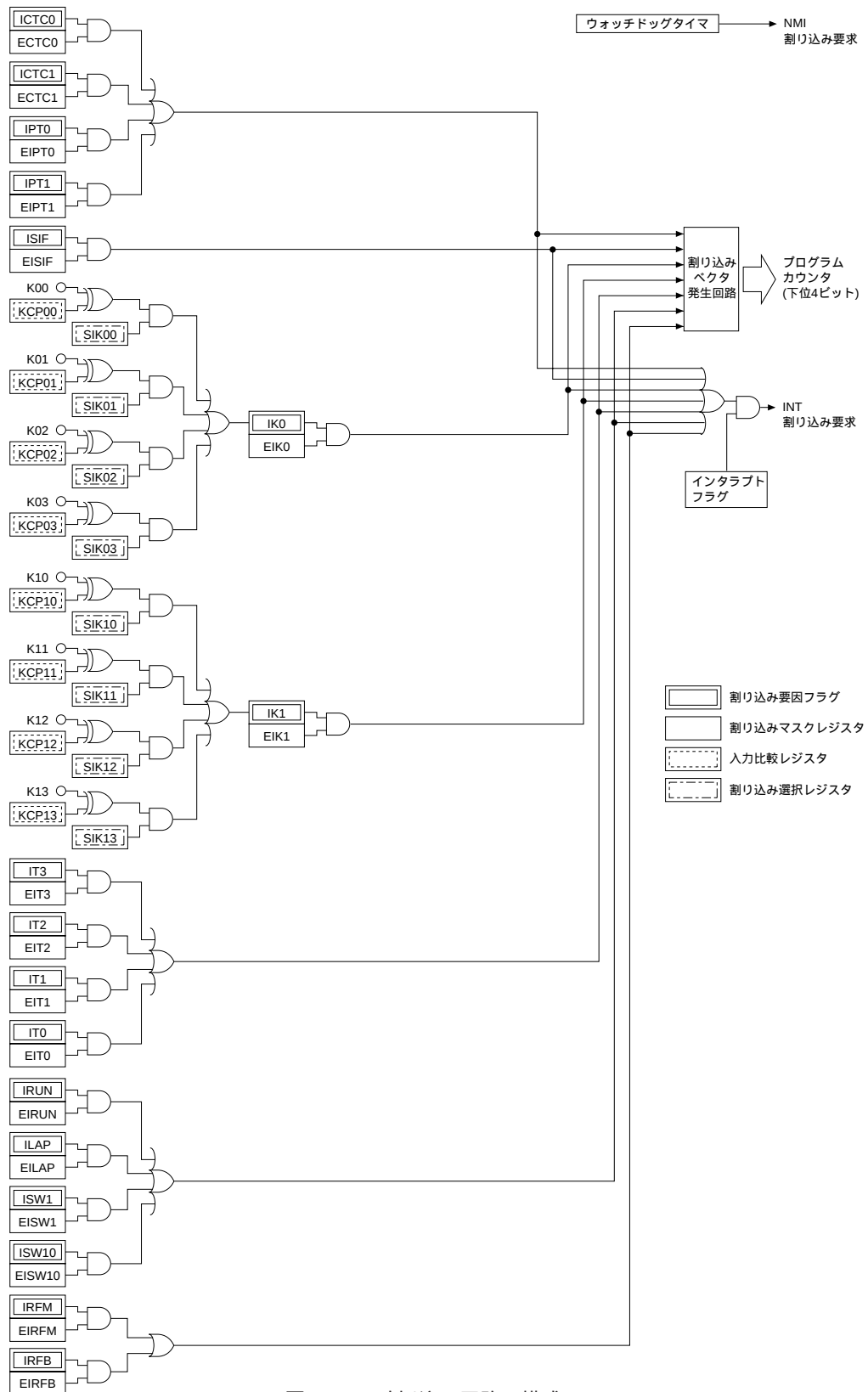
図4.16.1 割り込み回路の構成
