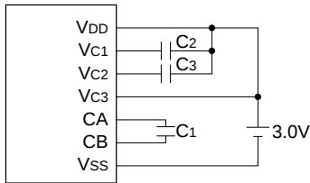
図2.1.5.1 LCD系定電圧回路を使用しない場合の外付け部品の構成
