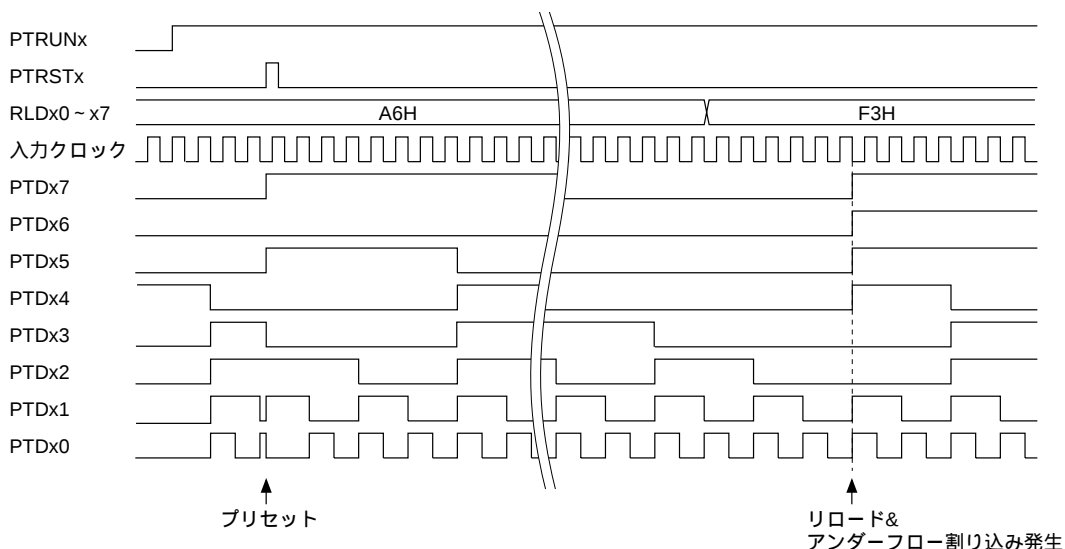
図4.11.2.1 カウンタの基本動作タイミング
