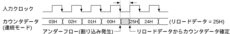
図4.11.11.2 プログラマブルタイマリロードタイミング
