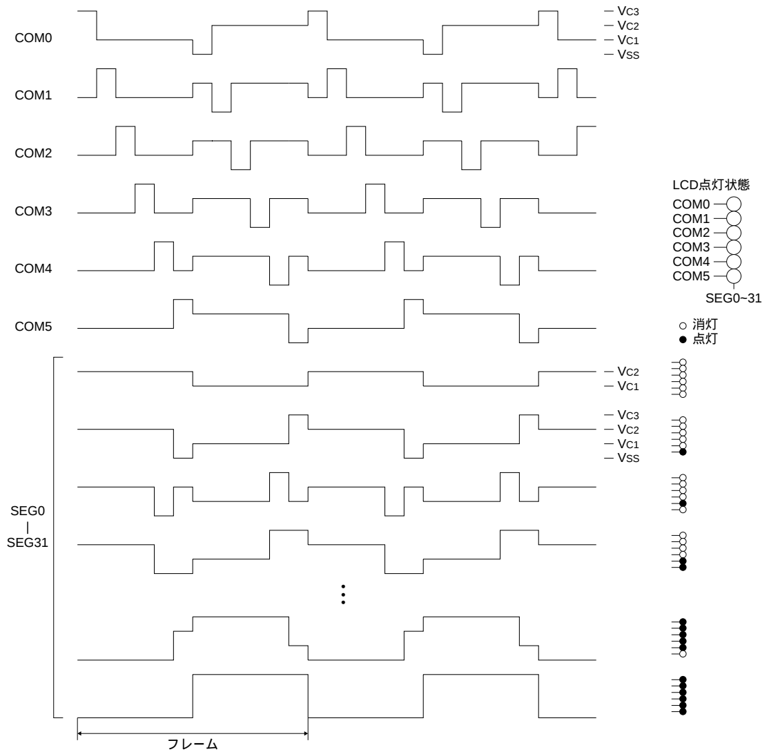
図4.8.3.1 1/6デューティLCD駆動波形
