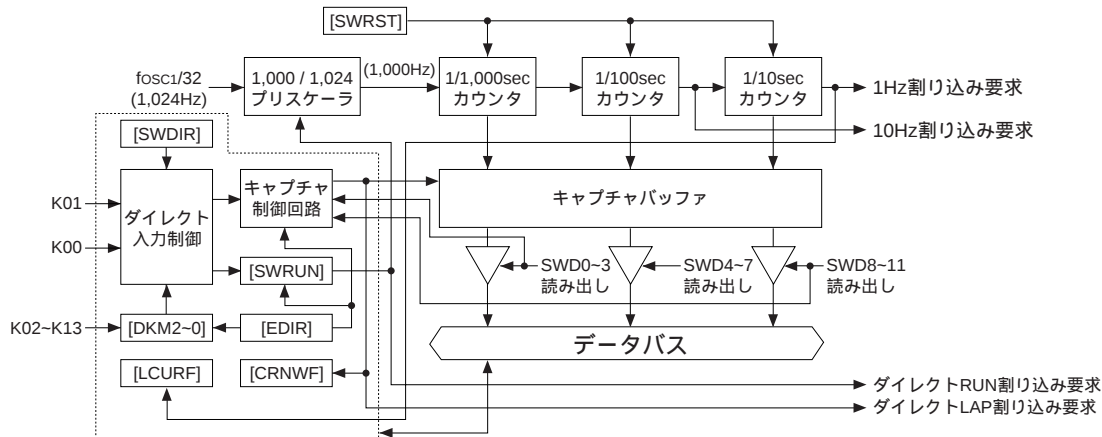
図4.10.1.1 ストップウォッチタイムのブロック図
