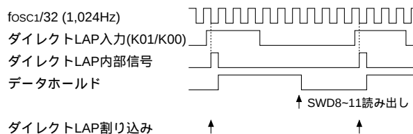
図4.10.5.2 ダイレクトLAP入力時の動作タイミング
