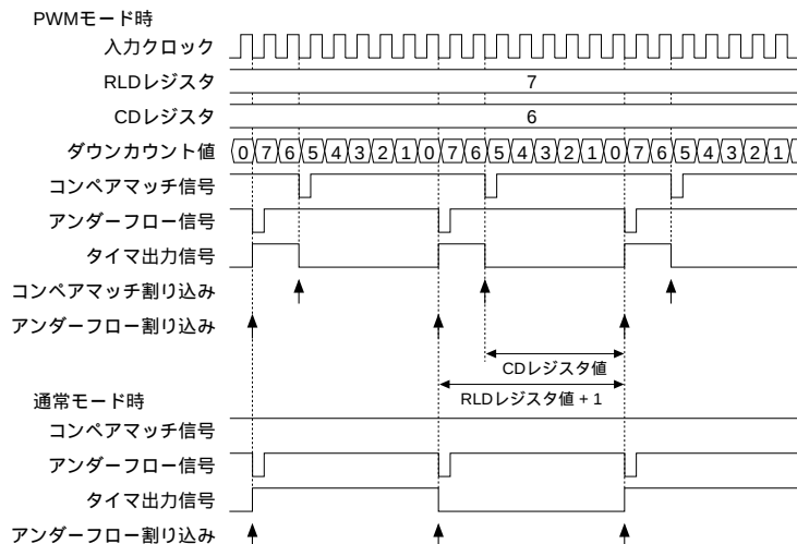
図4.11.5.1 PWM波形の生成
