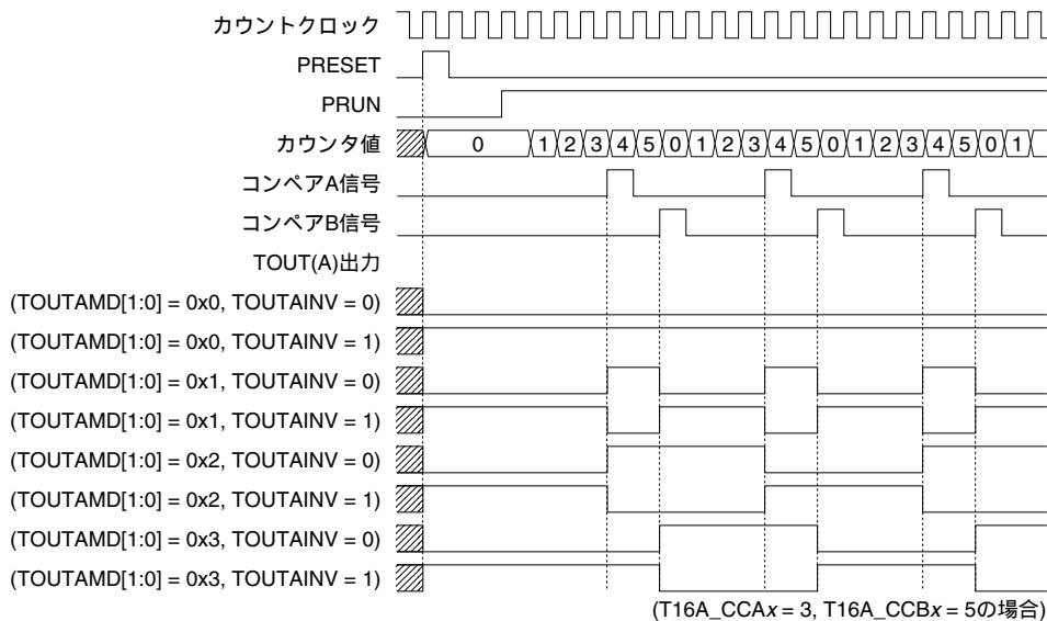
図12.6.2 TOU出力波形
