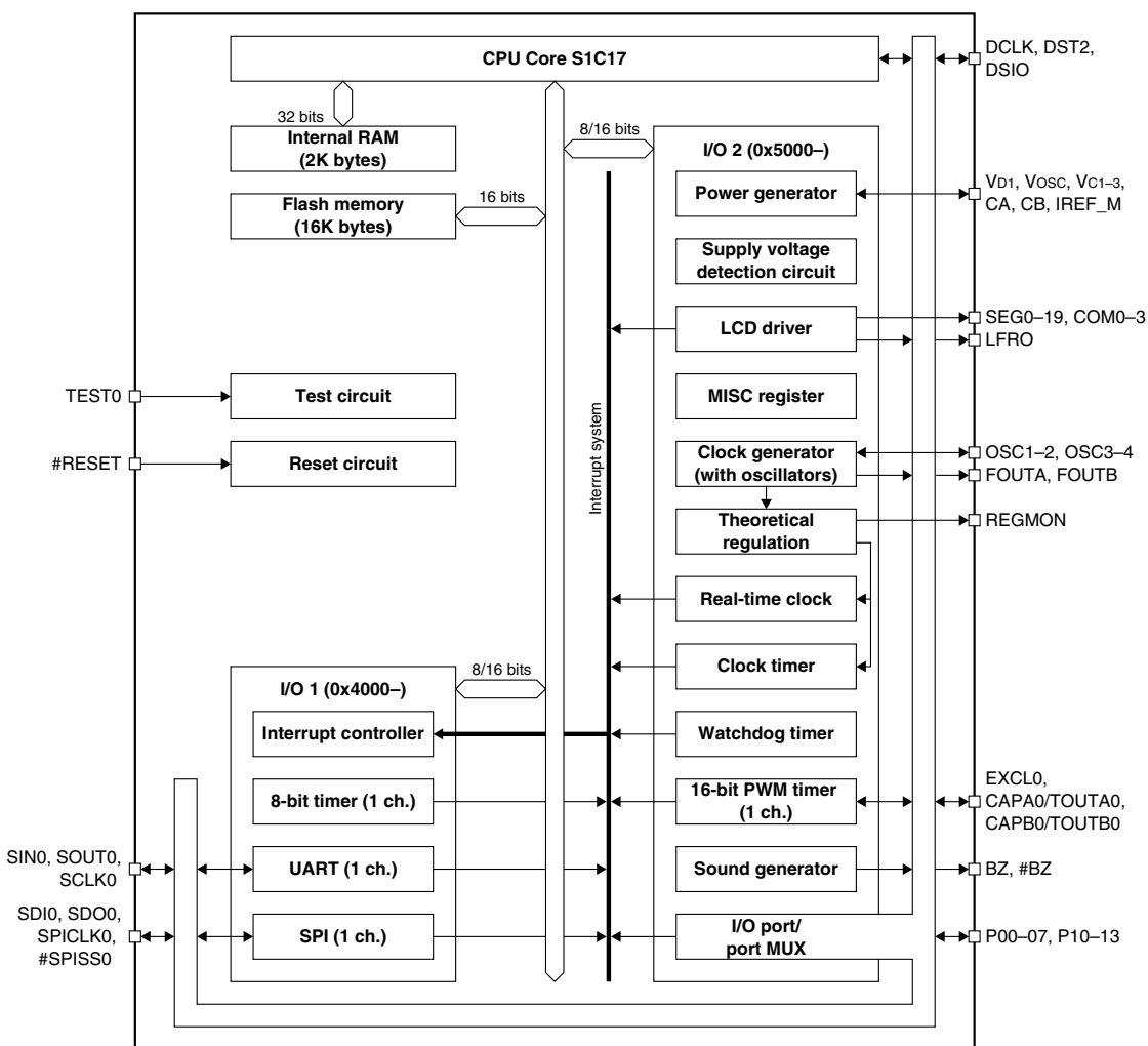
図1.2.1 S1C17651ブロック図
