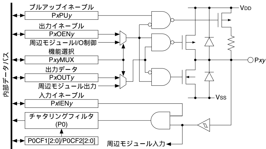
図10.1.1 入出力ポートの構成
