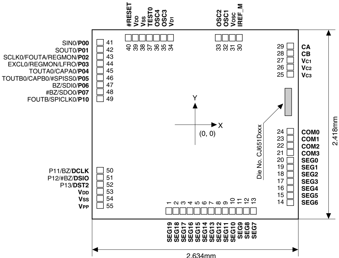
図1.3.1.2 S1C17651パッド配置図
