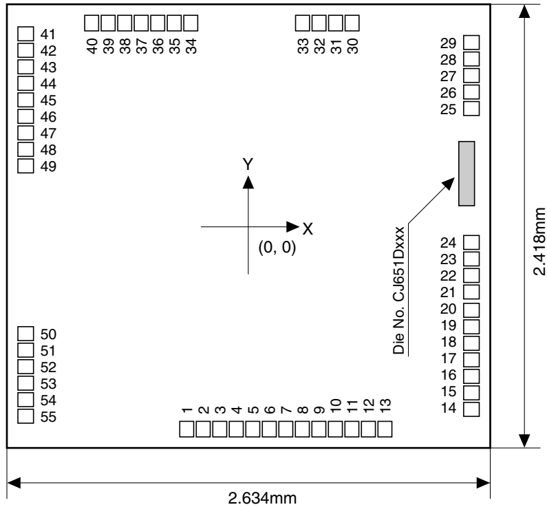
図24.2.1.1 S1C17651パッド配置図
