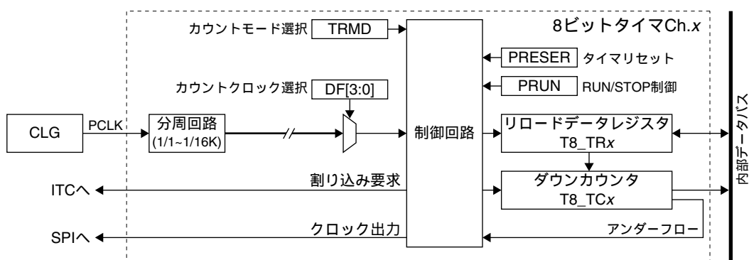
図11.1.1 T8モジュールの構成
