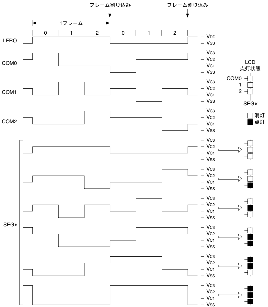
図17.4.2.2 1/3デューティ駆動波形
