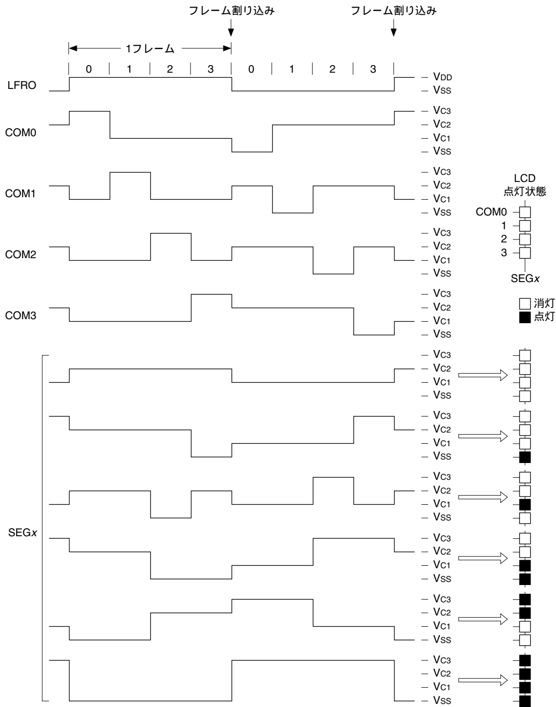
図17.4.2.1 1/4デューティ駆動波形
