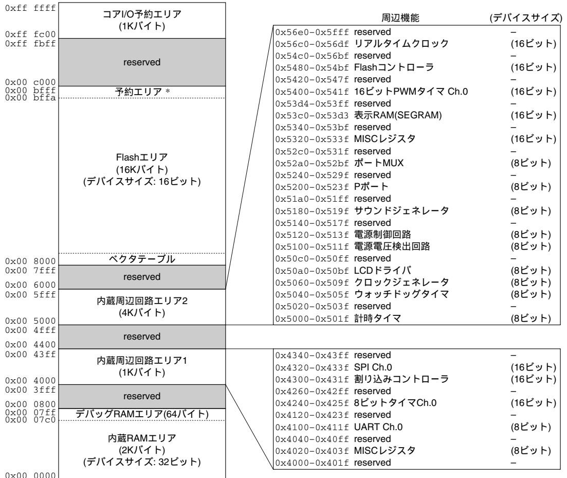
図3.1 S1C17651メモリマップ
