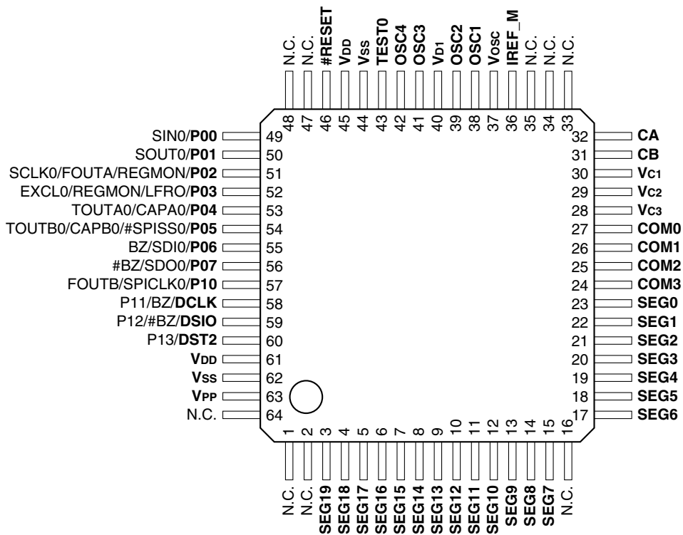
图1.3.1.1 S1C17651端子配置图(TQFP13-64pin)
