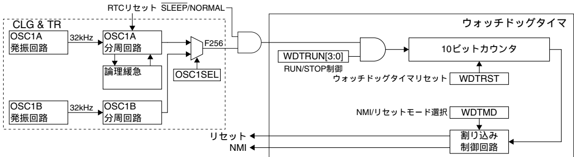
図14.1.1 WDTの構成
