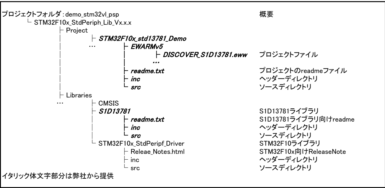
図 2-1 プロジェクトフォルダの構成(STM32)
