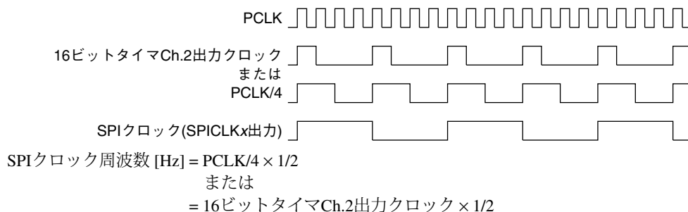
図16.3.1 マスタモードのSPIクロック
