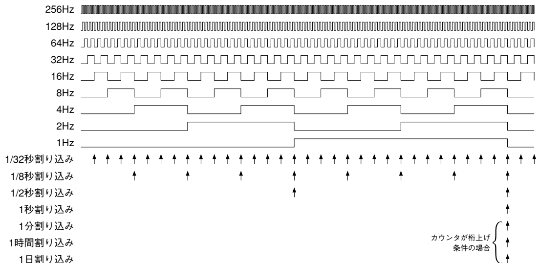
図13.4.1 リアルタイムクロックの割り込みタイミングチャート
