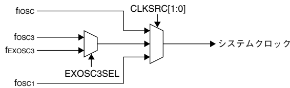
図7.4.1 システムクロックセレクタ
