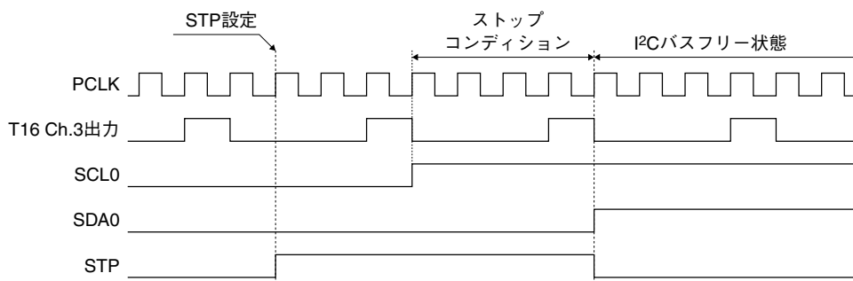
図17.5.9 ストップコンディション生成
