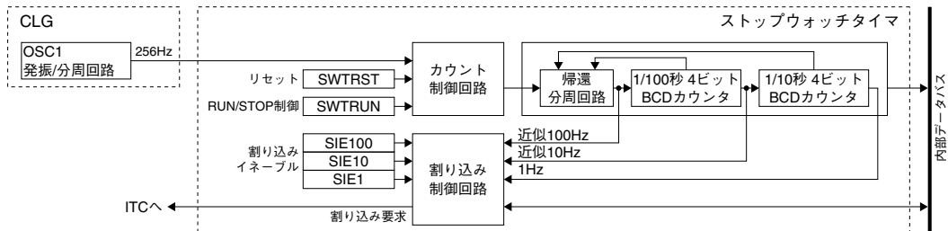
図12.1.1 SWTの構成
