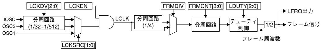
図21.4.1 LCDクロックシステム
