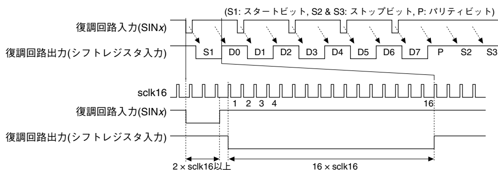
図15.8.2 受信信号波形
