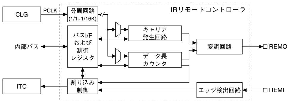
図19.1.1 REMCモジュールの構成
