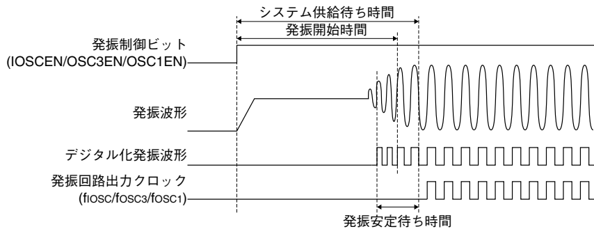
図7.3.1.2 発振開始時間と発振安定待ち時間
