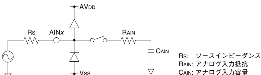
図22.3.5.1 アナログ入力等価回路
