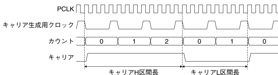
図19.3.1 キャリア信号の生成
