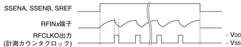
図23.4.3.1 CR発振クロック (RFCLK) 波形
