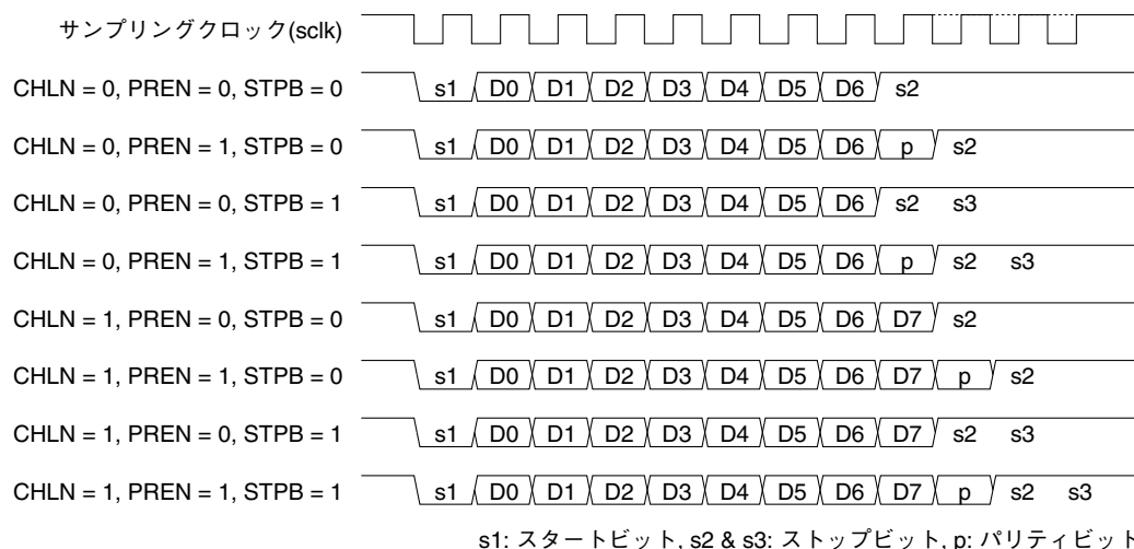
図15.4.1 転送データ形式
