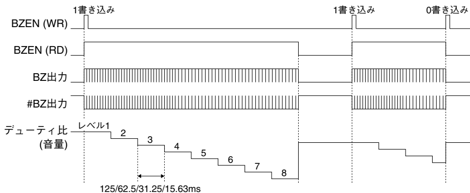
図20.5.4.1 エンベロープモードのブザー出力
