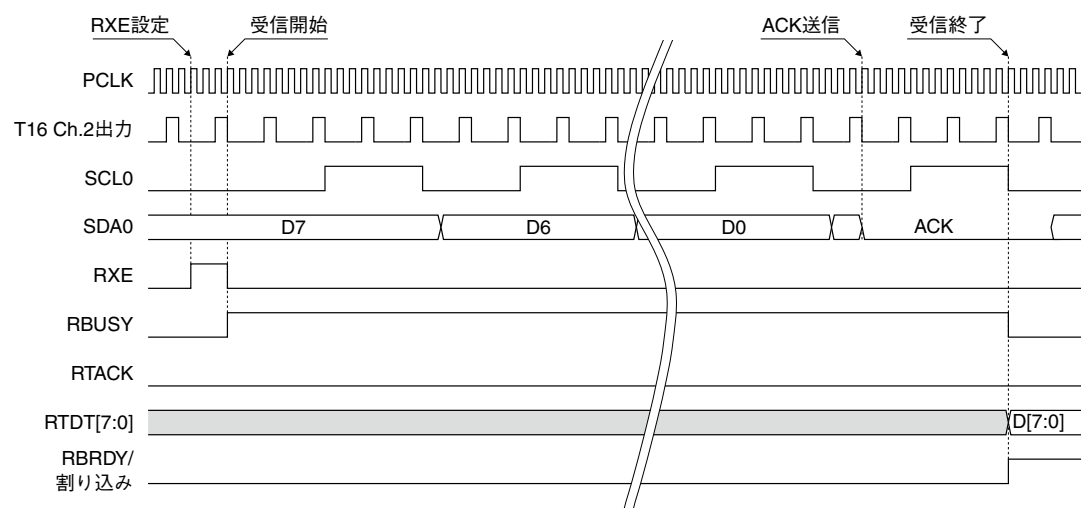
図17.5.8 データ受信
