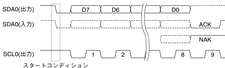
図17.5.3 ACKとNAK
