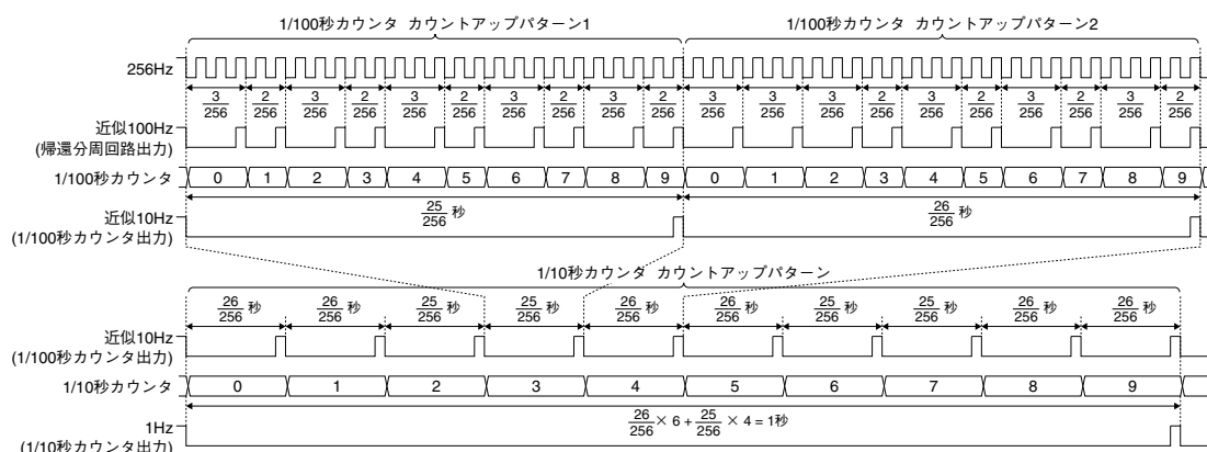
図12.3.1 SWTのカウントアップパターン
