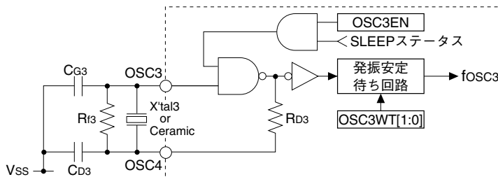
図7.3.2.1 OSC3発振回路
