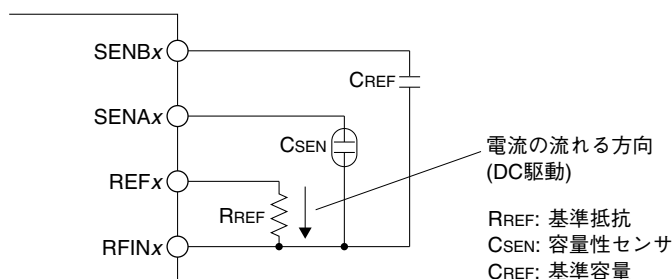
図23.4.1.3 容量性センサ測定用DC発振モードの接続例
