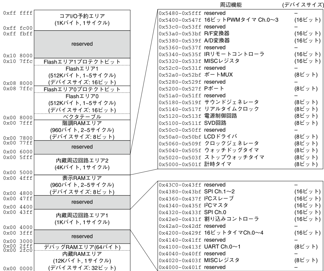
図3.1 S1C17706メモリマップ
