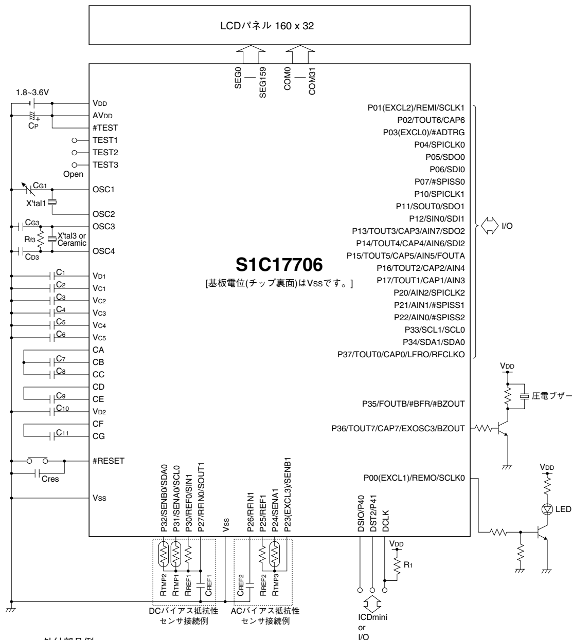
外付部品例
