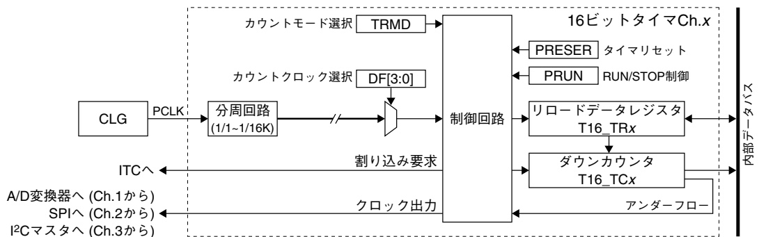
図9.1.1 T16モジュールの構成(1チャンネル)
