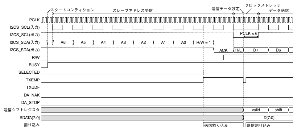
図18.5.5 I2CSタイミングチャート1(スタートコンディション→データ送信)
