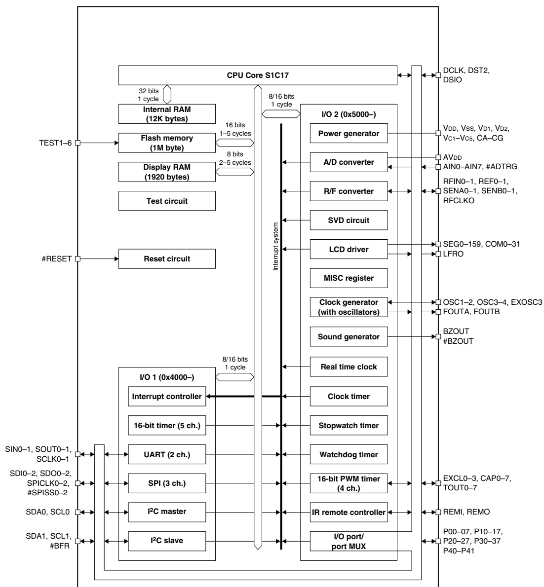
図1.2.1 ブロック図
