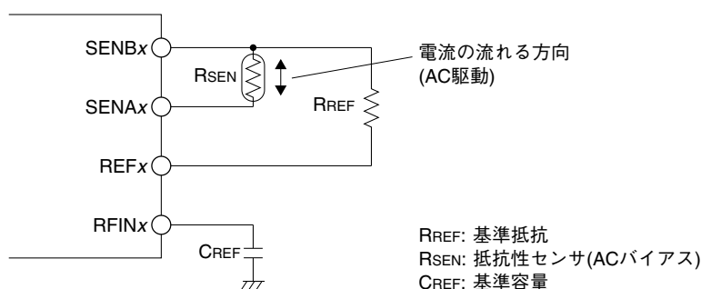
図23.4.1.2 抵抗性センサ測定用AC発振モードの接続例
