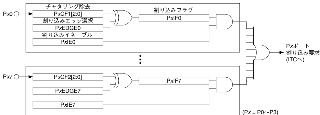
図8.7.1 ポート入力割り込み回路の構成
