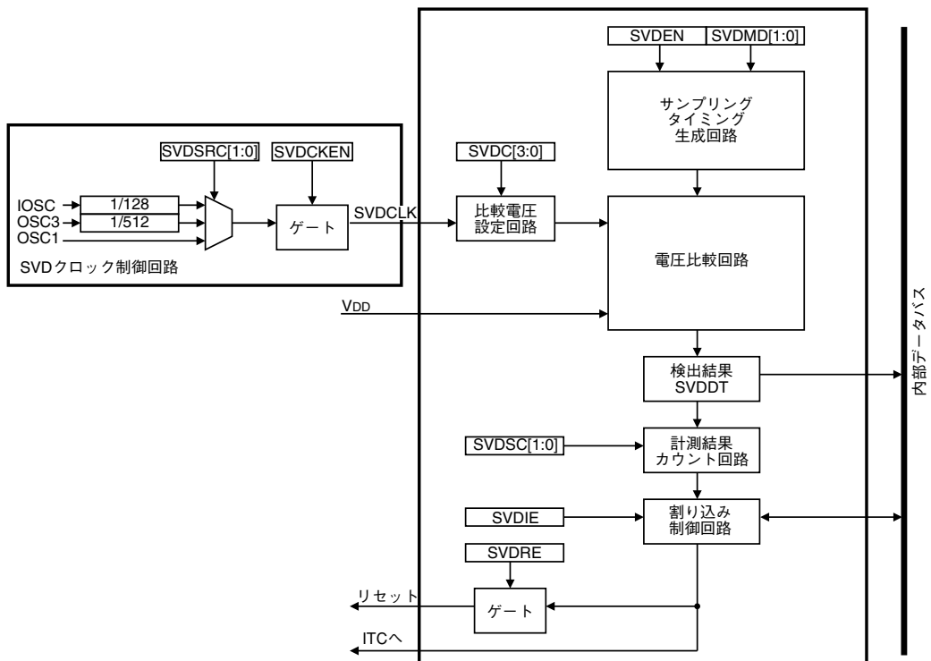
図24.1.1 SVD回路の構成
