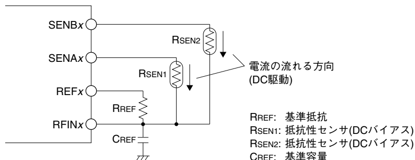
図23.4.1.1 抵抗性センサ測定用DC発振モードの接続例
