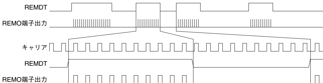
図19.5.1 データ送信
