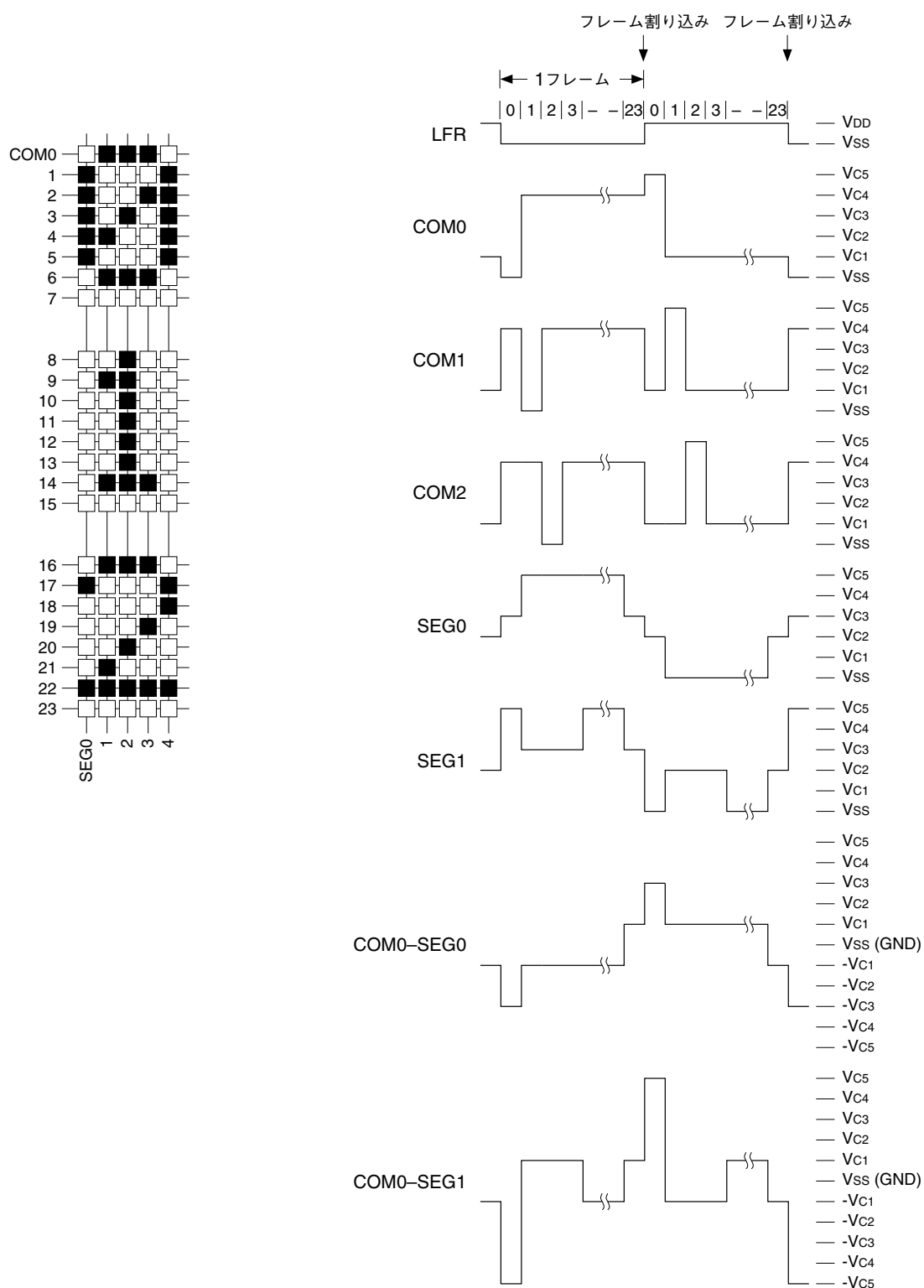
図21.5.2.2 1/24デューティの駆動波形
