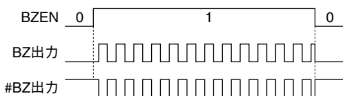
図20.5.2.1 ノーマルモードのブザー出力
