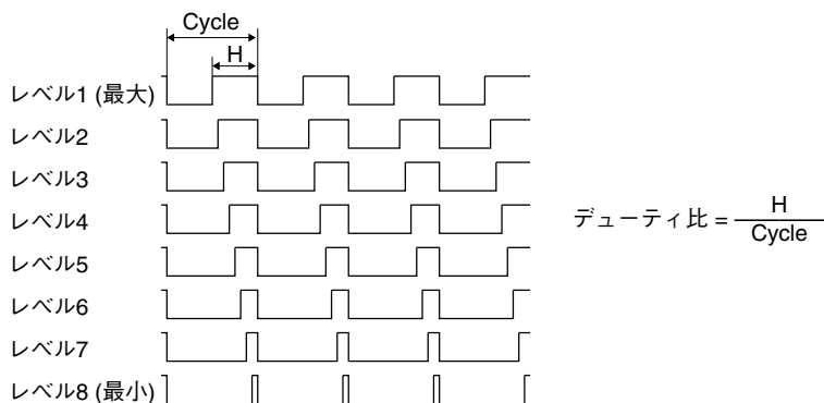
図20.4.2.1 ブザー信号波形のデューティ比
