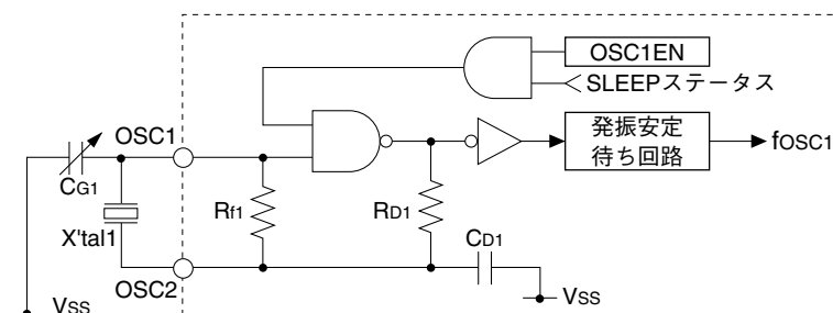
図7.3.3.1 OSC1発振回路
