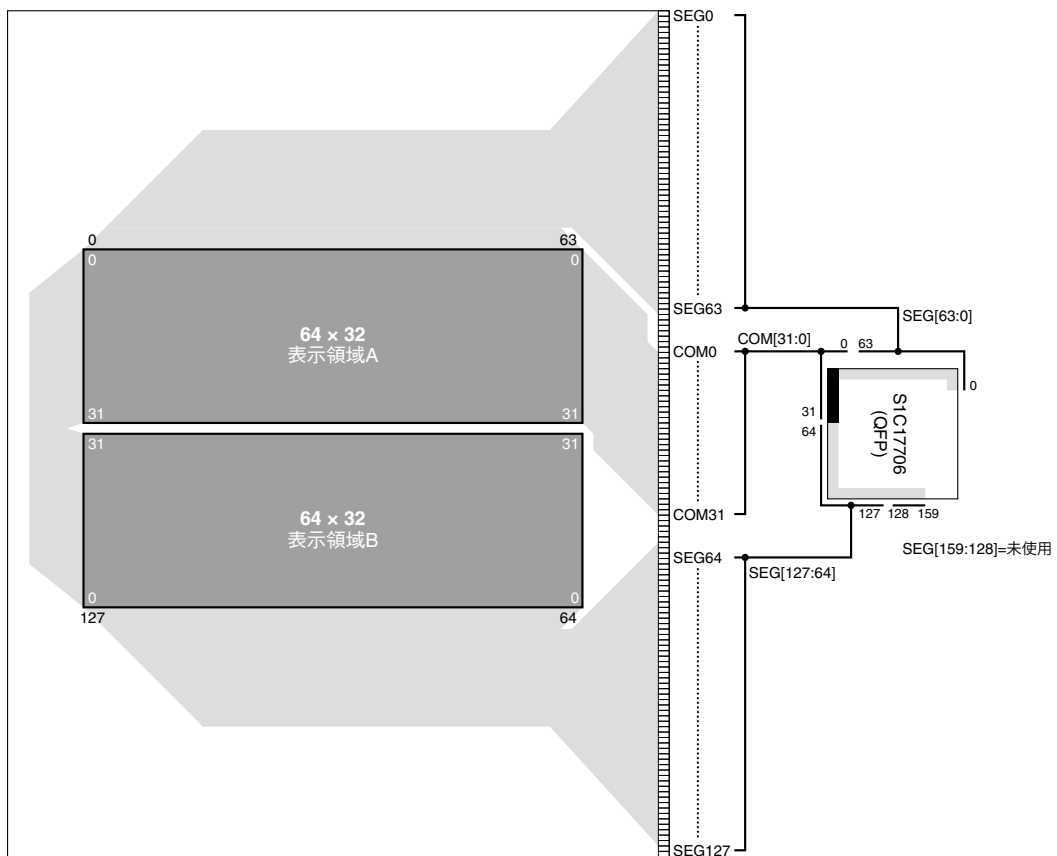
図21.5.3.1 擬似64COM/パネル接続例
