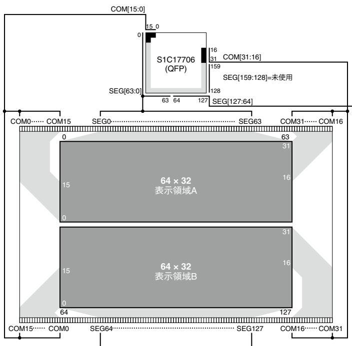
例1: COMPOS = 0, COMREV = 0, SEGREV = 1, LDUTY[2:0] = 0x2 (通常の1/32デューティ)
