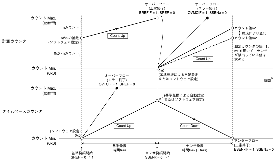
図23.6.2.1 基準発振/センサ発振によるカウンタの動作
