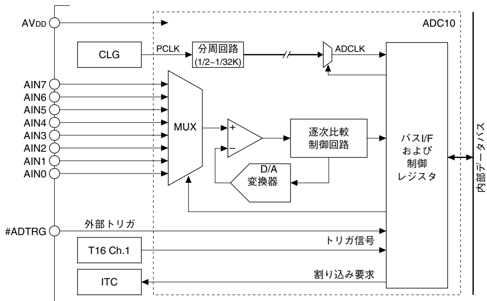
図22.1.1 A/D変換器の構成
