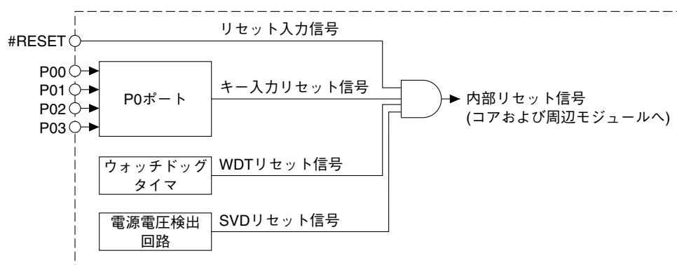
図5.1.1 イニシャルリセット回路の構成
