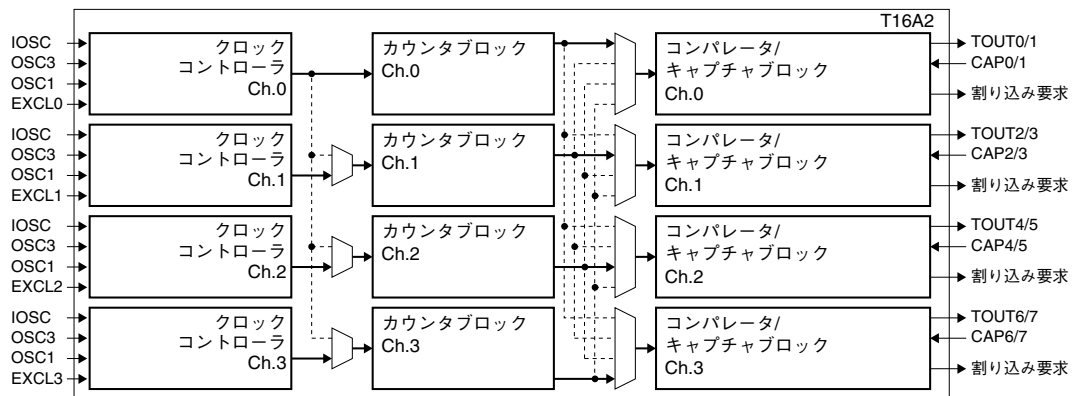
図10.4.3.1 ノーマルチャネルモードのタイマ構成 (2系統コンパレータ/キャプチャブロック × 4チャネル)
