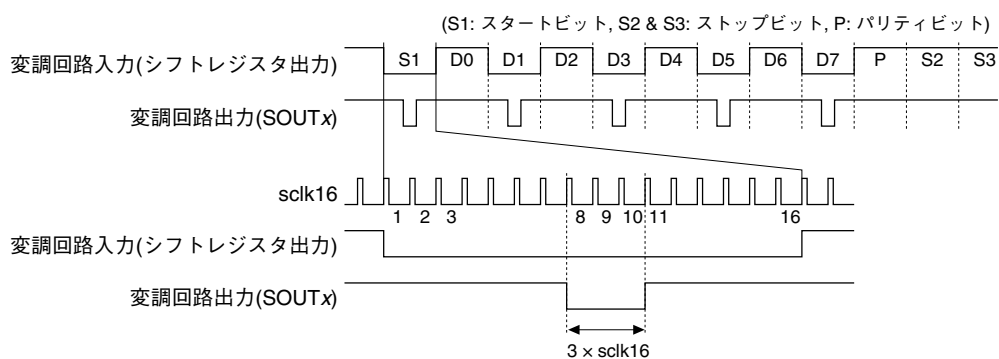
図15.8.1 送信信号波形
