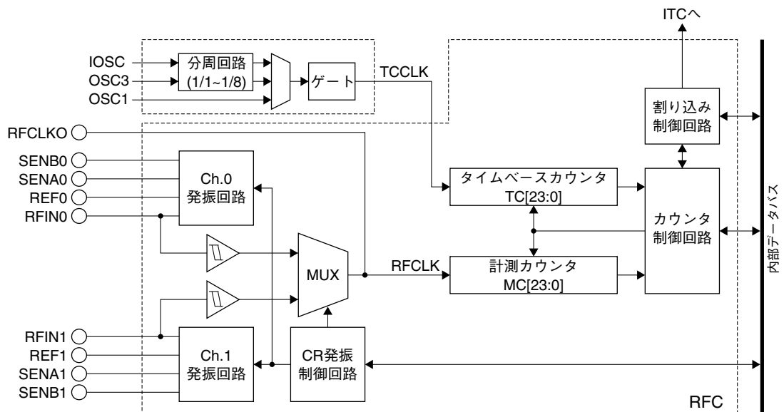
図23.1.1 R/F変換器の構成
