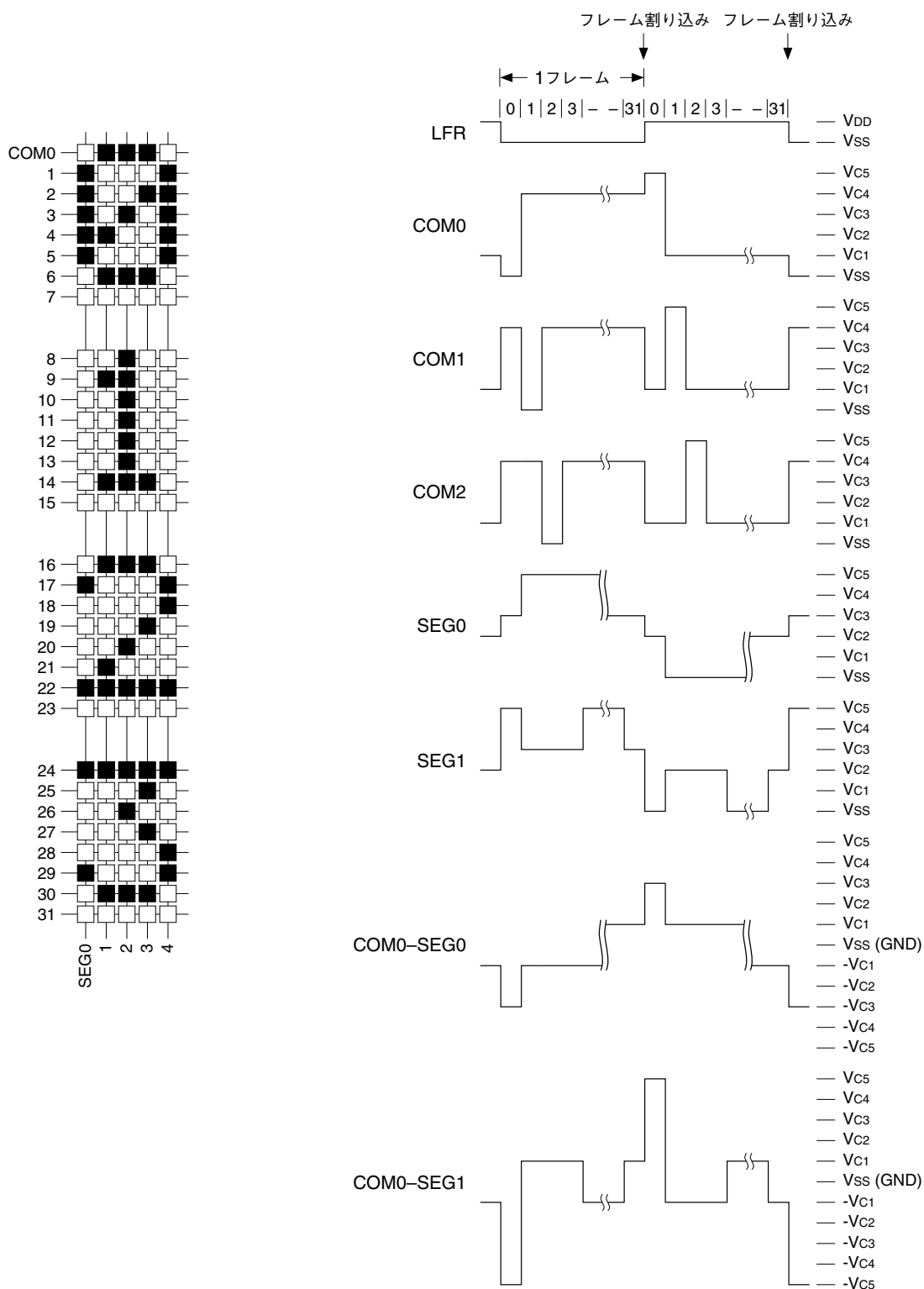
図21.5.2.1 1/32デューティの駆動波形
