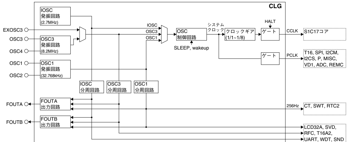
図B.1.1 クロックシステム
