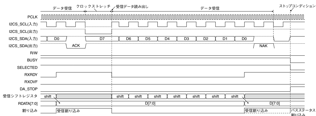
図18.5.8 I2CSタイミングチャート4(データ受信→ストップコンディション)
