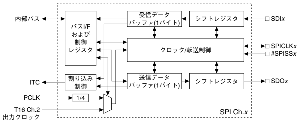
図16.1.1 SPIモジュールの構成(1チャネル)
