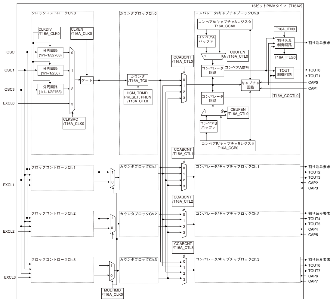
図10.1.1 T16A2の構成
