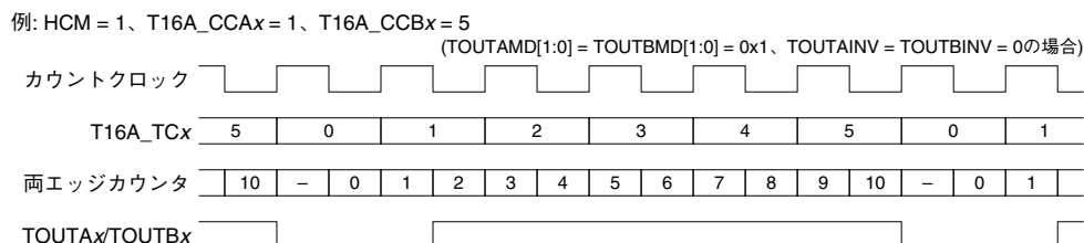
図10.6.4 ハーフクロックモードのPWM波形出力タイミング
