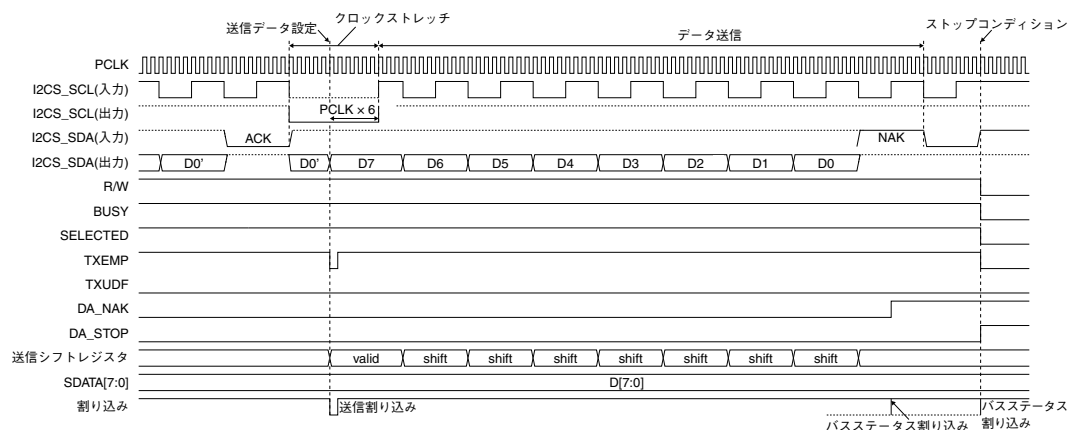
図18.5.6 I2CSタイミングチャート2(データ送信→ストップコンディション)
