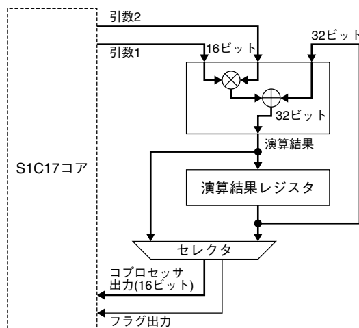
図26.5.2 積和演算モード時のデータ経路
