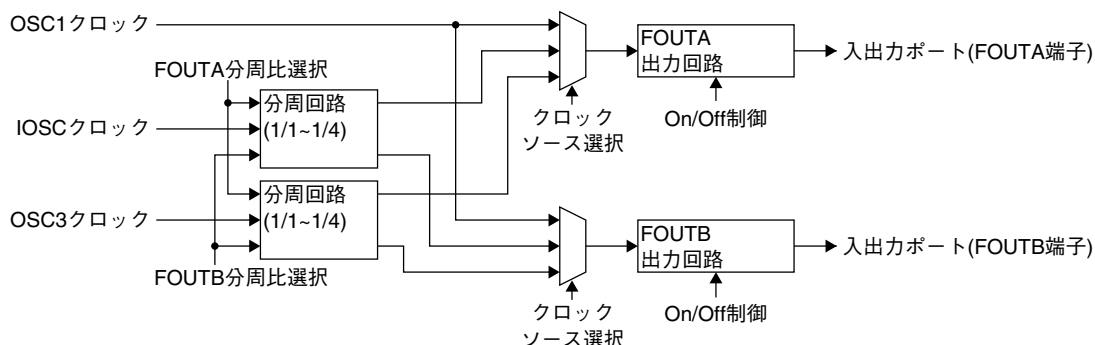
図7.7.1 クロック出力回路
