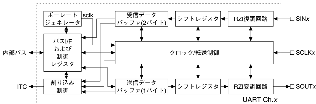
図15.1.1 UARTの構成
