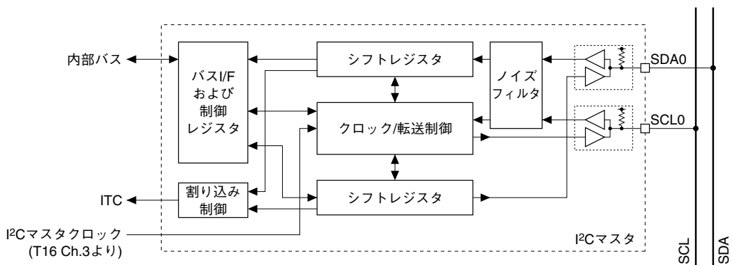
図17.1.1 I2CMモジュールの構成
