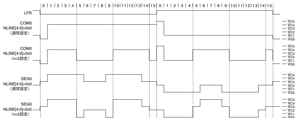
図21.5.5.1 1/16デューティの通常時とn=5設定時の駆動波形
