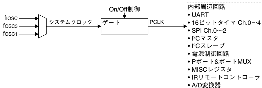
図7.6.1 周辺モジュールクロック制御回路
