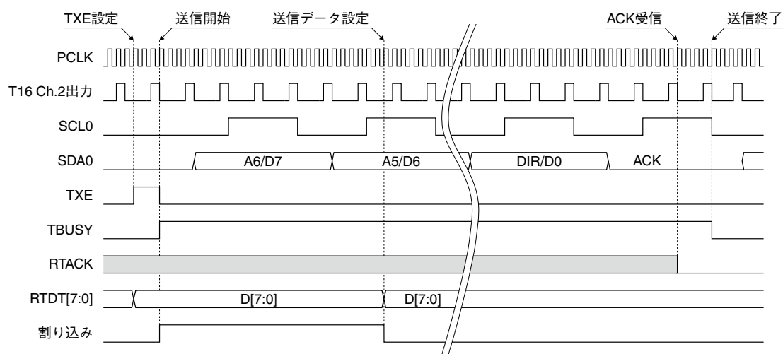
図17.5.7 スレーブアドレス送信 / データ送信
