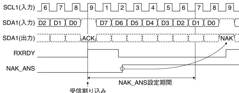
図18.5.3 NAK_ANSの設定とNAK応答タイミング
