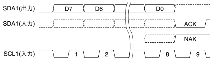
図18.5.2 ACKとNAK
