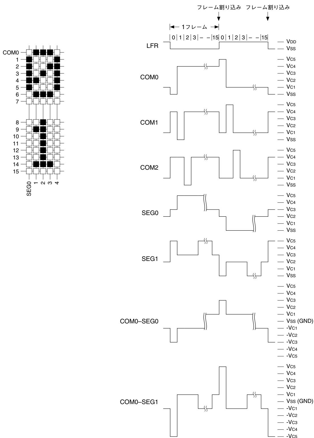
図21.5.2.3 1/16デューティの駆動波形
