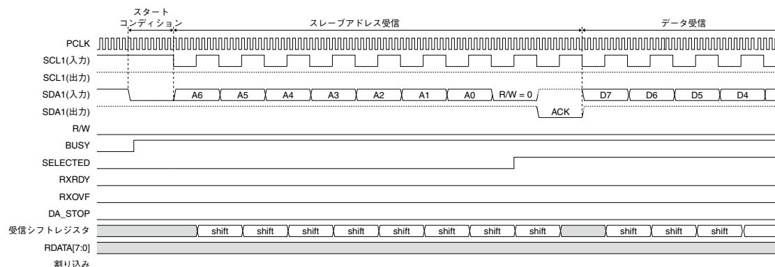
図18.5.7 I2CSタイミングチャート3(スタートコンディション→データ受信)
