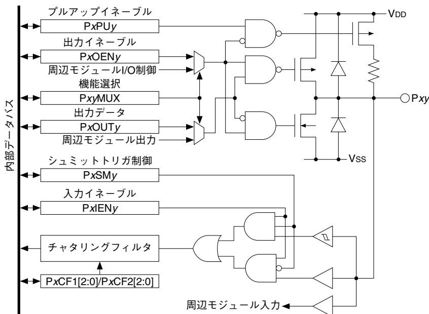
図8.1.1 入出力ポートの構成
