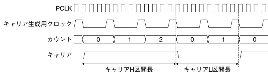
図19.7.1 キャリア信号の生成
