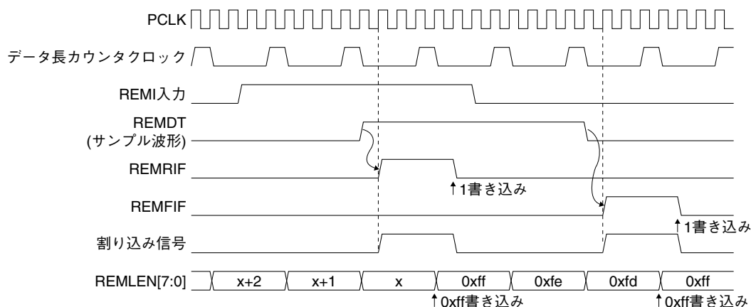
図19.5.3 データ受信
