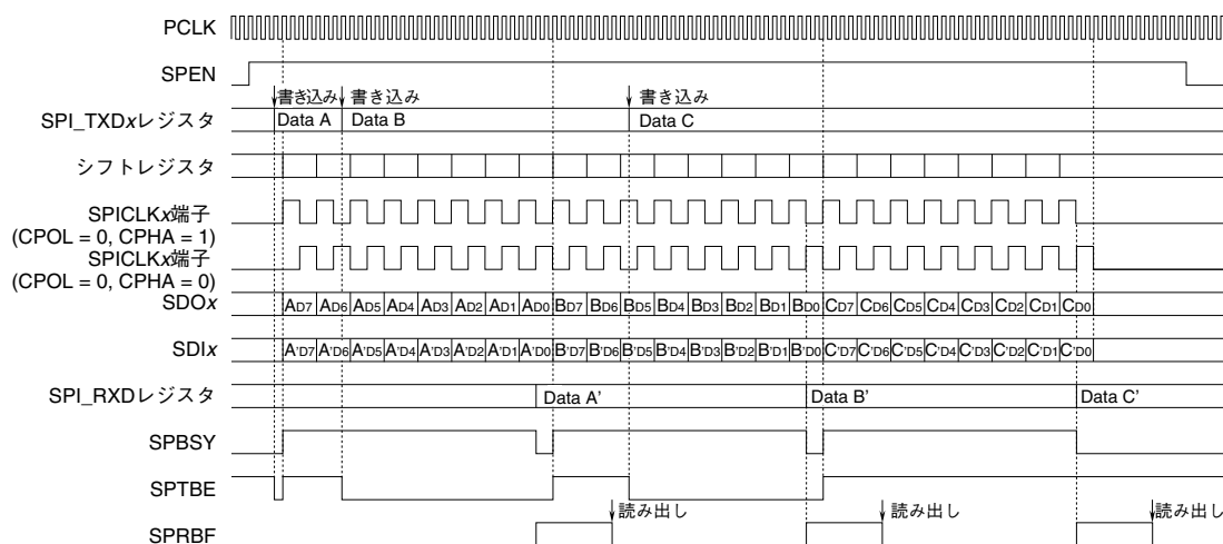
図16.5.1 データ送受信タイミングチャート (MSB先頭)
