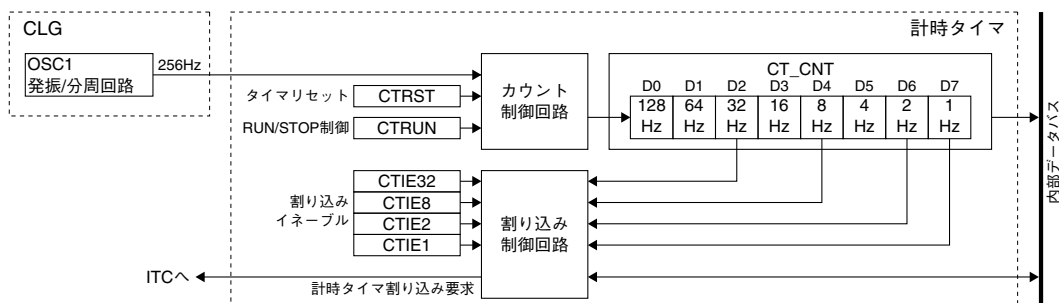
図11.1.1 CTの構成
