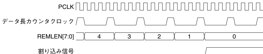
図19.5.2 アンダーフロー割り込み発生タイミング
