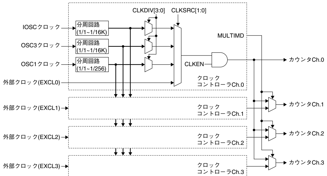
図10.3.1 クロックコントローラ
