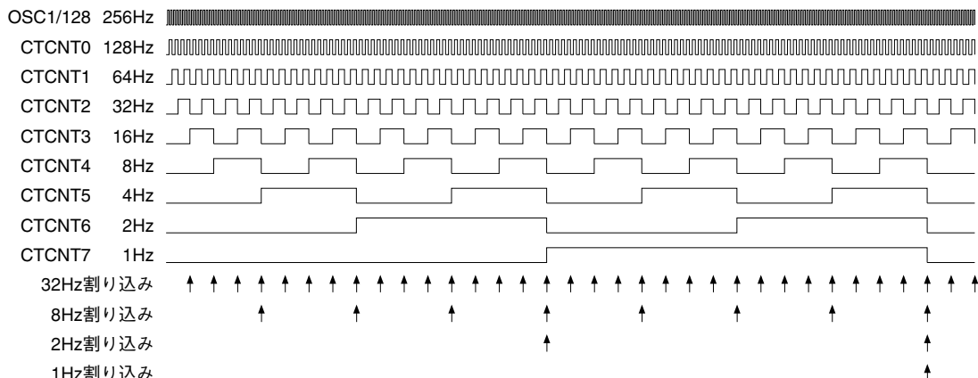
図11.4.1 計時タイマのタイミングチャート
