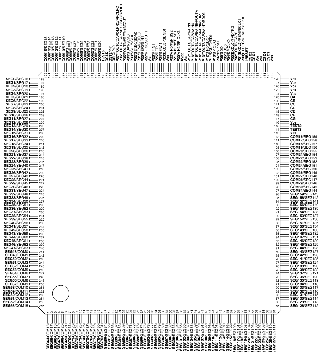
図1.3.1.1 端子配置図 (QFP22-256pin)
