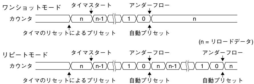
図9.4.1 プリセットタイミング
