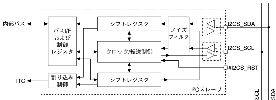
図18.1.1 I2CSモジュールの構成
