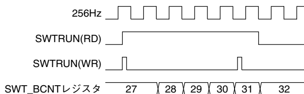
図12.5.2 Run/Stop制御のタイミングチャート
