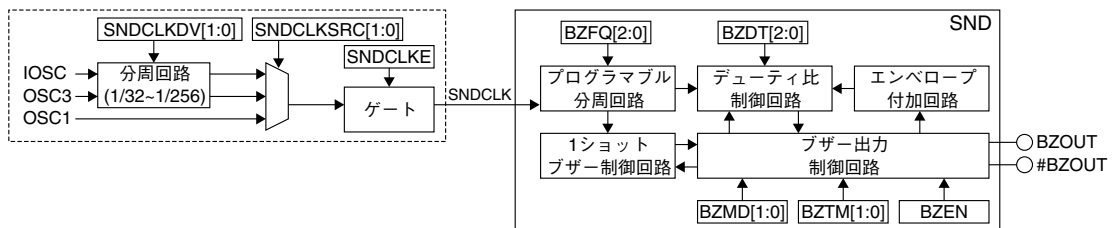
図20.1.1 SNDモジュールの構成
