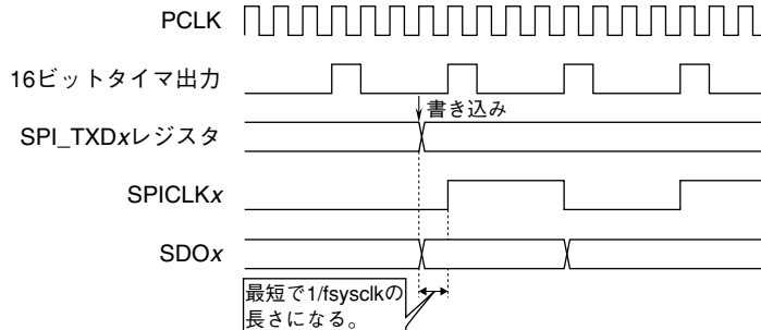
図16.4.2 CPHA = 0 時のSDOxおよびSPICLKxの変化タイミング
