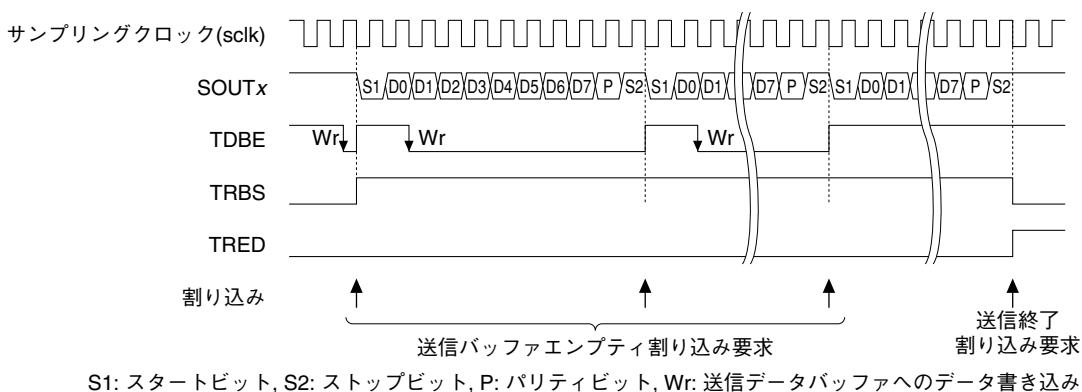
図15.5.1 データ送信タイミングチャート
