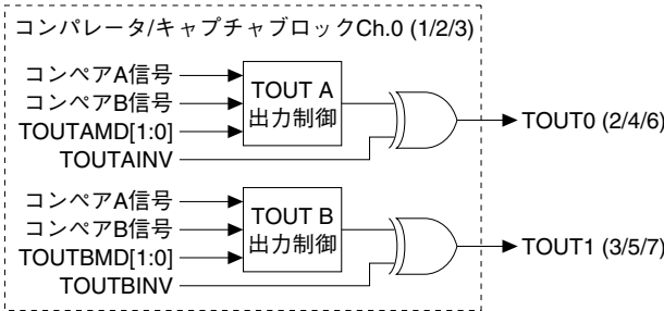
図10.6.1 TOUT出力回路
