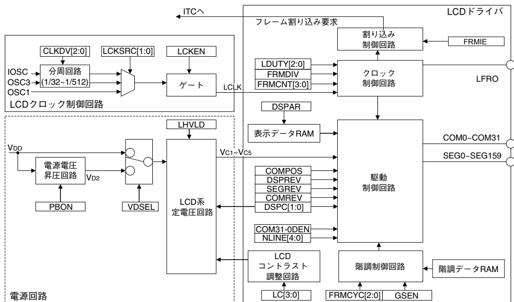
図21.1.1 LCDドライバと駆動電源の構成
