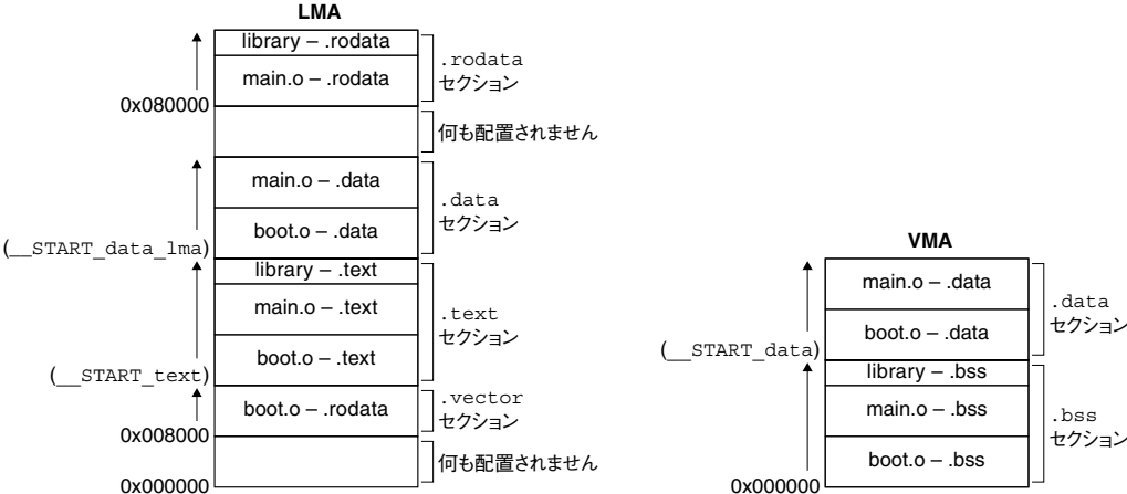
図5.7.6.5 セクション配置例2
