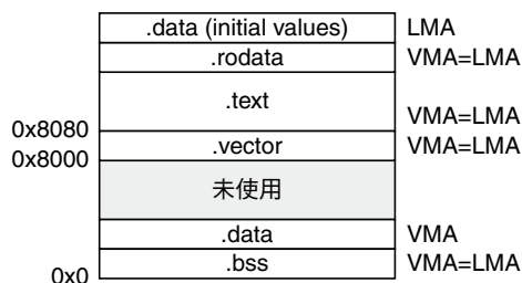
図9.4.1.1 デフォルトリンクスクリプトによるメモリマップ
