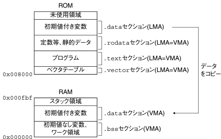
図5.7.6.2 メモリ構成例1
