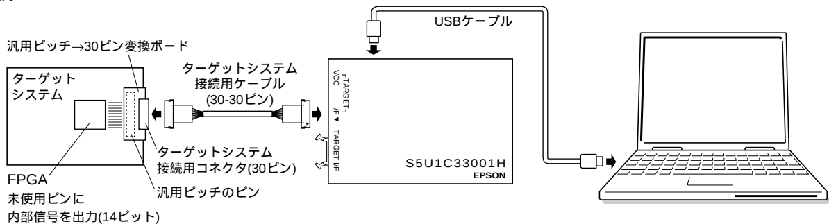
図18 ユーザロジック信号トレース用接続例
