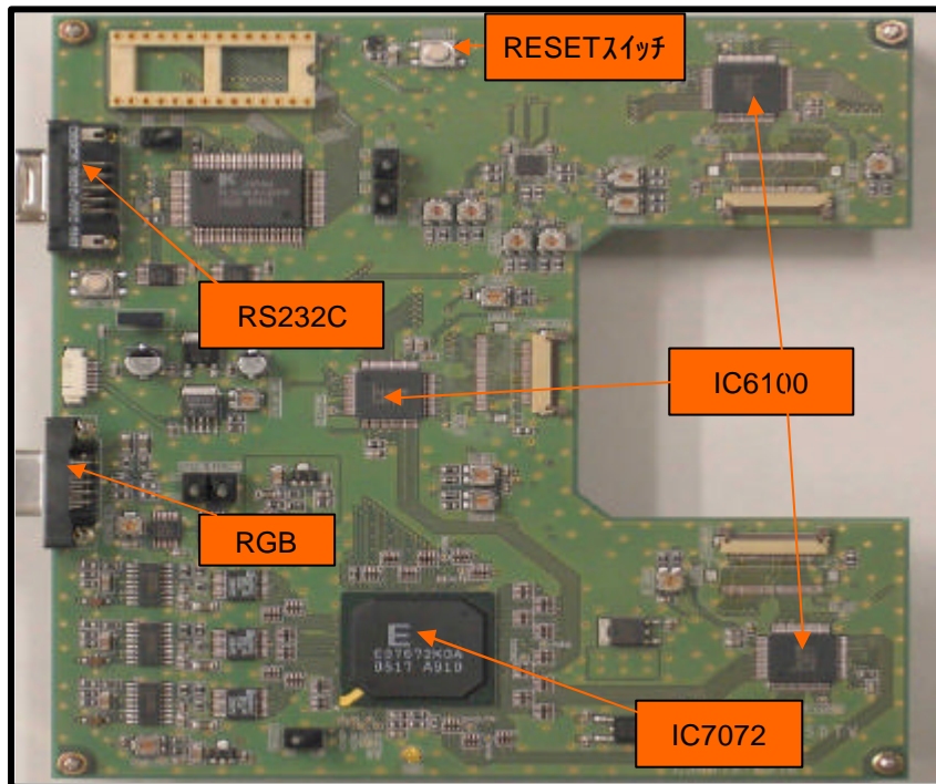
外形図 (外形寸法 :W150mm * H180mm)
