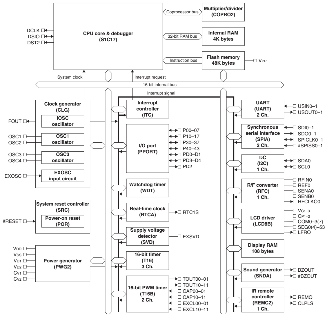
図1.2.1 S1C17W14ブロック図
