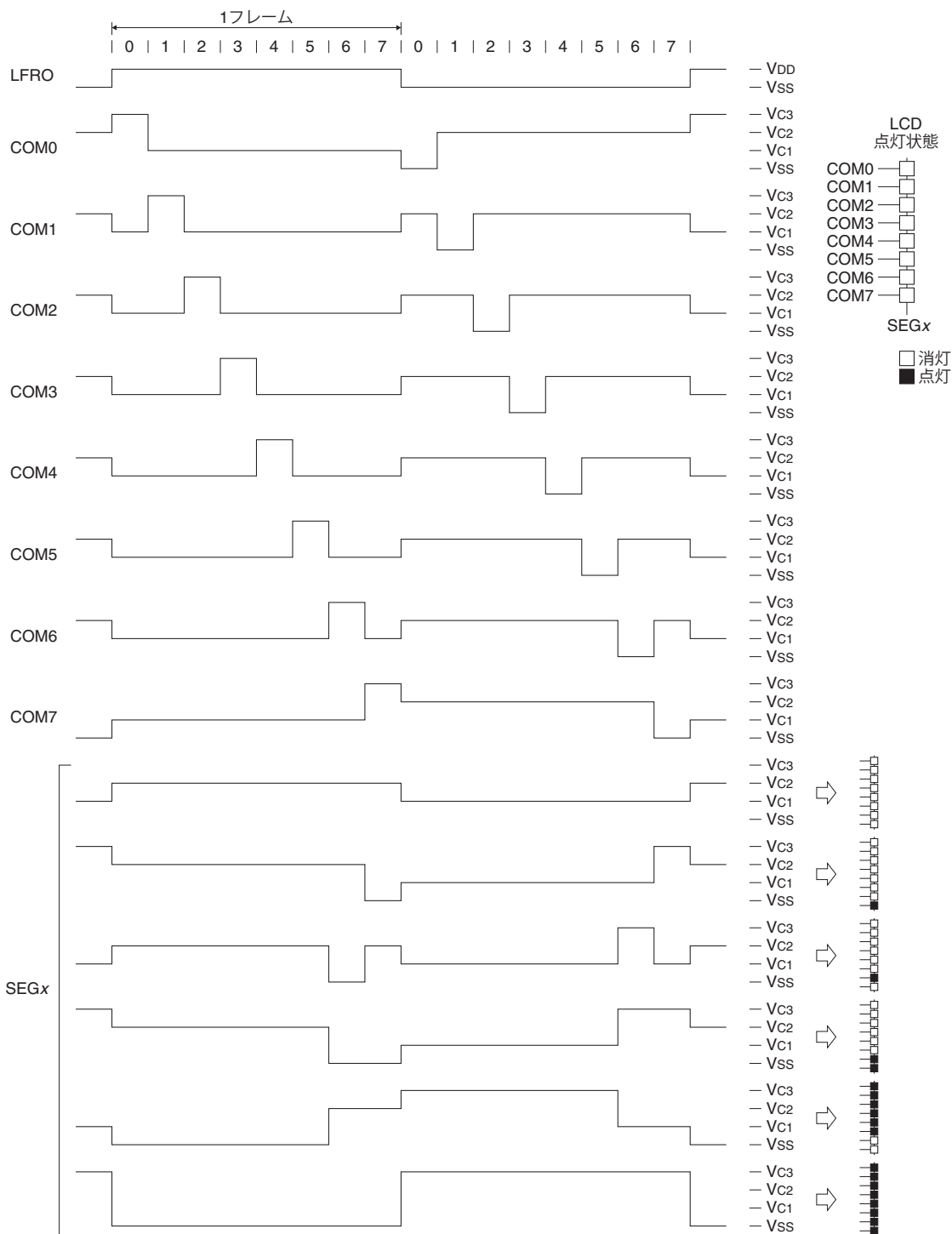
図18.5.5.1 1/8デューティの駆動波形(1/3バイアス)
