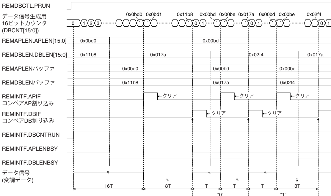
図17.4.4.1 連続送信例
