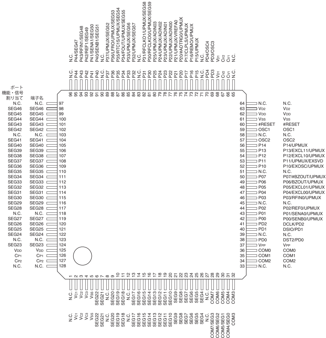
図1.3.1.2 S1C17W16端子配置図(TQFP15-128PIN)
