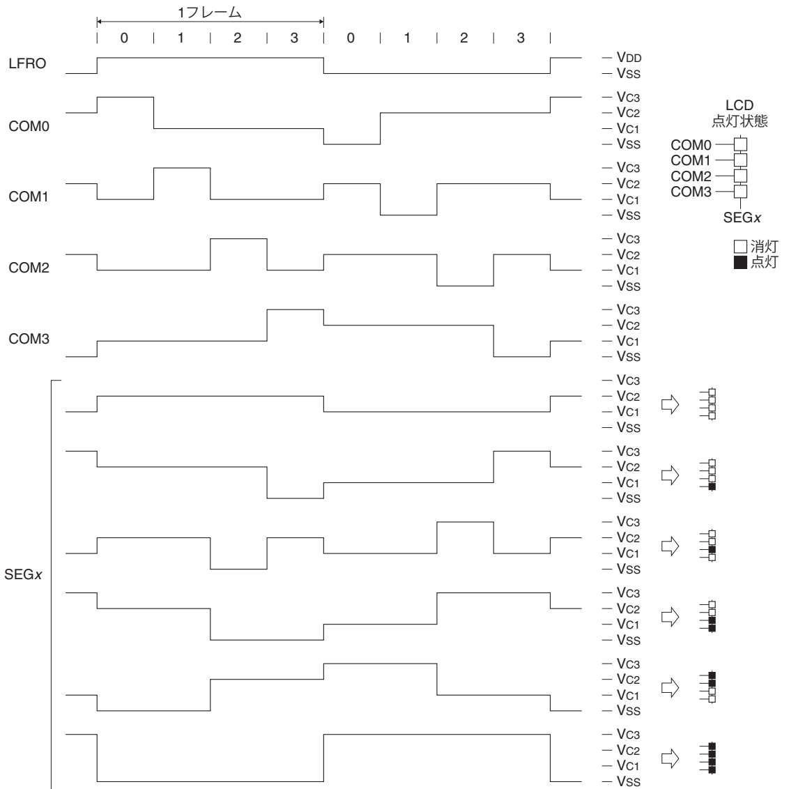
図18.5.5.2 1/4デューティの駆動波形(1/3バイアス)
