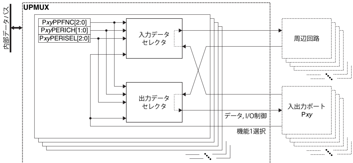
図7.1.1 UPMUXの構成
