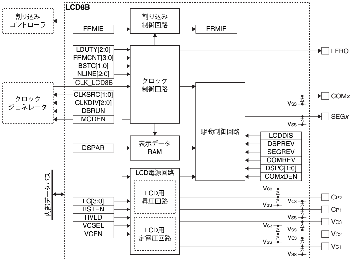
図18.1.1 LCD8Bの構成
