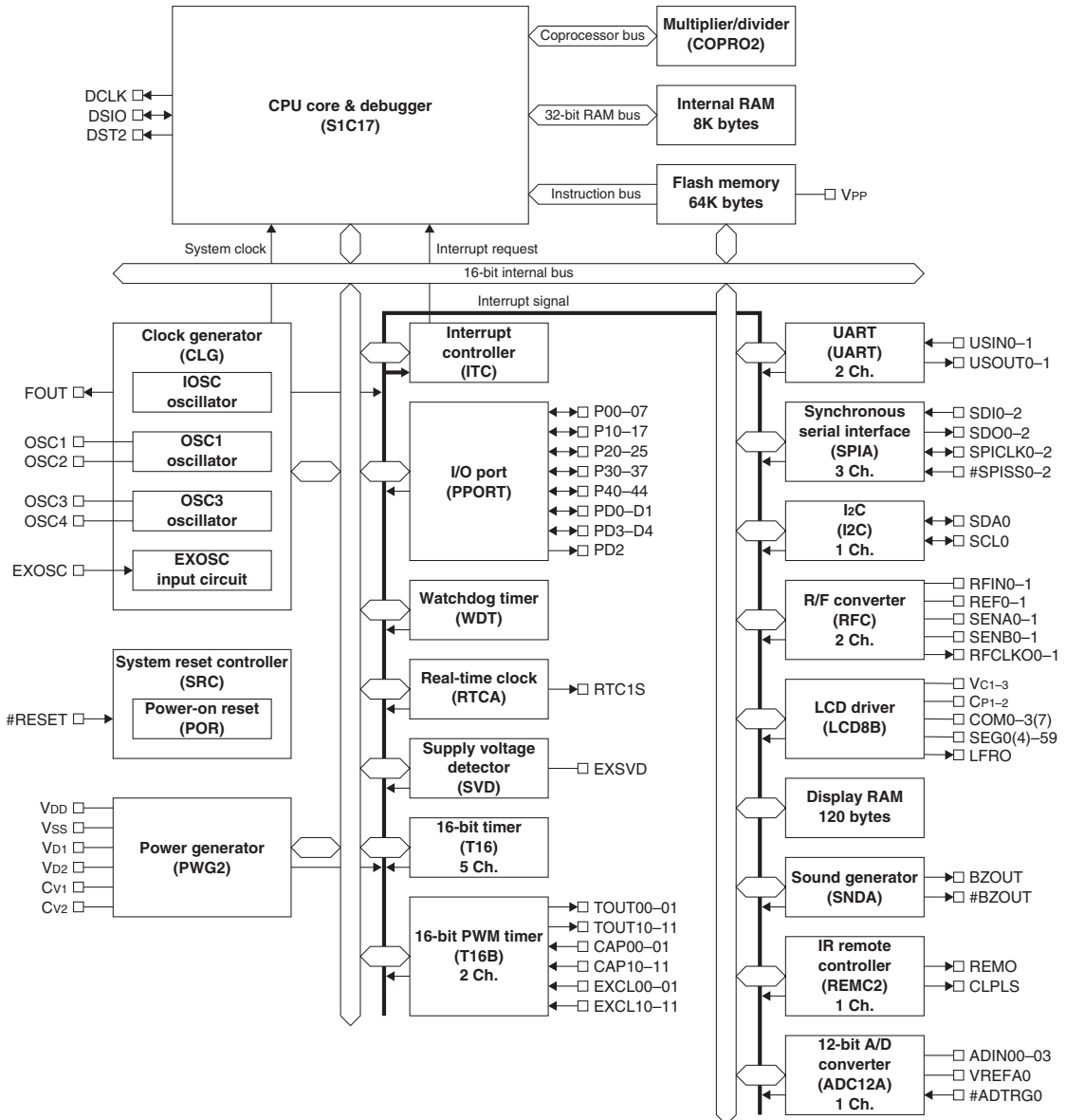
図1.2.2 S1C17W16ブロック図
