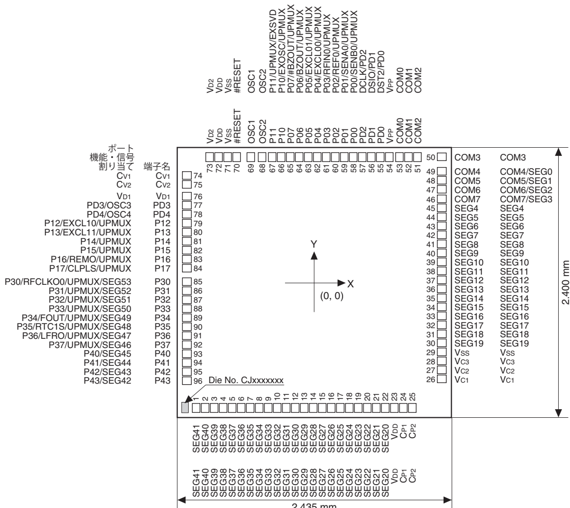
図1.3.2.1 S1C17W14パッド配置図(チップ)
