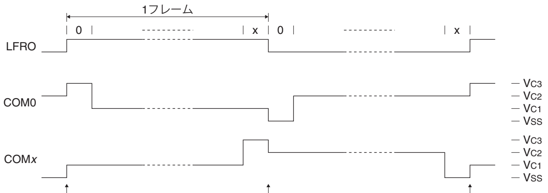
図18.7.1 フレーム割り込みタイミング(1/xデューティ、1/3バイアス)
