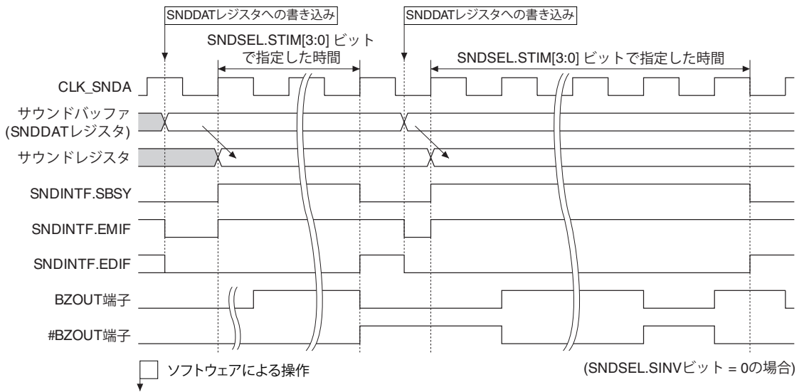
図16.4.3.1 ワンショットブザーモードのブザー出力タイミング
