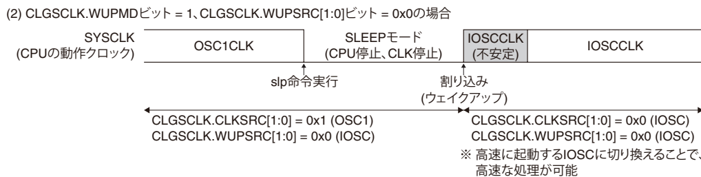
図2.3.4.4 SLEEP解除時のクロック制御例
