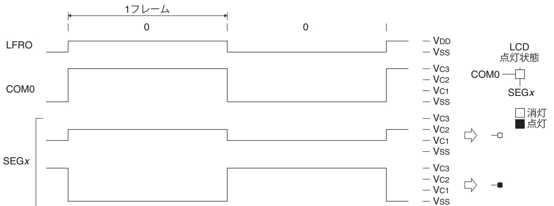
図18.5.5.3 スタティック駆動波形(1/3バイアス)
