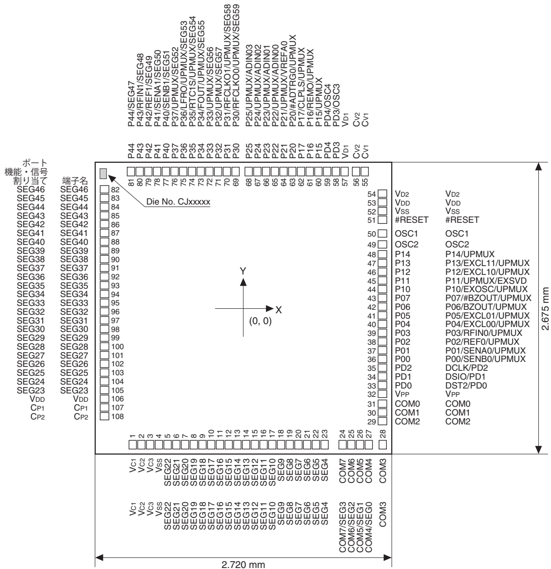
図1.3.2.2 S1C17W16/パッド配置図(チップ)
