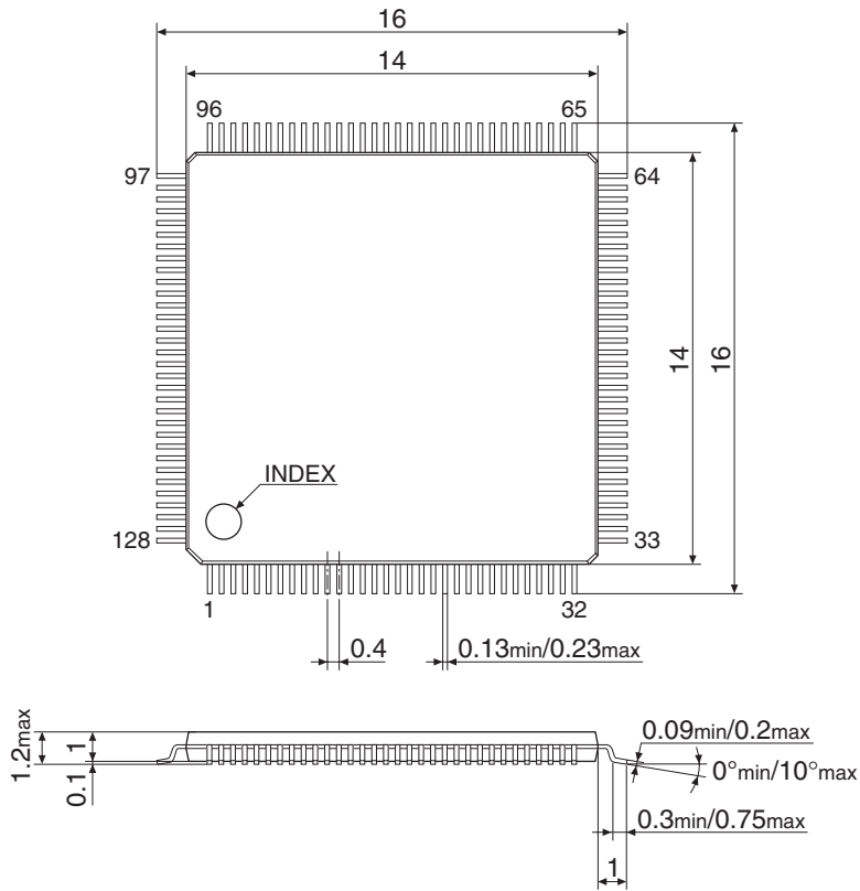
図24.2 TQFP15-128PIN/パッケージ寸法
