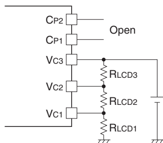
図18.4.2.1 外部印加モード1外部結線例(抵抗分割)
