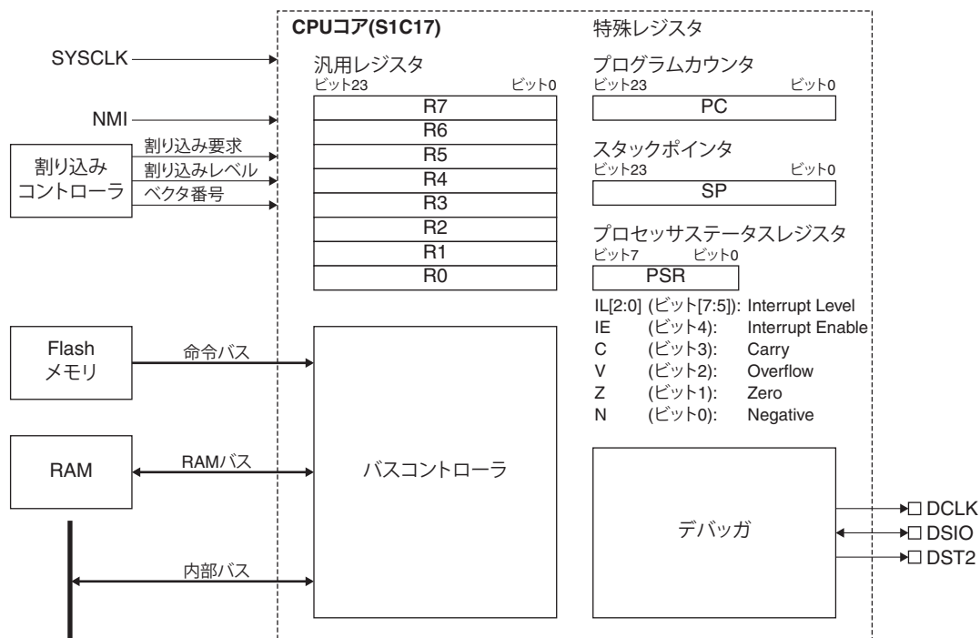
図3.1.1 S1C17の構成
