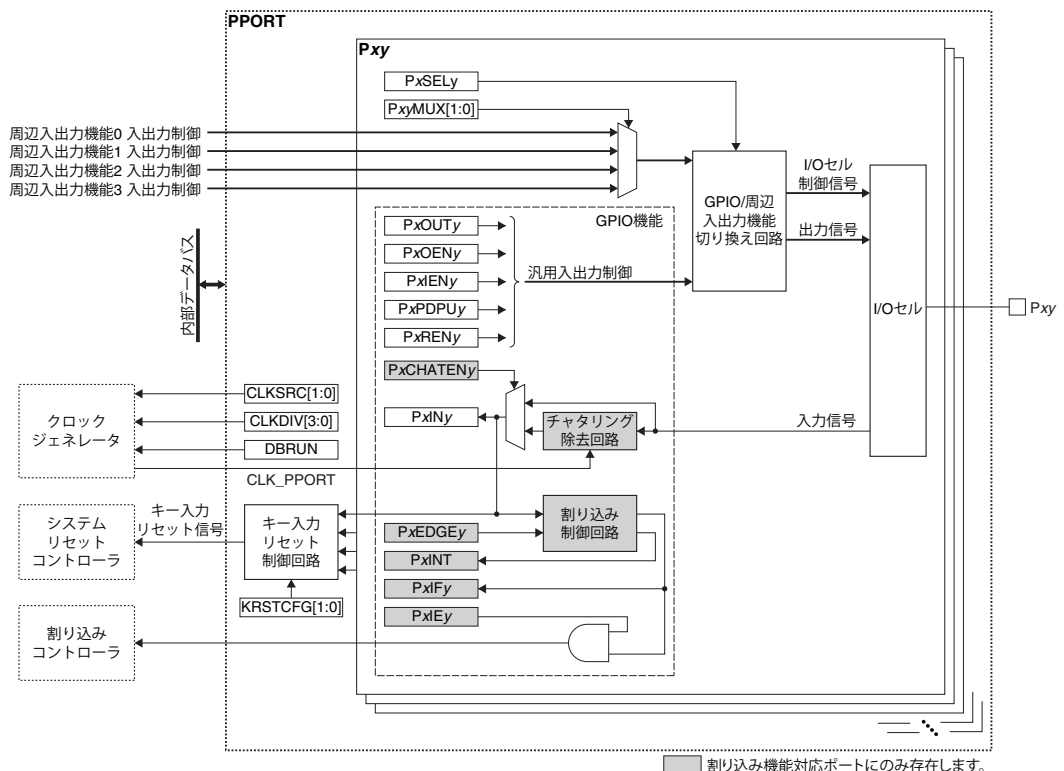
図6.1.1 PPORTの構成
