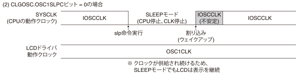
図2.3.4.3 SLEEPモード時のクロック制御例
