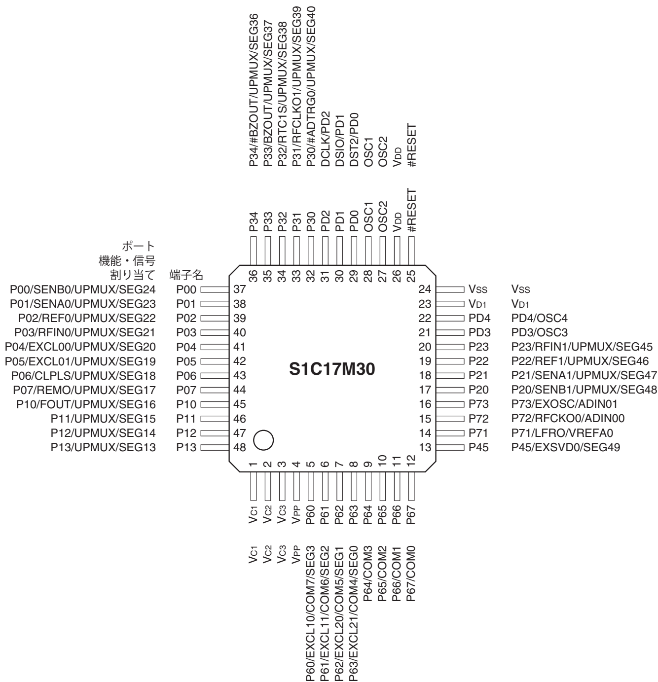
S1C17M30 端子配置図 (TQFP12-48PIN)
