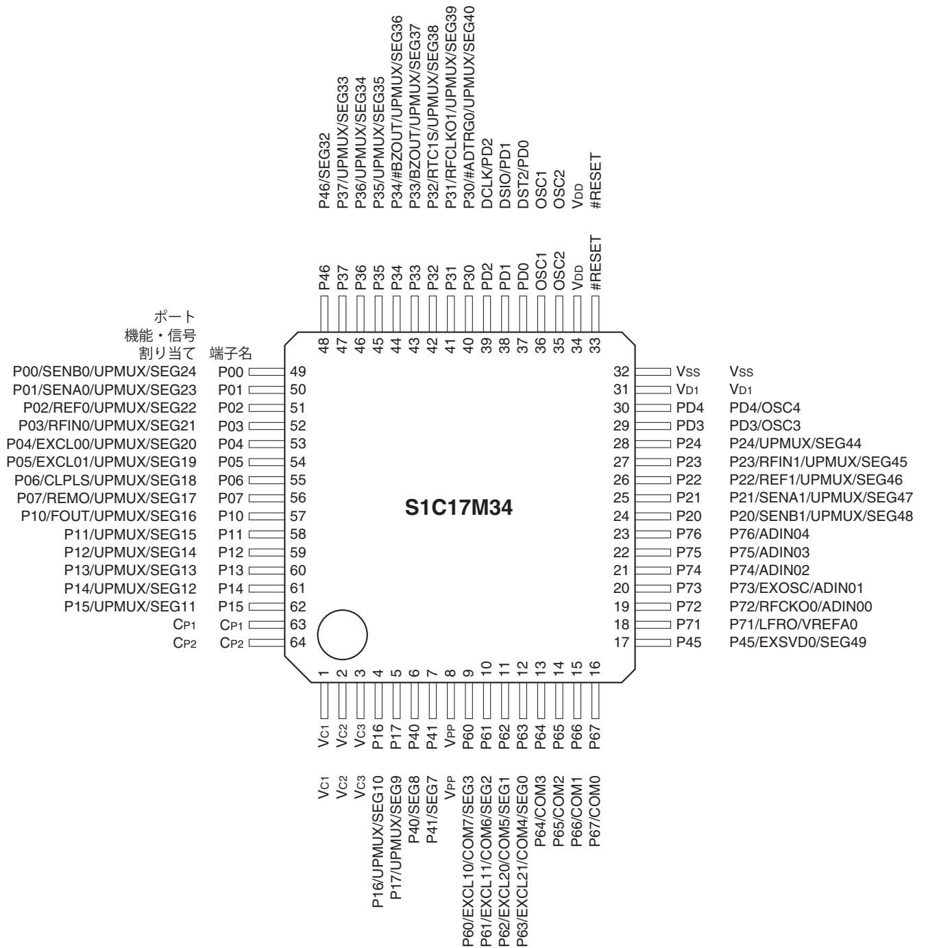
S1C17M34 端子配置図 (TQFP13-64PIN)
