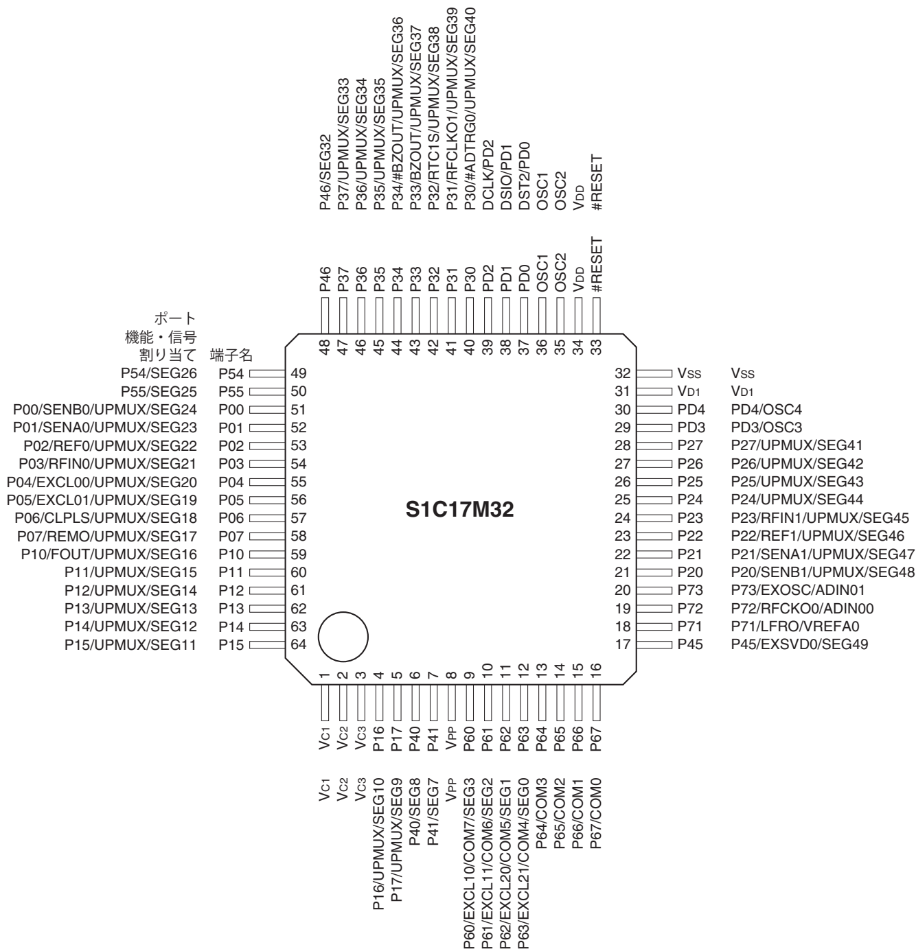
S1C17M32 端子配置図 (TQFP13-64PIN)
