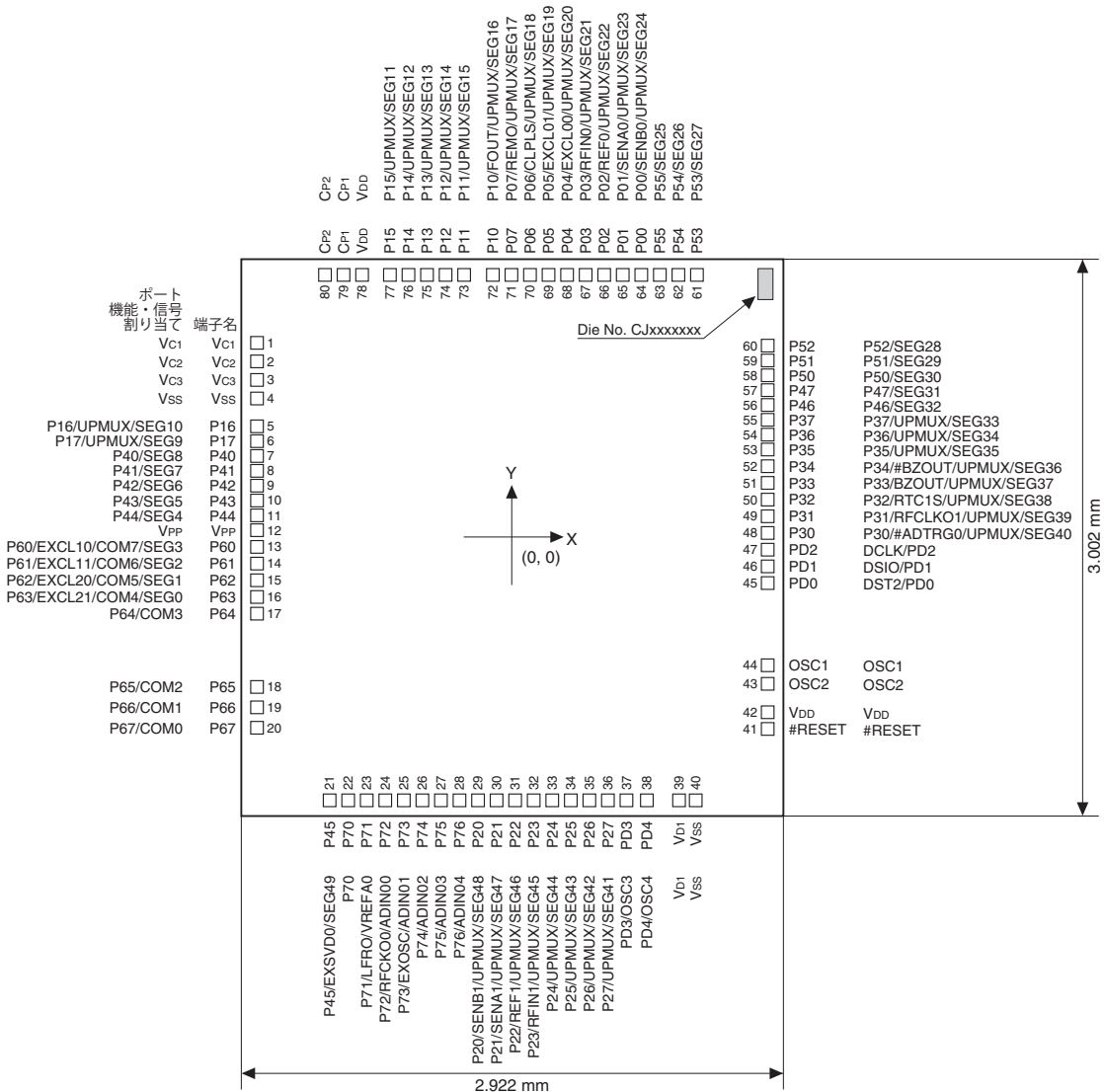
図1.3.5.1 S1C17M33パッド配置図(チップ)
