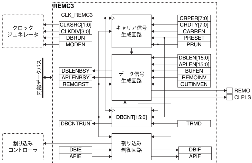
図17.1.1 REMC3の構成
