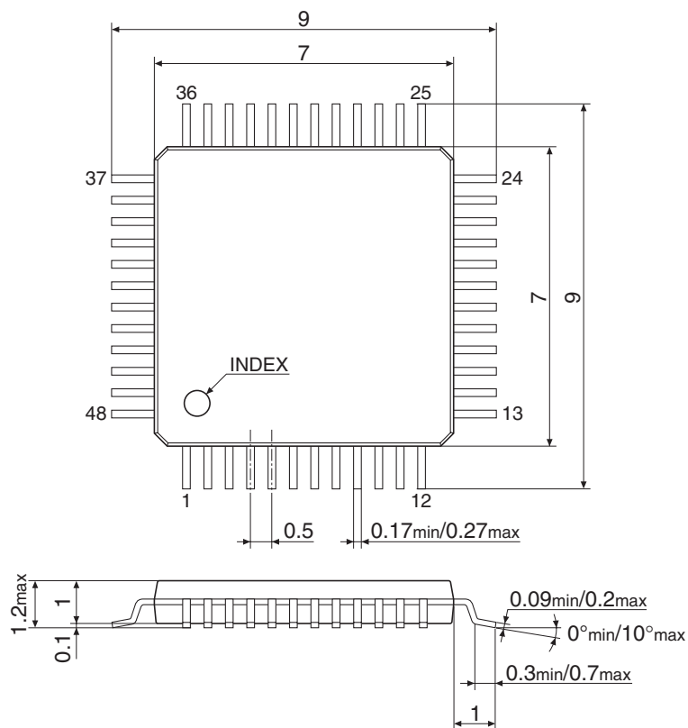
図25.1 TQFP12-48PIN/パッケージ寸法
