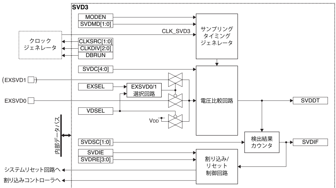
図10.1.1 SVD3の構成
