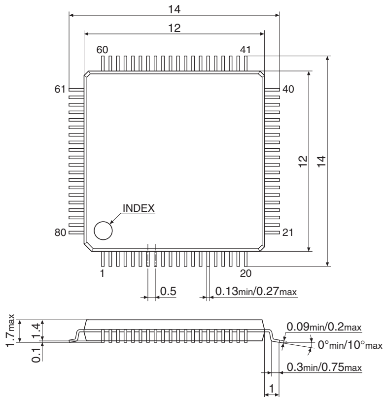
図25.3 QFP14-80PIN/パッケージ寸法
