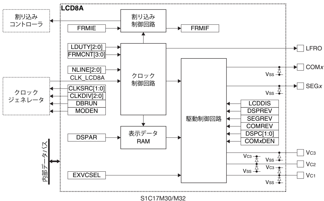
図18.1.1 LCD8Aの構成
