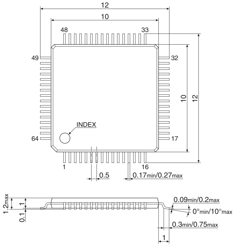
図25.2 TQFP13-64PIN/パッケージ寸法
