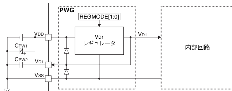
図2.1.1.1 PWGの構成
