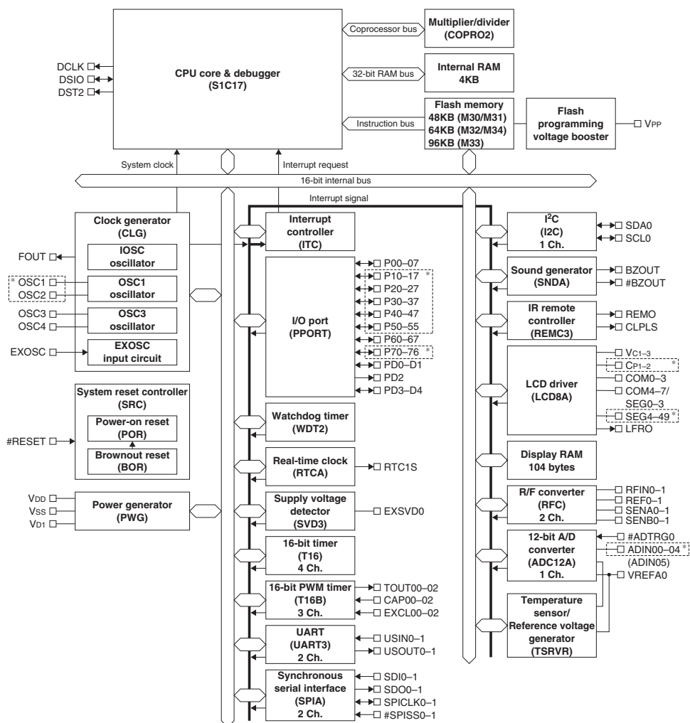
図1.2.1 S1C17M30/M31/M32/M33/M34ブロック図
