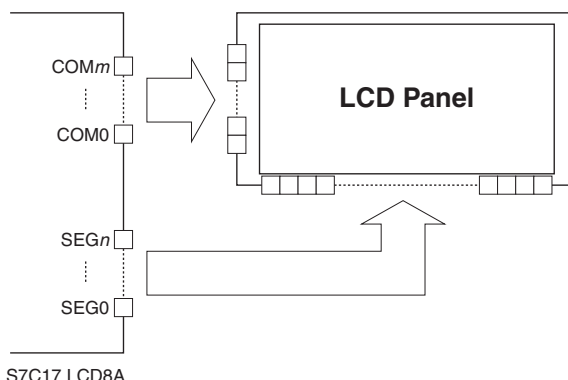
図18.2.2.1 LCD8AとLCDパネルの接続例
