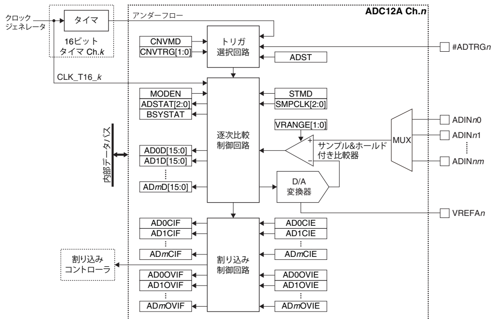
図20.1.1 ADC12Aの構成
