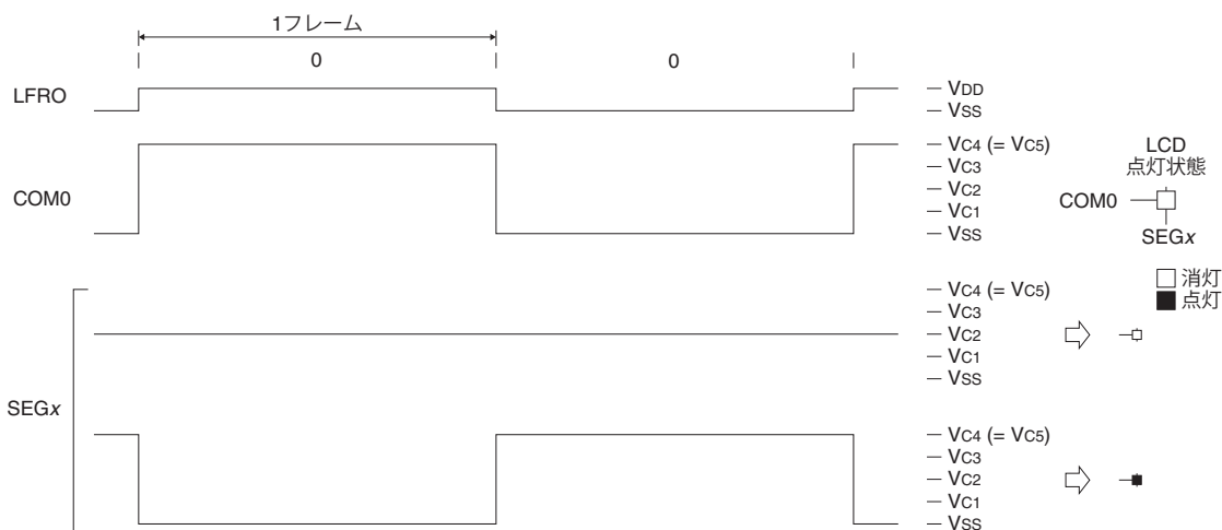
図18.5.5.8 スタティック駆動波形(1/4バイアス)
