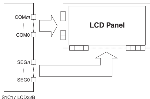
図18.2.2.1 LCD32BとLCDパネルの接続例
