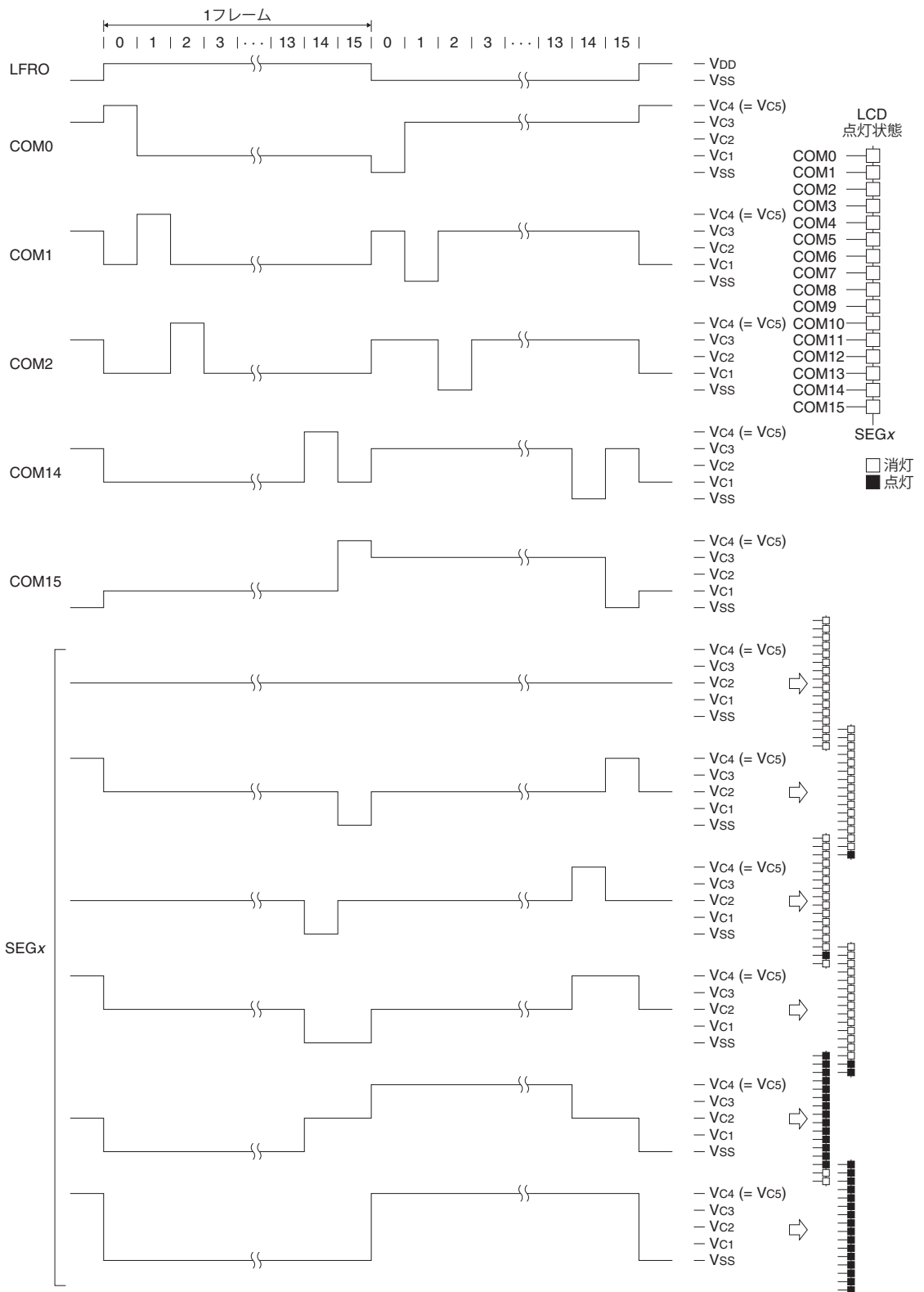
図18.5.5.4 1/16デューティの駆動波形(1/4バイアス)
