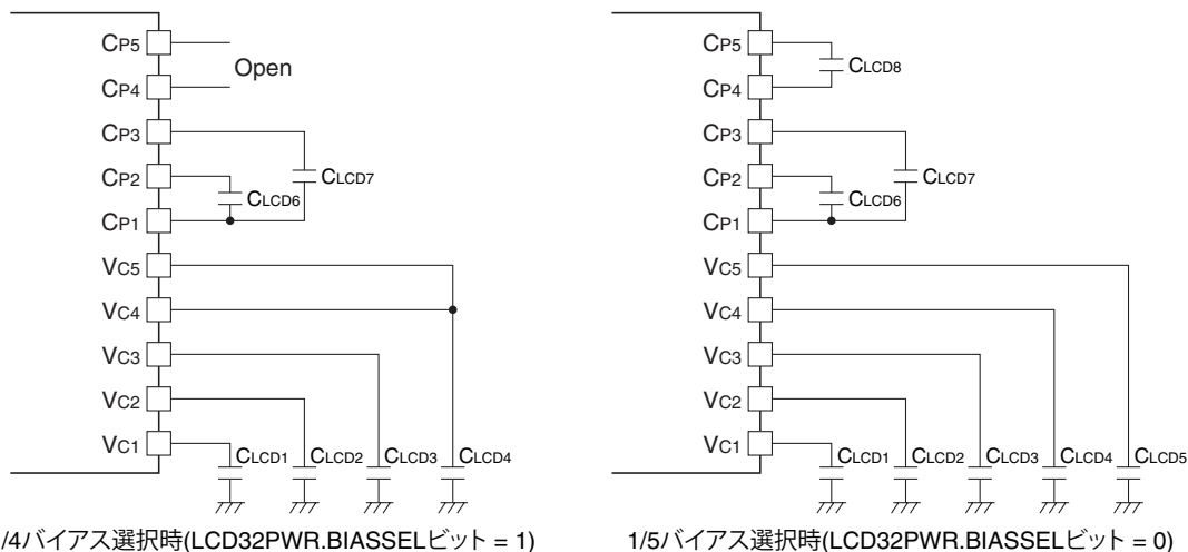
図18.4.1.1 内部生成モード外部結線例
