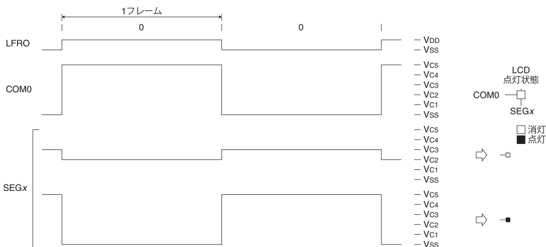
図18.5.5.7 スタティック駆動波形(1/5バイアス)
