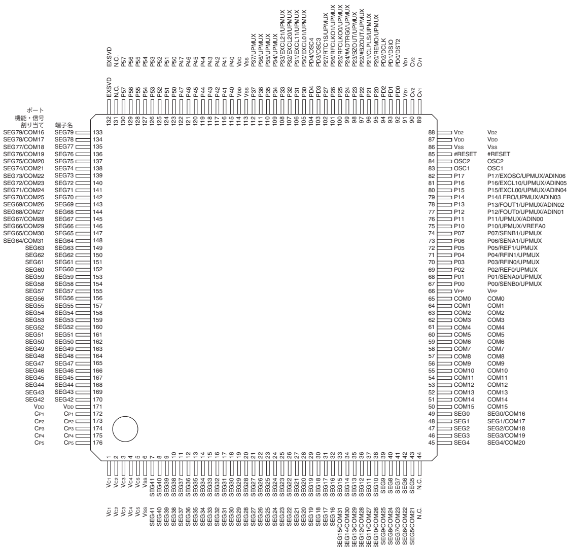
図1.3.1.1 S1C17W34/W35/W36端子配置図(QFP21-176PIN)
