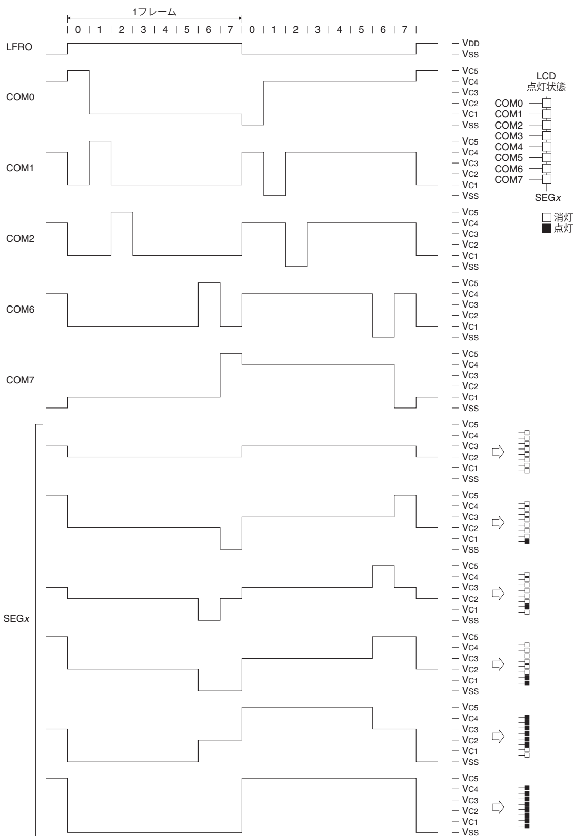
図18.5.5.5 1/8デューティの駆動波形(1/5バイアス)
