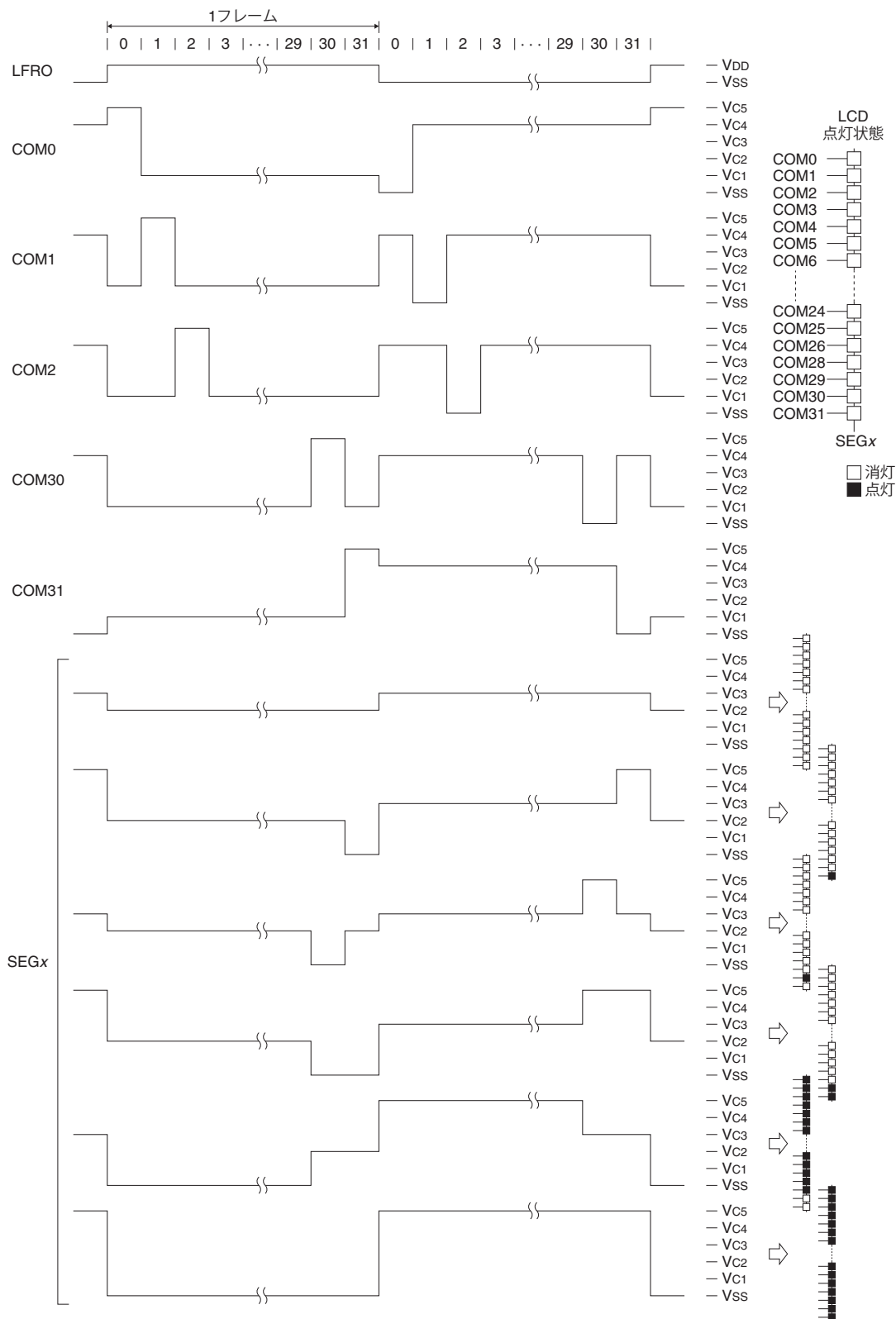
図18.5.5.1 1/32デューティの駆動波形(1/5/バイアス)
