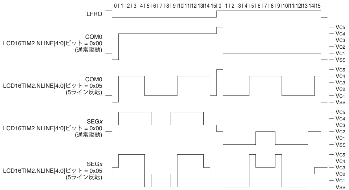
図18.5.7.1 1/16デューティ (1/5バイアス)の通常駆動時と5ライン反転時の駆動波形
