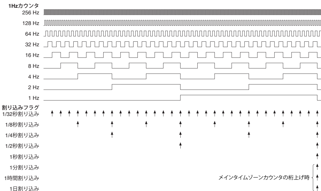
図9.5.1 RTCA2割り込みタイミング
