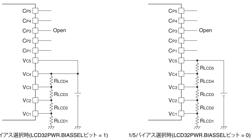
図18.4.2.1 外部印加モード外部結線例(抵抗分割)
