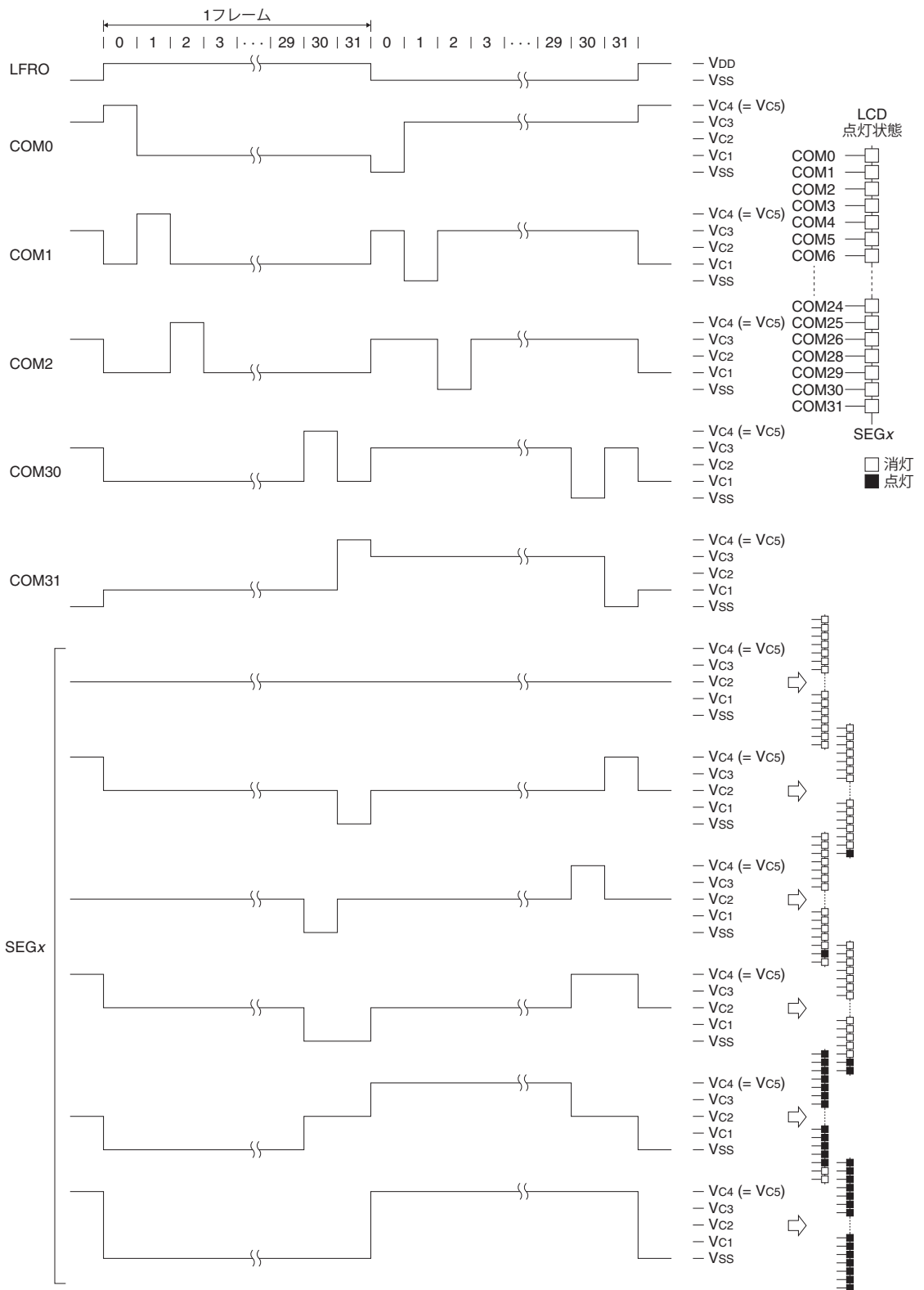
図18.5.5.2 1/32デューティの駆動波形(1/4バイアス)
