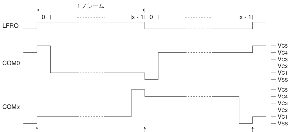
図18.7.1 フレーム割り込みタイミング(1/xデューティ、1/5バイアス)
