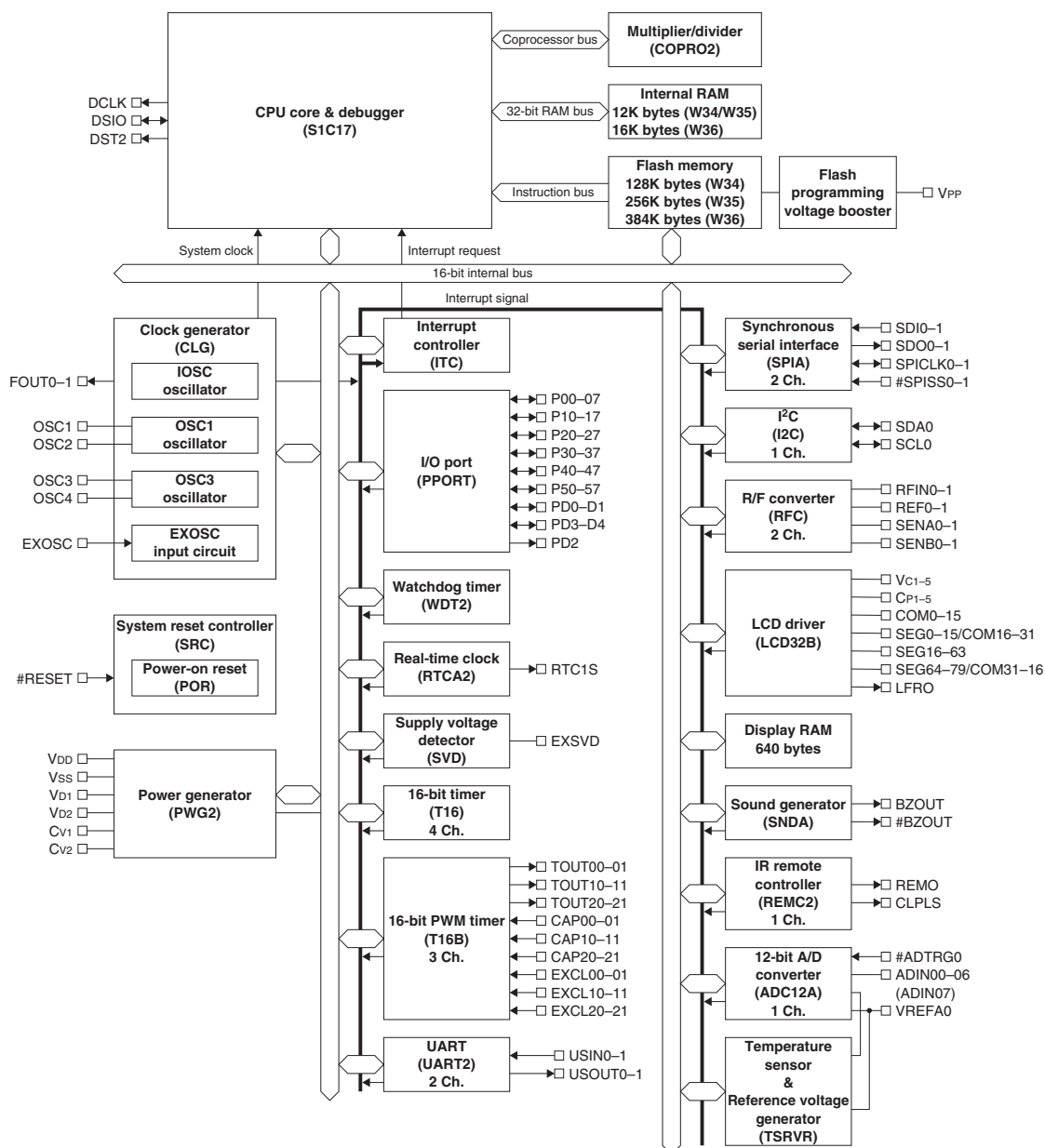
図1.2.1 S1C17W34/W35/W36ブロック図
