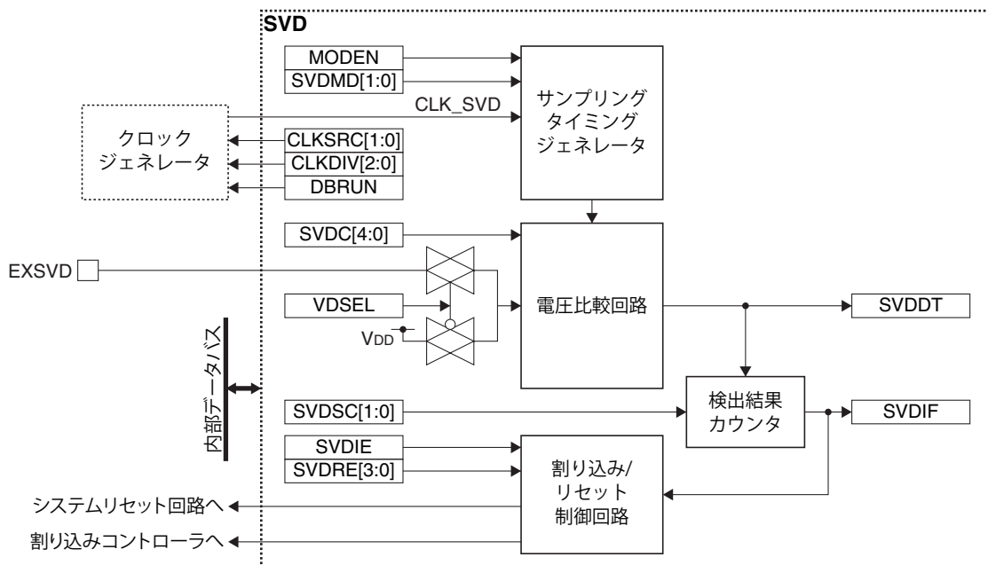
図10.1.1 SVDの構成
