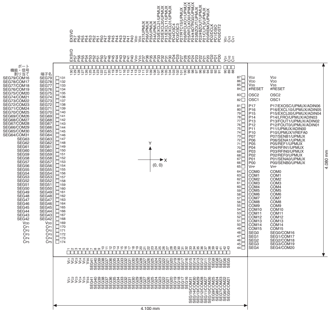
図1.3.2.1 S1C17W34/W35/W36/パッド配置図(チップ)
