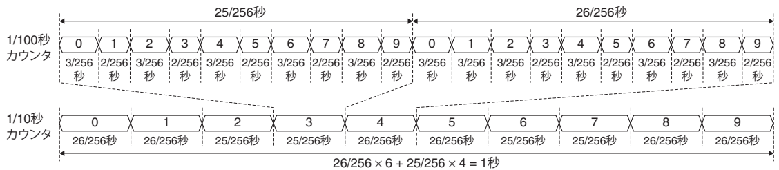
図9.4.4.1 ストップウォッチのカウンタアップパターン
