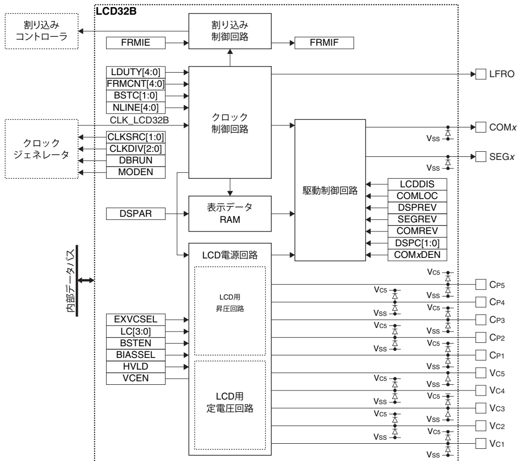
図18.1.1 LCD32Bの構成
