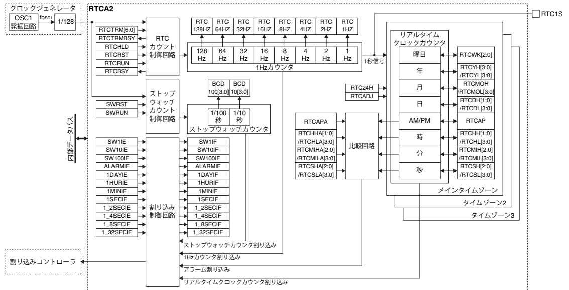
図9.1.1 RTCA2の構成
