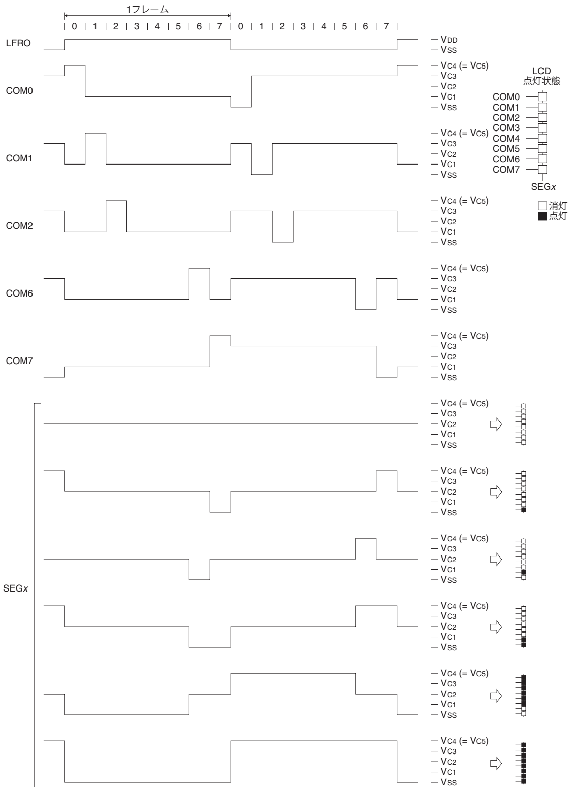
図18.5.5.6 1/8デューティの駆動波形(1/4バイアス)
