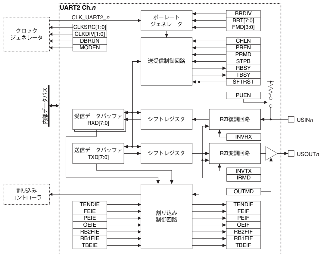
図12.1.1 UART2の構成
