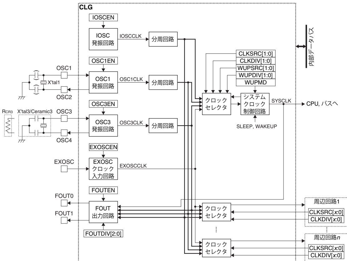
図2.3.1.1 CLGの構成
