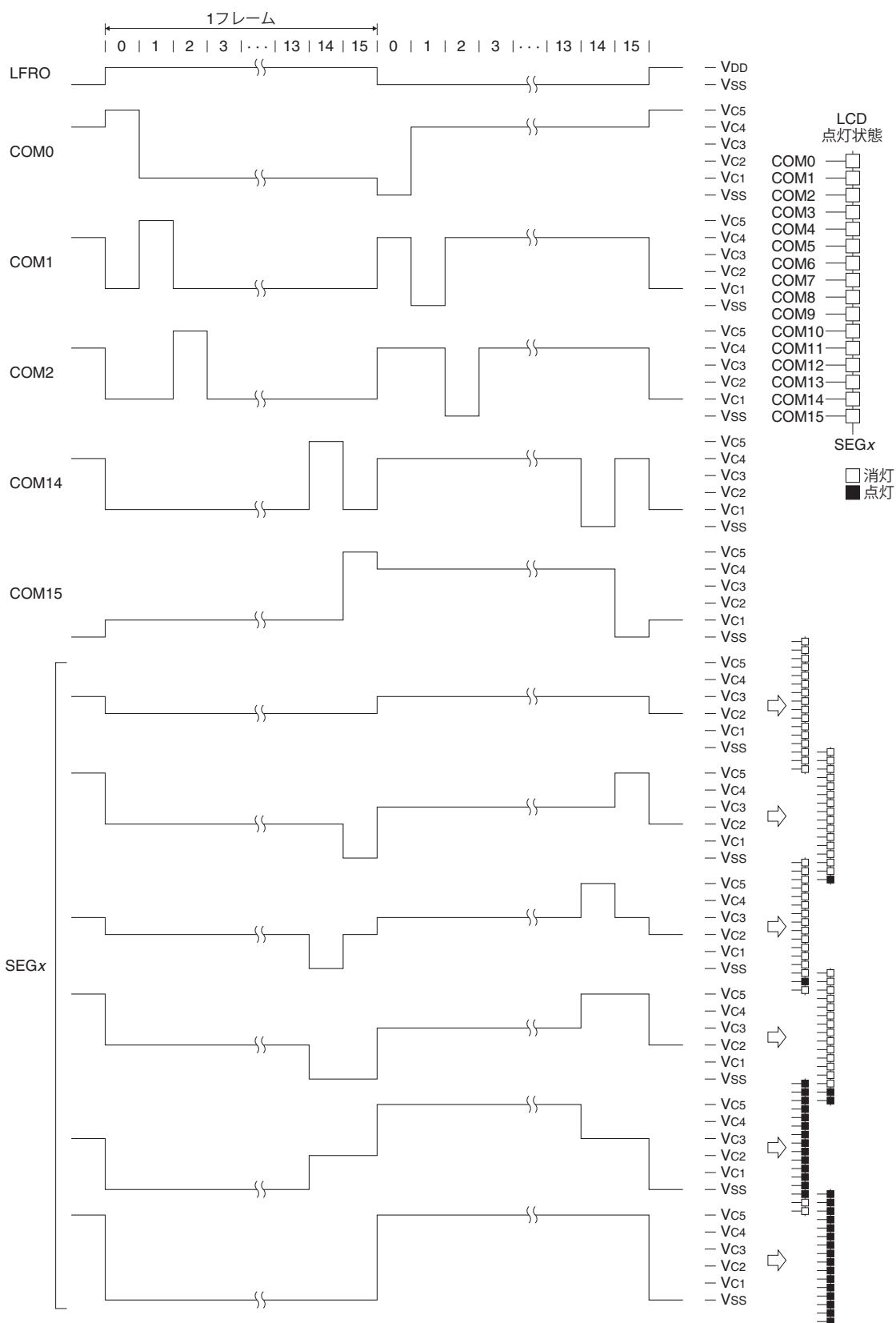
図18.5.5.3 1/16デューティの駆動波形(1/5バイアス)
